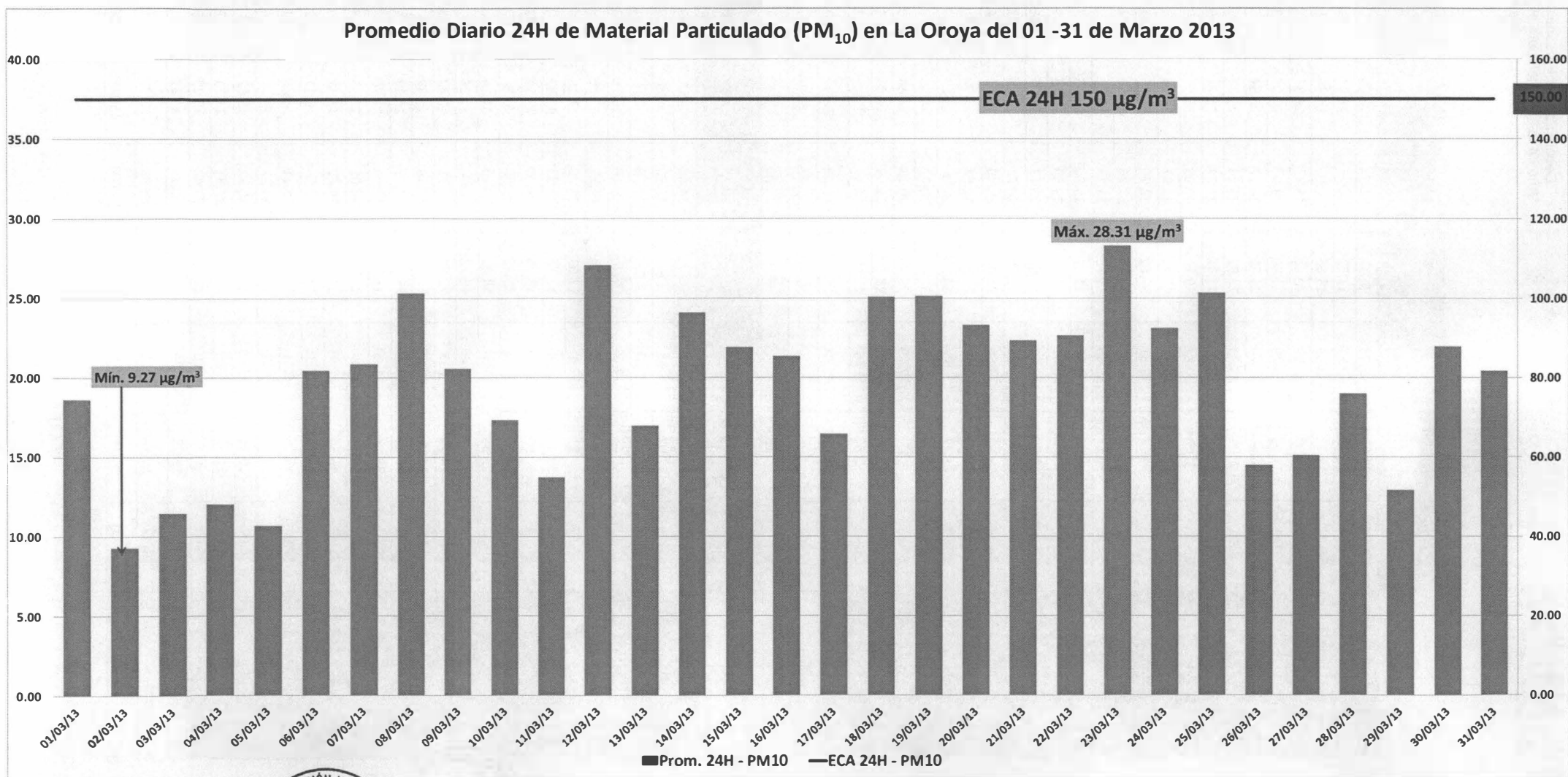
Gráfica N° 07. Promedio Diario de PM 10 – Vista Mensual
