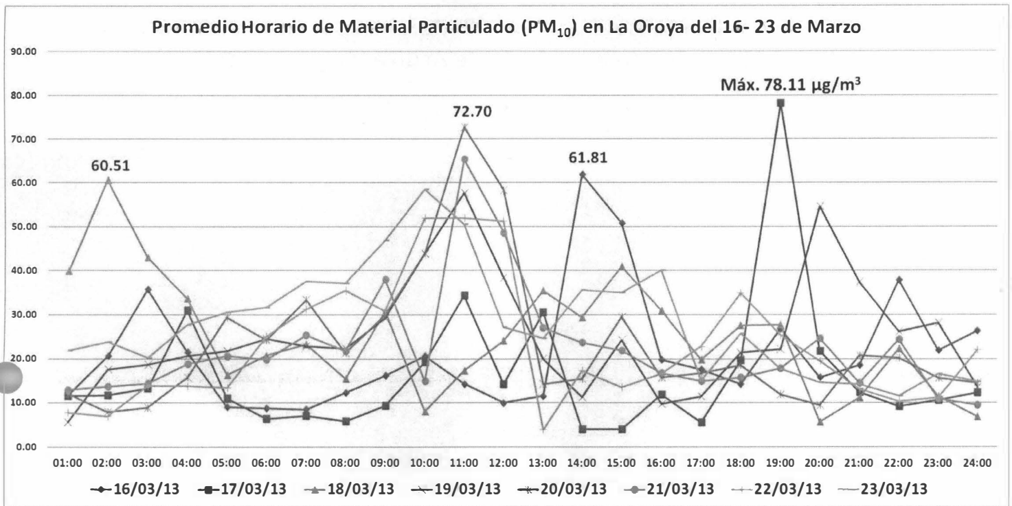
Gráfica N° 11. Promedio Horario de PM 10 – Vista Semanal
