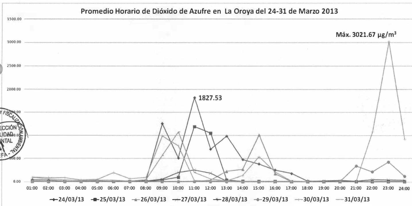
Gráfica N° 06. Promedio Horario de SO 2 – Vista Semanal
