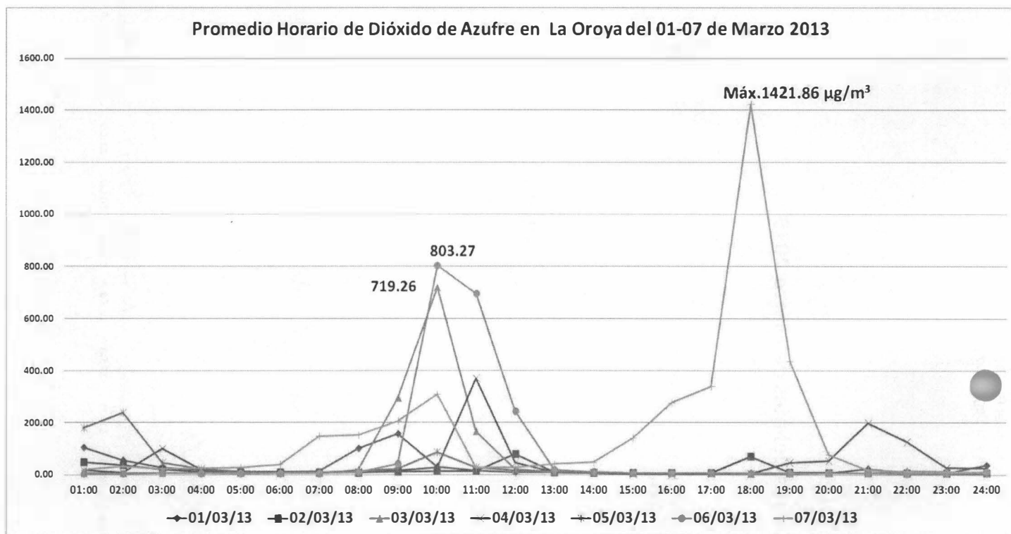
Gráfica N° 03. Promedio Horario de SO 2 – Vista Semanal
