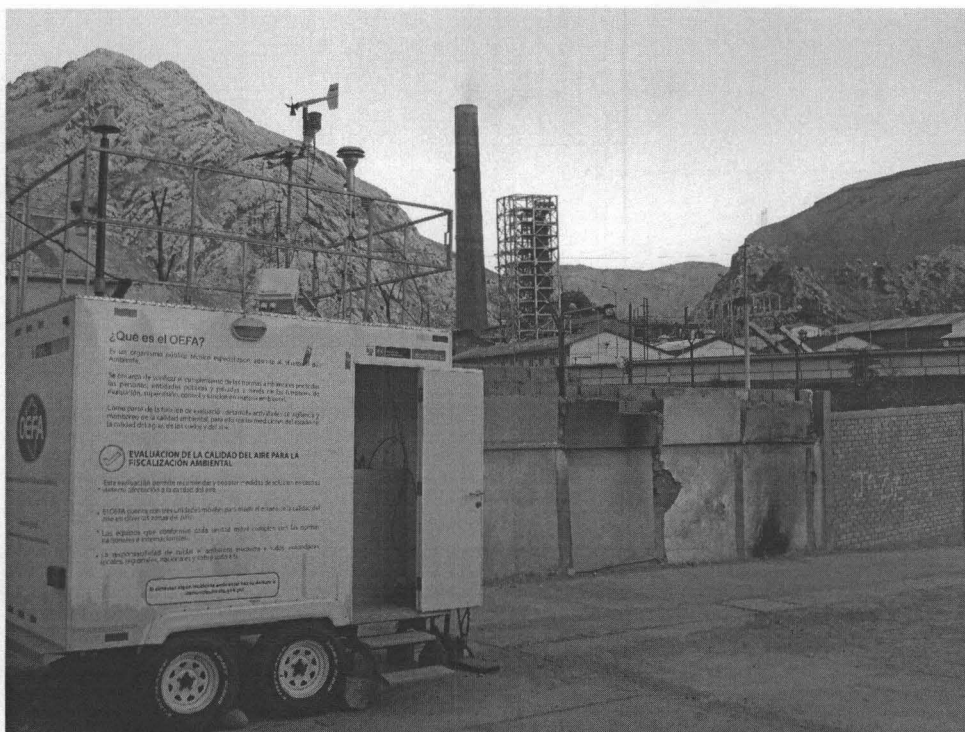
Fotografía N° 01.- Unidad Móvil de Calidad del Aire – Estación Meteorológica (Costado Mercado Nuevo La Oroya Antigua).
