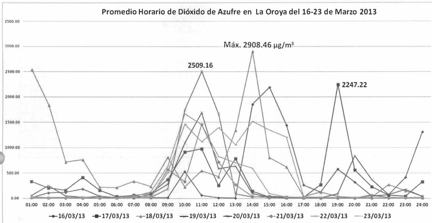
Gráfica N° 05. Promedio Horario de SO 2 – Vista Semanal
