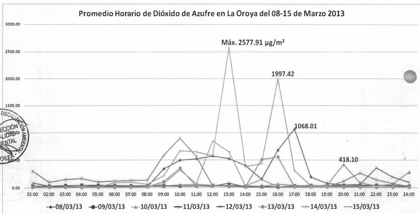
Gráfica N° 04. Promedio Horario de SO 2 – Vista Semanal
