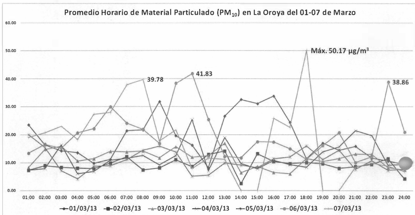
Gráfica N° 09. Promedio Horario de PM 10 – Vista Semanal
