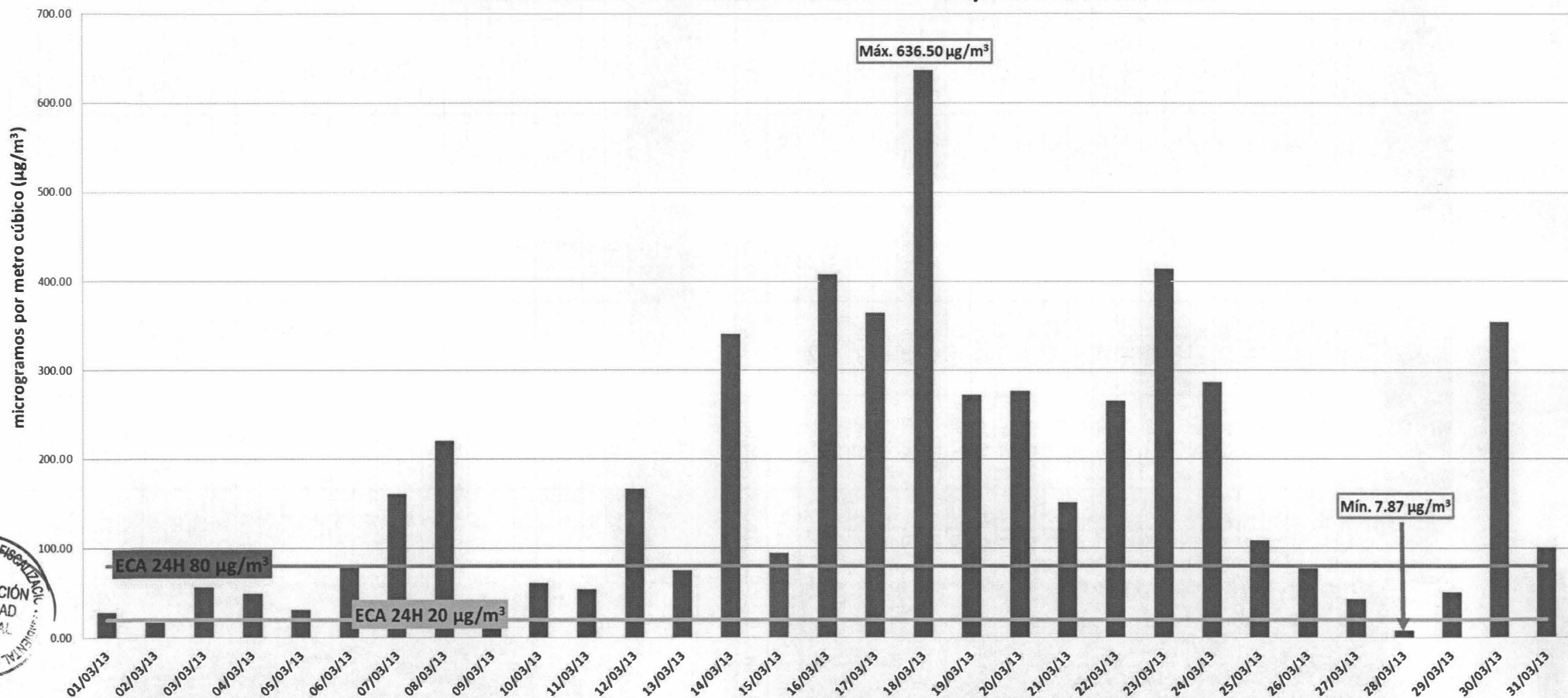
Promedio Diario 24H de Dióxido de Azufre en La Oroya del mes de marzo 2013
