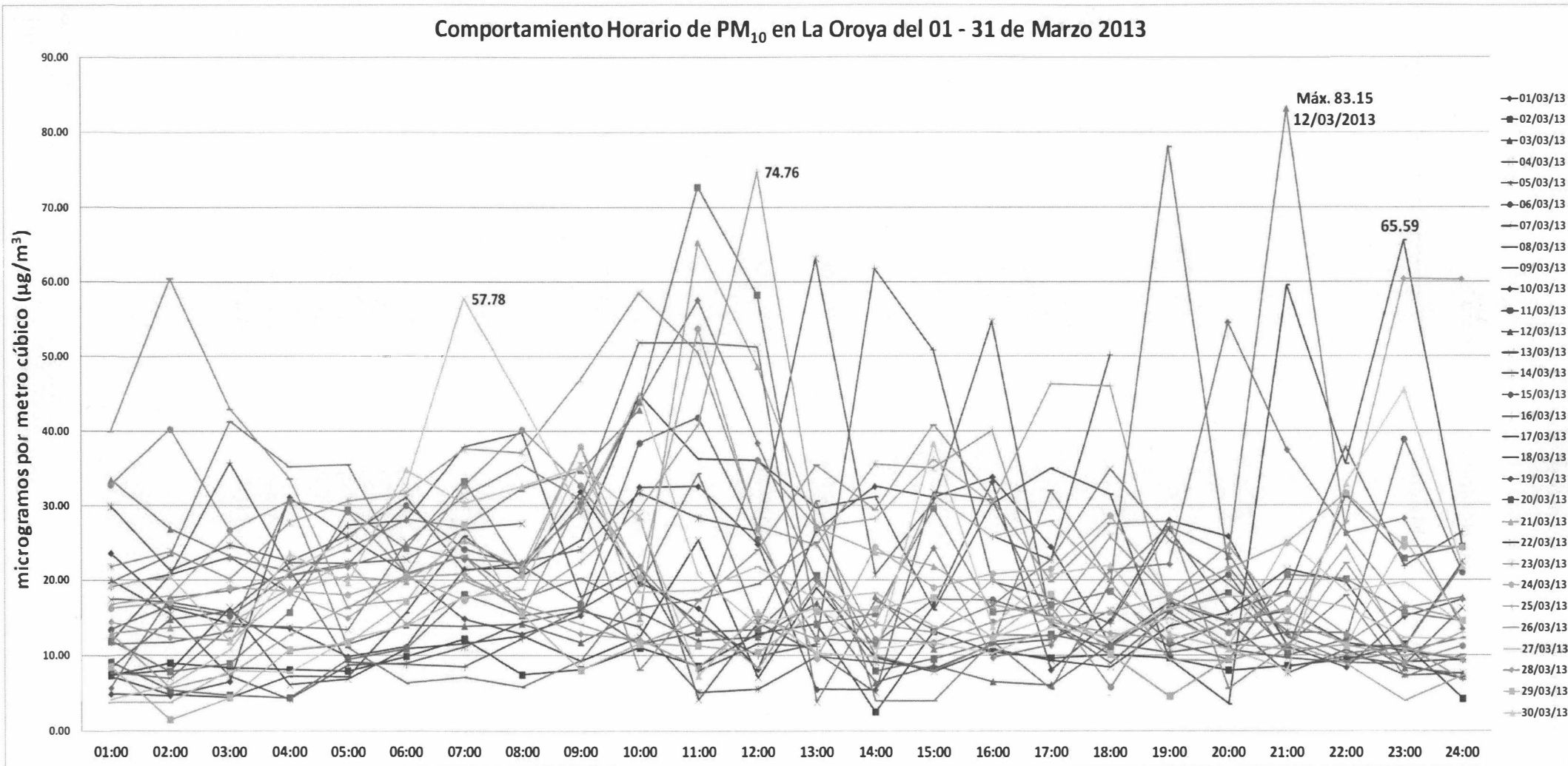
Gráfica N° 08. Promedio Horario de PM 10 – Vista Mensual.
