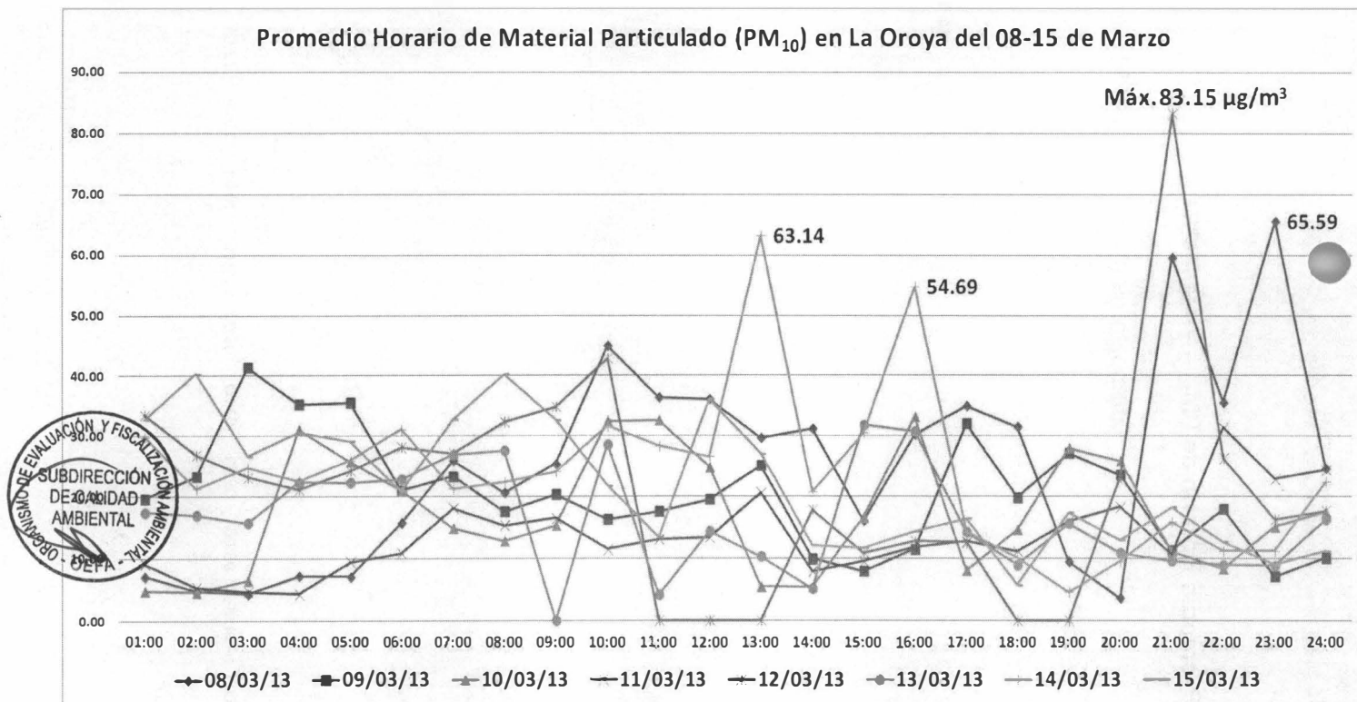
Gráfica N° 10. Promedio Horario de PM 10 – Vista Semanal
