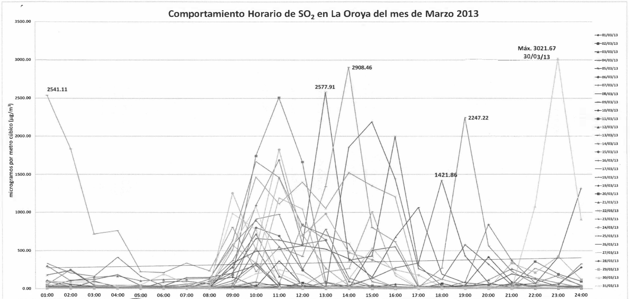
Gráfica N° 02. Promedio Horario de SO 2 – Vista Mensual
