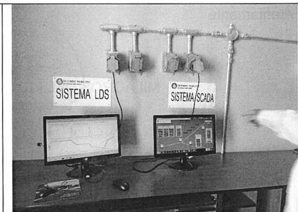
Fotografía 6. Equipos de monitoreo Sistema Scada localizados en la estación Paita, mediante el cual se cierra ducto en caso de emergencia
