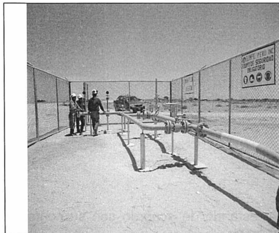
Fotografía 3 Manifold
