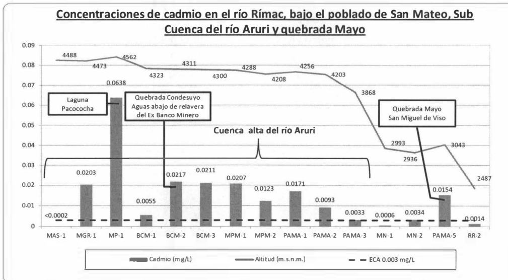
Gráfica N° 07: Concentraciones de cadmio en el río Rímac bajo el poblado de San Mateo, Sub Cuenca del río Aruri y quebrada Mayo
