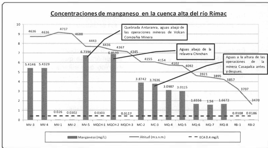
Gráfica N° 04: Concentraciones de manganeso en la cuenca alta
