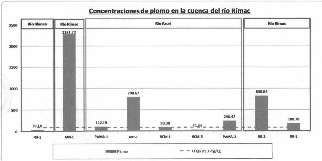
Gráfica N° 14: Concentración de Plomo en sedimento de la cuenca del río Rímac
