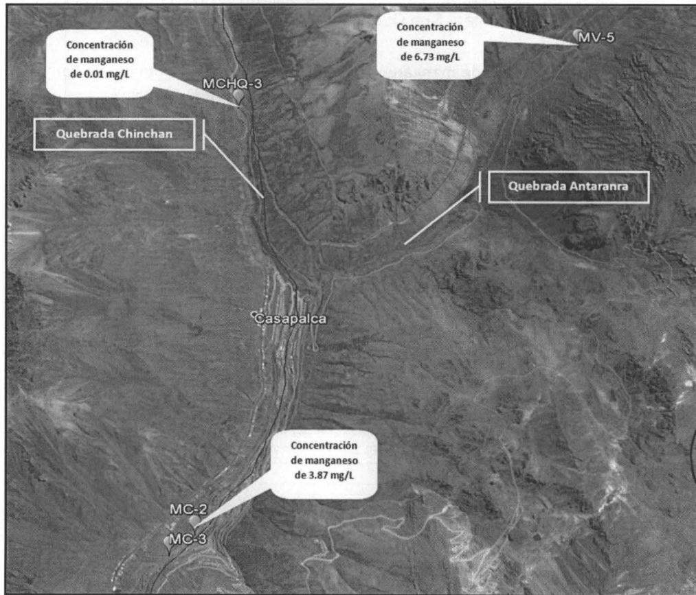
Gráfica N° 03: Concentraciones de manganeso en la cabecera del Rimac
