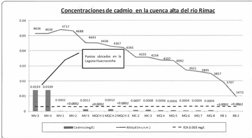
Gráfica N° 06: Concentraciones de cadmio en la cuenca alta del río Rímac
