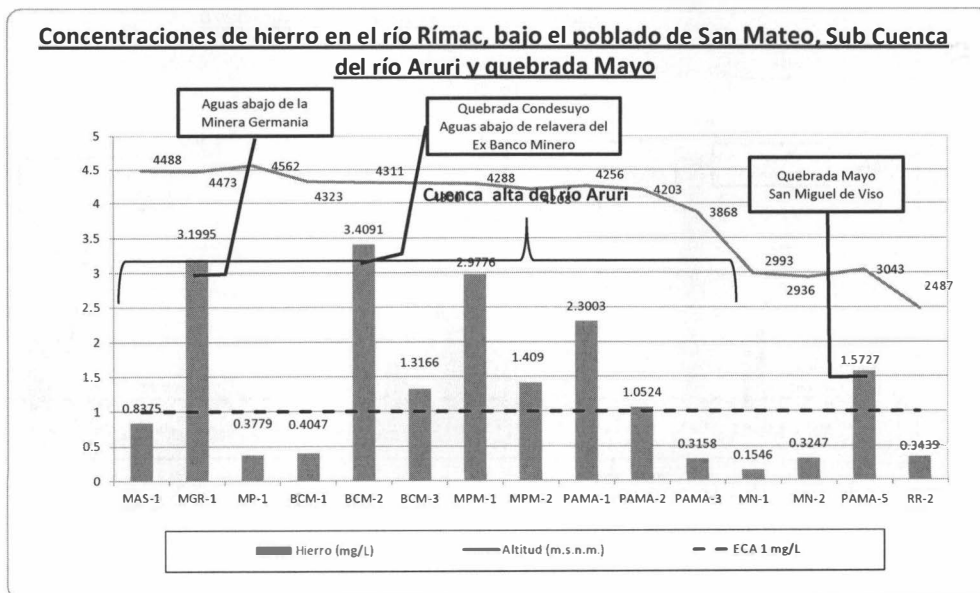
Gráfica N° 09: Concentraciones de hierro en el río Rímac bajo el poblado de San Mateo, Sub Cuenca del río Aruri y quebrada Mayo
