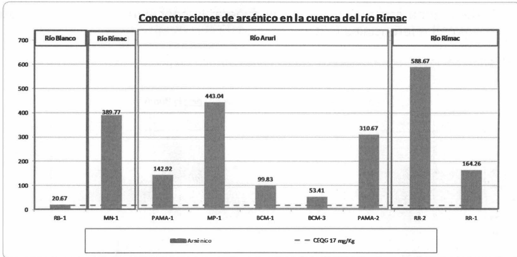
Gráfica N° 13: Concentración de arsénico en sedimento de la cuenca del río Rímac
