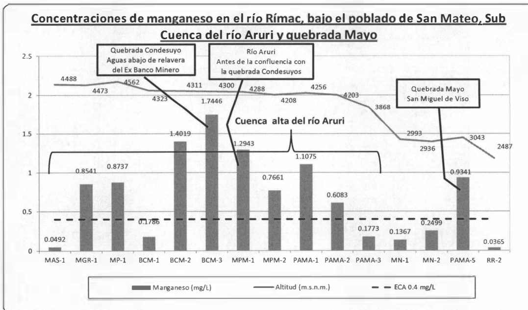
Gráfica N° 05: Concentraciones de manganeso en el río Rímac bajo el poblado de San Mateo, Sub Cuenca del río Aruri y quebrada Mayo
