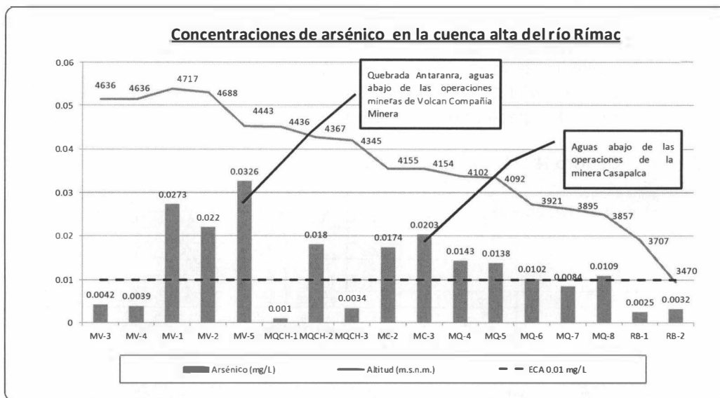
Gráfica N° 01: Concentraciones de arsénico en la cuenca alta del Rímac
