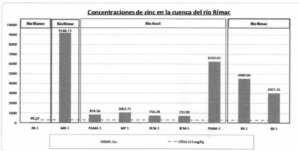
Gráfica N° 12: Concentración de zinc en sedimento en la cuenca del río Rímac
