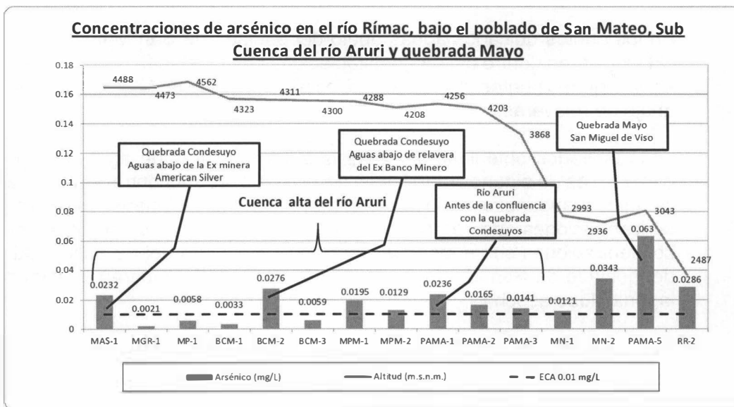
Gráfica N° 02: Concentraciones de arsénico en el río Rímac bajo el poblado de San Mateo, Sub Cuenca del río Aruri y quebrada Mayo
