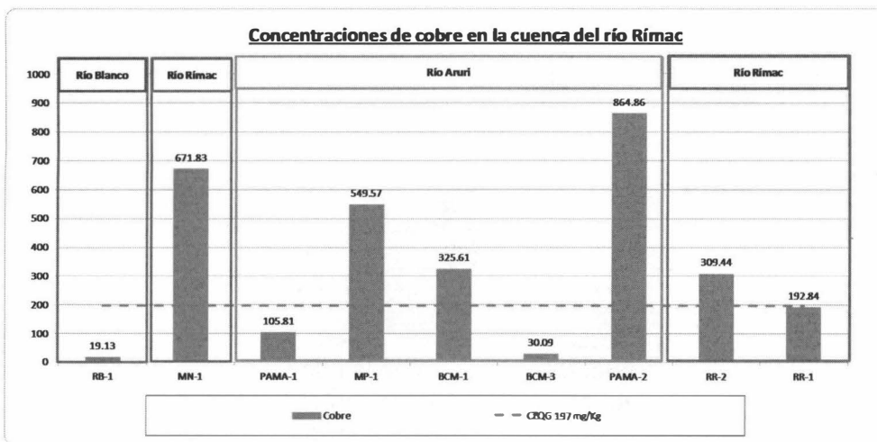
Gráfica N° 11: Concentración de cobre en sedimento en la cuenca del río Rímac
