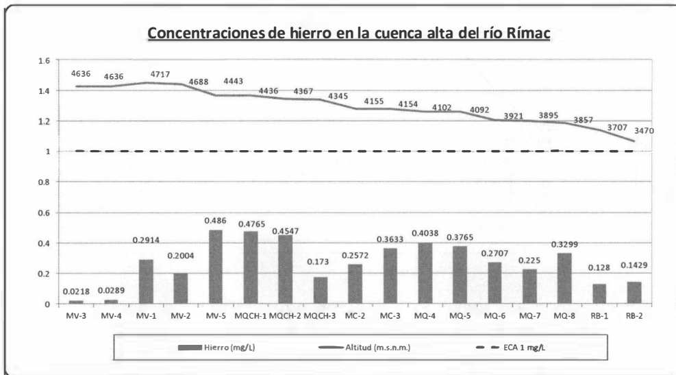
Gráfica N° 08: Concentraciones de hierro en la cuenca alta del río Rímac
