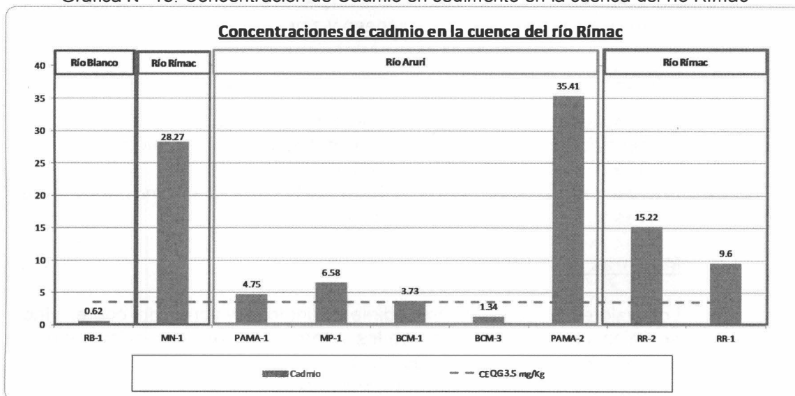
Gráfica N° 15: Concentración de Cadmio en sedimento en la cuenca del río Rímac
