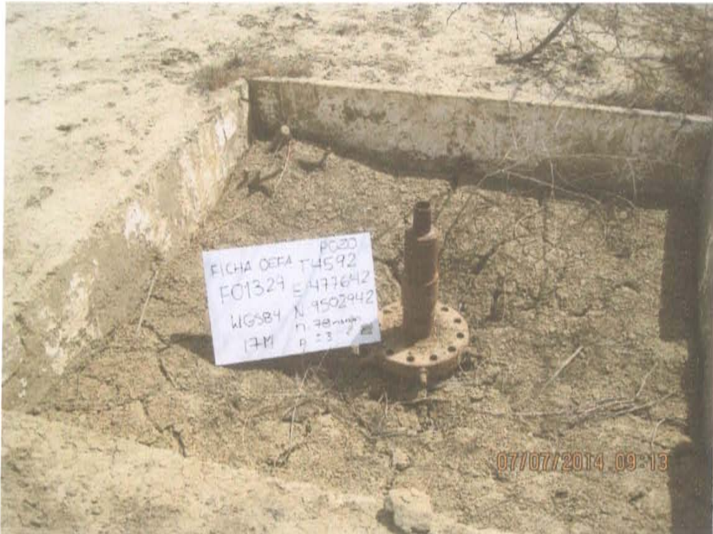
Fotografía N° 1. Se observa casing corroído con brida que sobresale aproximadamente 0,69 m desde el fondo de una cantina de concreto.
