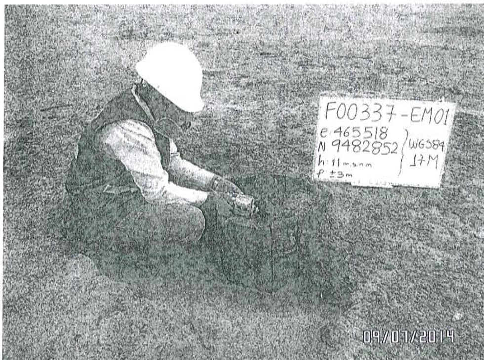
Fotografía N° 1. Medición en el punto F00337-EM01, ubicado en la fuente de emisión en boca del Pozo T_530.
