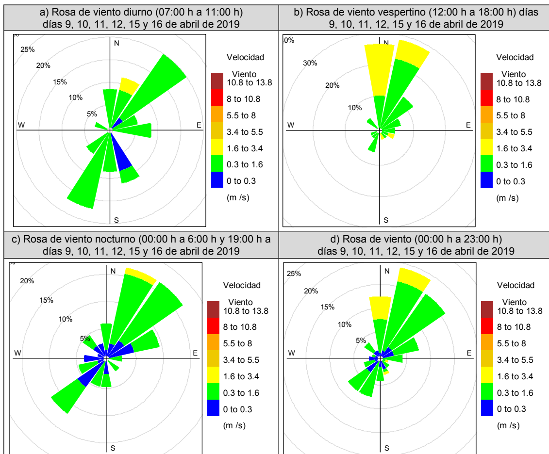
Figura 5.1. Rosa de viento en el distrito de Simón Bolívar los días 9, 10, 11, 12, 15 y 16 de abril de 2019 a) en horario diurno, b) en horario vespertino, c) en horario nocturno, d) en todas las horas.
