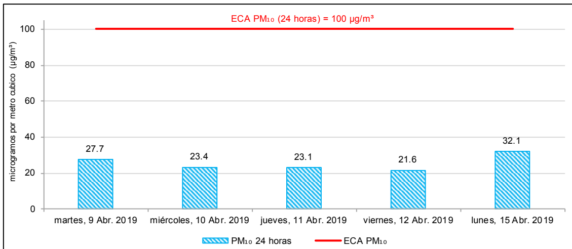
Figura 5.3. Concentraciones de 24 horas de PM 10 en la estación de vigilancia ambiental CA-SB-02, del 9, 10, 11, 12 y 15 de abril de 2019.
