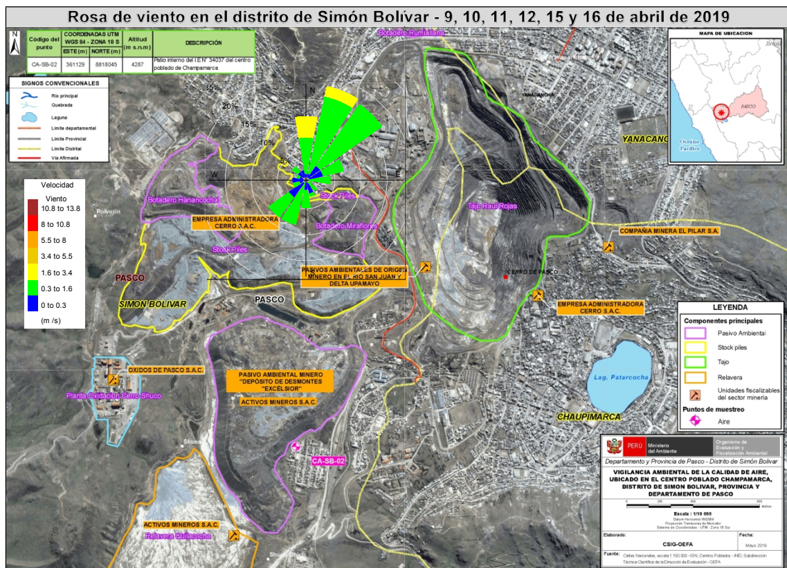
Figura 5.2. Ubicación de la estación meteorológica en el distrito de Simón Bolívar y rosa de Vientos los días 9, 10, 11, 12, 15 y 16 de abril de 2019, respecto a la ubicación de la estación CA-SB-02. Referencia: Imágenes satelital extraídas de Google Earth.
