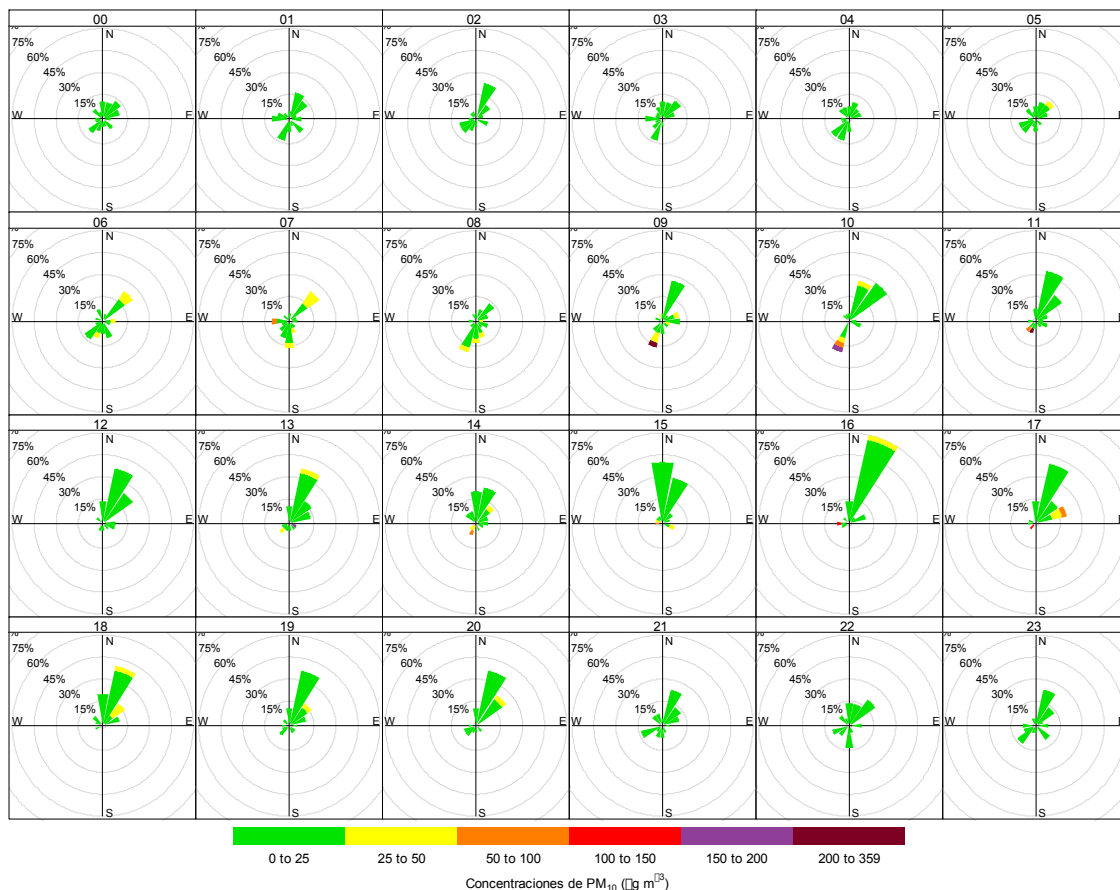
Figura 5.5. Rosas de concentración por horas de PM 10 en la estación de vigilancia CA-SB-01, desde las 00:00 horas hasta las 23:00 horas, en abril de 2019 Nota: Las paletas indican la dirección de donde proviene las concentraciones de PM 10
