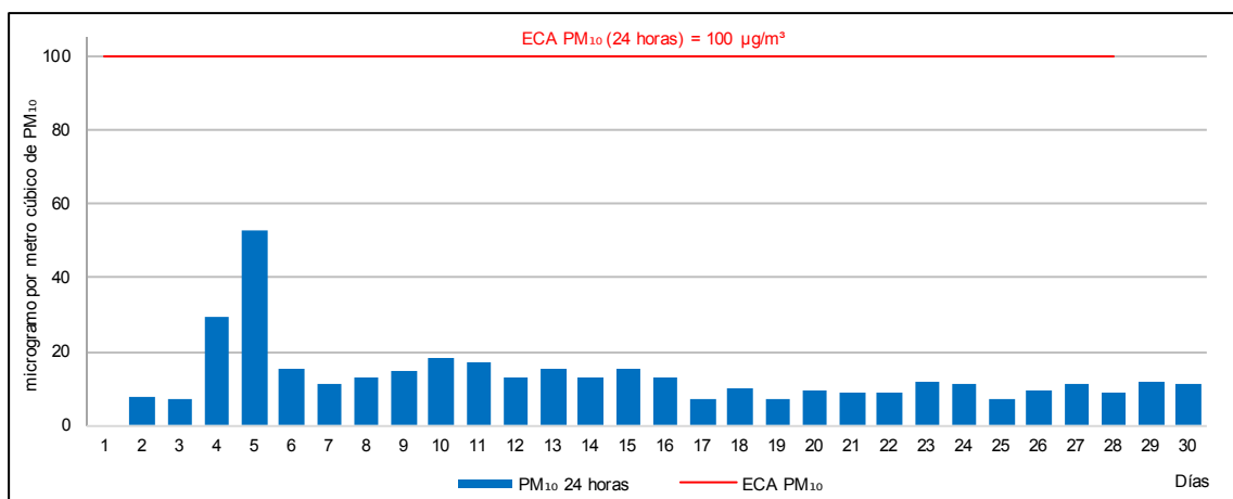
Figura 5.3. Concentraciones de 24 horas de PM 10 en la estación de vigilancia ambiental CA-SB-01, abril de 2019
