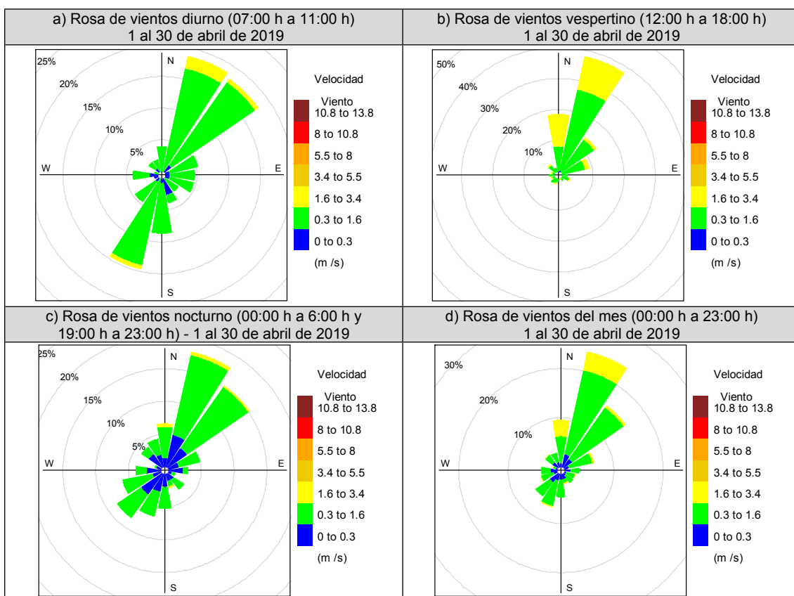
Figura 5.1. Representación gráfica de las rosas de vientos en la estación de vigilancia ambiental CA-SB-01, en abril de 2019 a) en horario diurno, b) en horario vespertino, c) en horario nocturno, d) en todas las horas del mes
