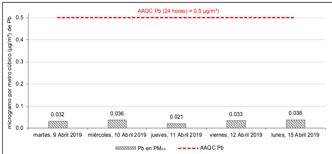
Figura 5.6. Concentraciones de plomo en material particulado con diámetro menor a 10 micras (Pb en PM 10 ) a 10°C y de 24 horas en abril 2019, de la estación de vigilancia ambiental de la calidad del aire CA-SB-01 comparadas de manera referencial con la normativa canadiense AAQC-2012.
