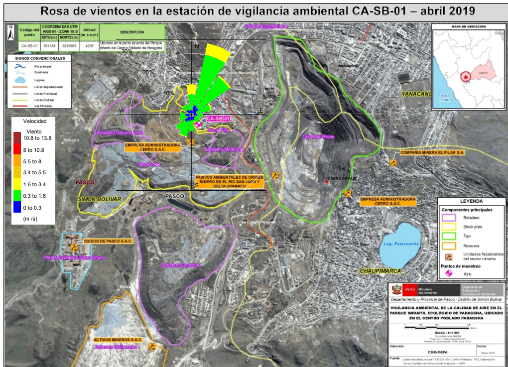
Figura 5.2. Ubicación de la estación de vigilancia ambiental CA-SB-01 y rosa de vientos en abril de 2019
