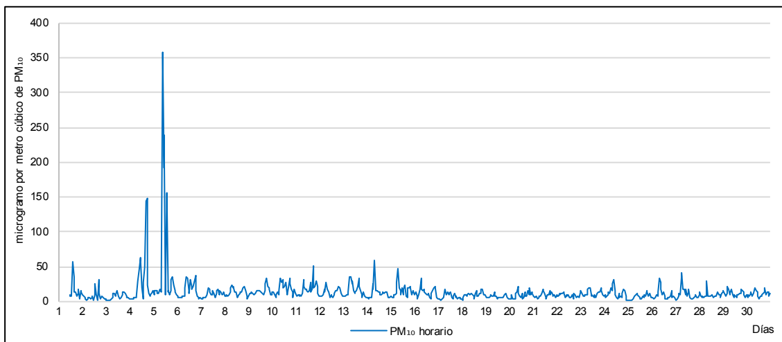
Figura 5.4. Concentraciones horarias de PM 10 en la estación de vigilancia ambiental CA-SB-01 en abril de 2019.
