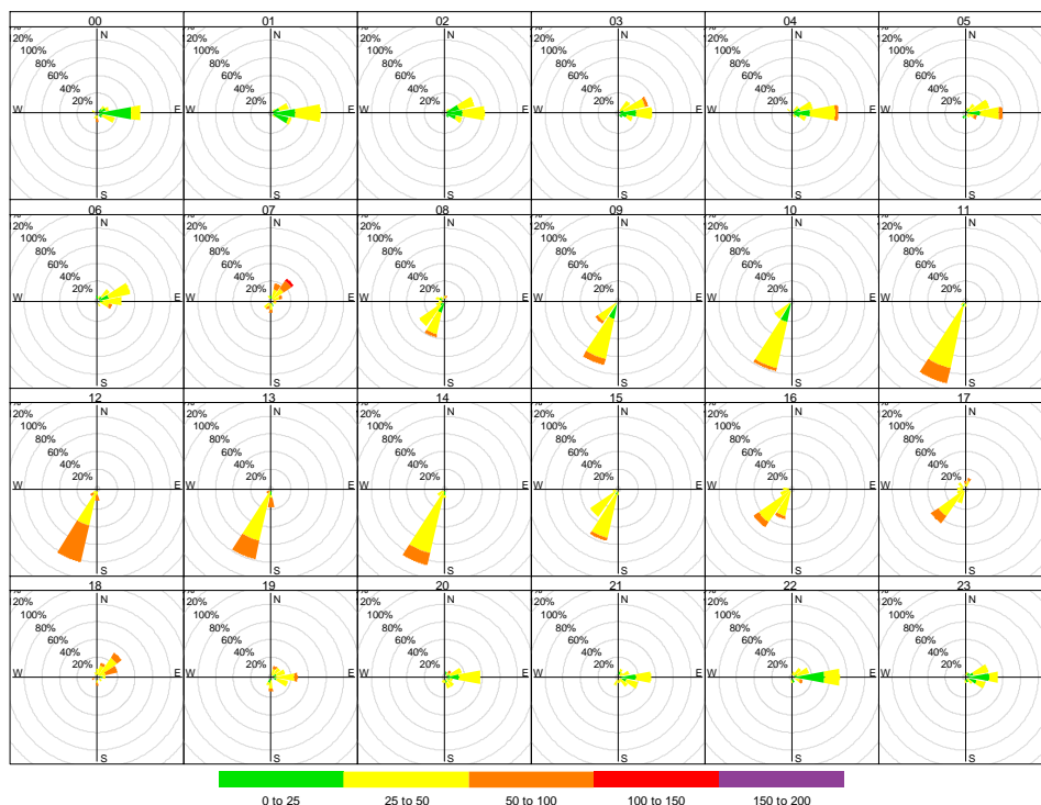
Figura 5.5. Rosas de concentración por horas de PM_{10} en la estación de vigilancia CA-TO-01, desde las 00:00 horas hasta las 23:00 horas, en abril de 2019
