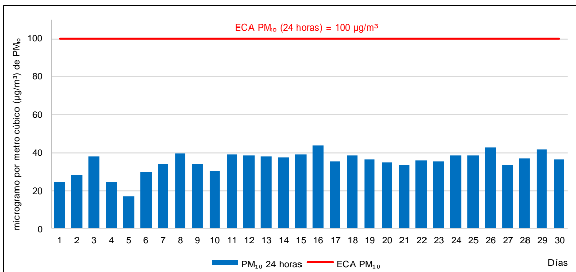
Figura 5.3. Concentraciones de 24 horas de PM 10 en la estación de vigilancia ambiental CA-TO-01 en abril de 2019
