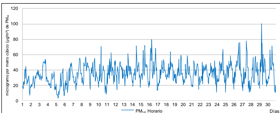
Figura 5.4. Concentraciones horarias de PM 10 en la estación de vigilancia ambiental CA-TO-01 en abril de 2019
