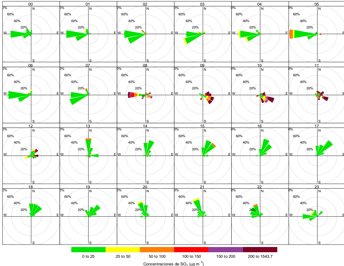
Figura 5.5. Rosas de concentración por horas para el SO 2 en la estación de vigilancia ambiental CA-CC-01, desde las 00:00 horas hasta las 23:00 horas en julio de 2019 Nota: Las paletas indican la dirección de donde provienen las concentraciones de SO 2 .
