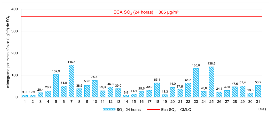
Figura 5.3. Concentraciones de 24 horas de SO 2 en la estación de vigilancia ambiental CA-CC-01, en julio de 2019
