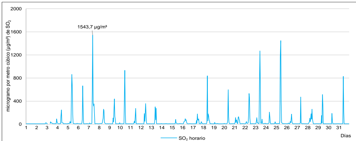
Figura 5.4. Concentraciones horarias de SO 2 en la estación de vigilancia ambiental CA-CC-01 en julio de 2019.
