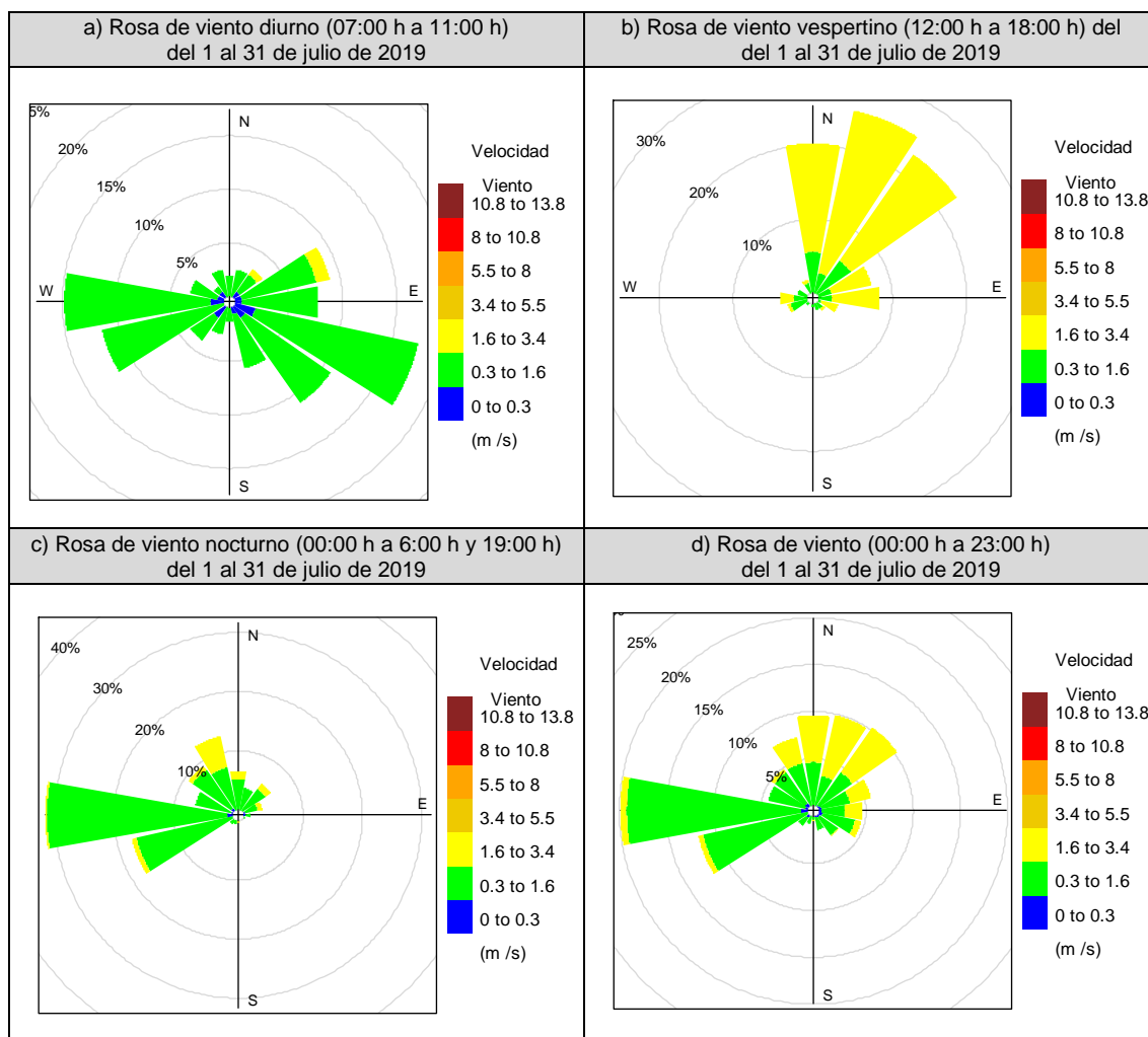
Figura 5.1. Representación gráfica de las rosas de vientos en la estación de vigilancia ambiental CA-CC-01, en julio de 2019 a) en horario diurno, b) en horario vespertino, c) en horario nocturno, d) en todas las horas del mes.
