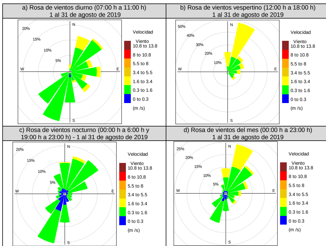
Figura 5.1. Representación gráfica de las rosas de vientos en la estación de vigilancia ambiental CA-SB-01, en agosto de 2019 a) en horario diurno, b) en horario vespertino, c) en horario nocturno, d) en todas las horas del mes
