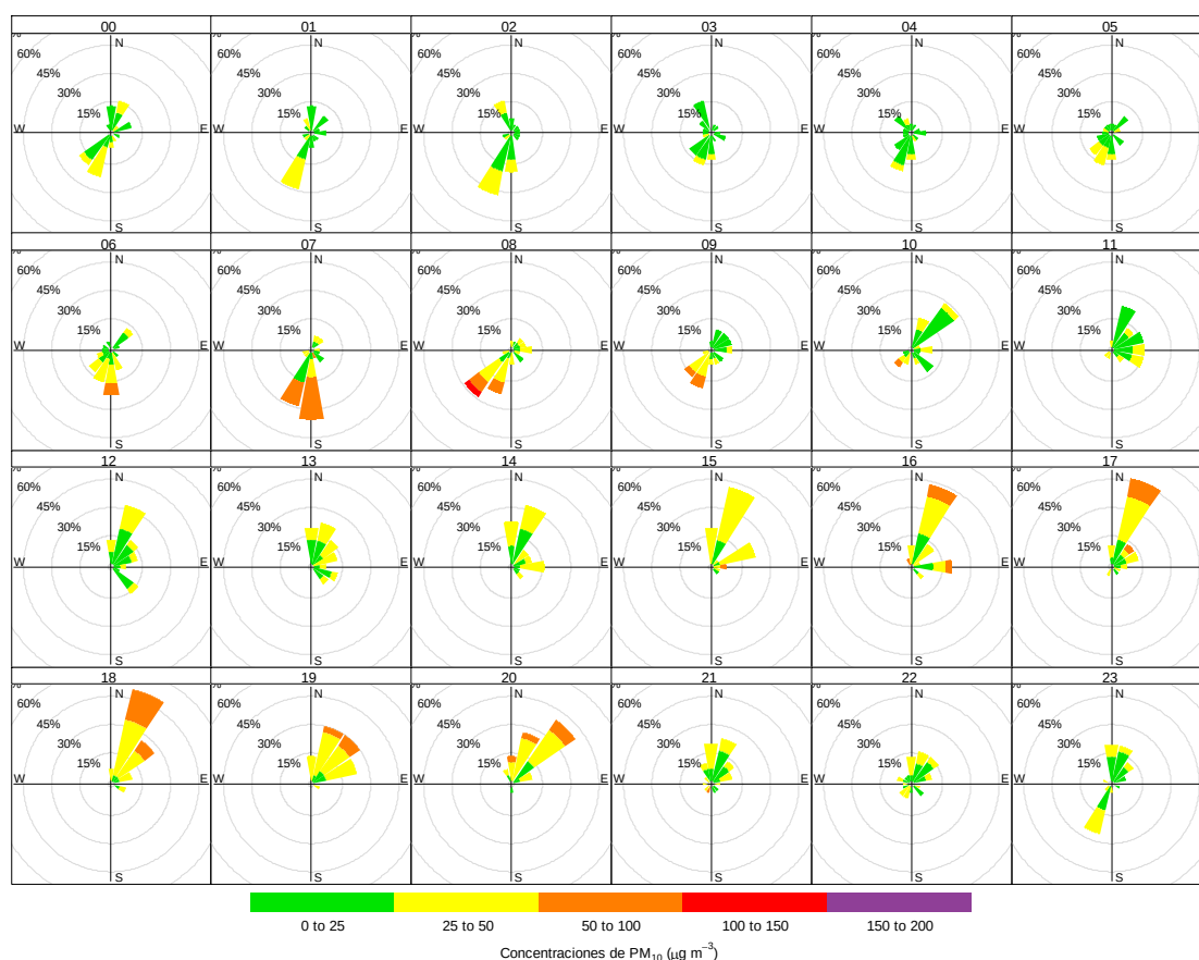
Figura 5.5. Rosas de concentración por horas de PM_{10} en la estación de vigilancia CA-SB-01, desde las 00:00 horas hasta las 23:00 horas, en agosto de 2019
