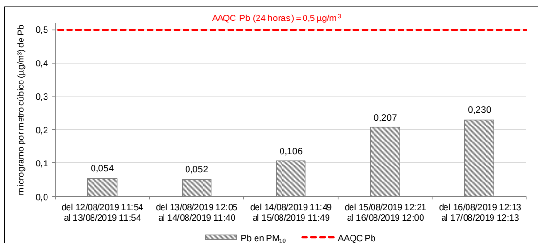
Figura 5.6. Concentraciones de plomo en material particulado con diámetro menor a 10 micras (Pb en PM 10 ) a 10°C y de 24 horas en agosto 2019, de la estación de vigilancia ambiental de la calidad del aire CA-SB-01, comparadas de manera referencial con la normativa canadiense AAQC-2012.
