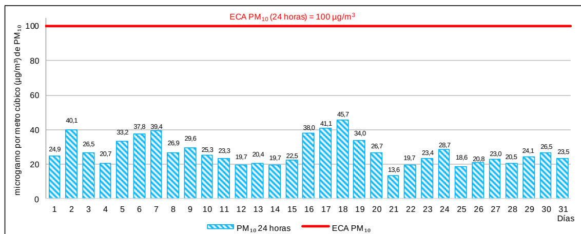
Figura 5.3. Concentraciones de 24 horas de PM_{10} en la estación de vigilancia ambiental CA-SB-01, agosto de 2019.
