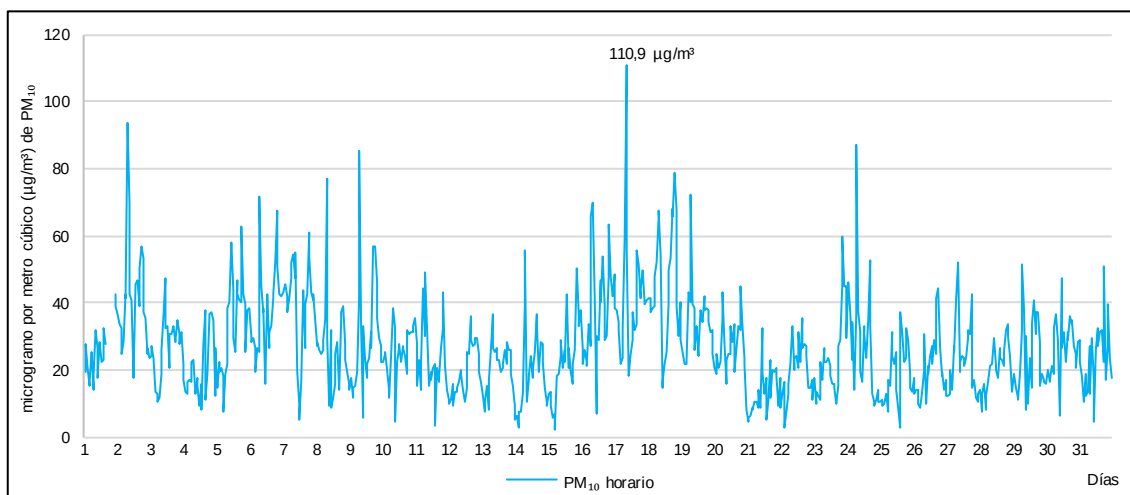
Figura 5.4. Concentraciones horarias de PM_{10} en la estación de vigilancia ambiental CA-SB-01 en agosto de 2019.
