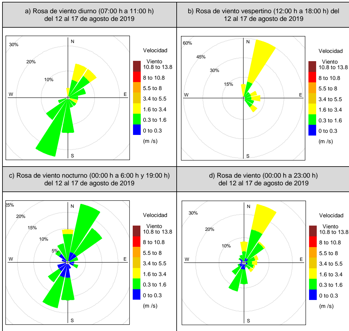
Figura 5.1. Rosas de vientos en el distrito de Simón Bolívar de 12 al 17 de agosto de 2019 a) en horario diurno, b) en horario vespertino, c) en horario nocturno, d) en todas las horas.
