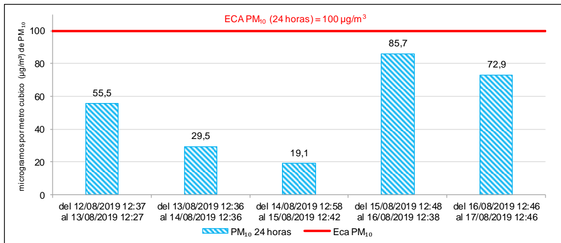
Figura 5.3. Concentraciones de 24 horas de PM 10 en la estación de vigilancia ambiental CA-SB-02, del 12 al 17 de agosto de 2019.
