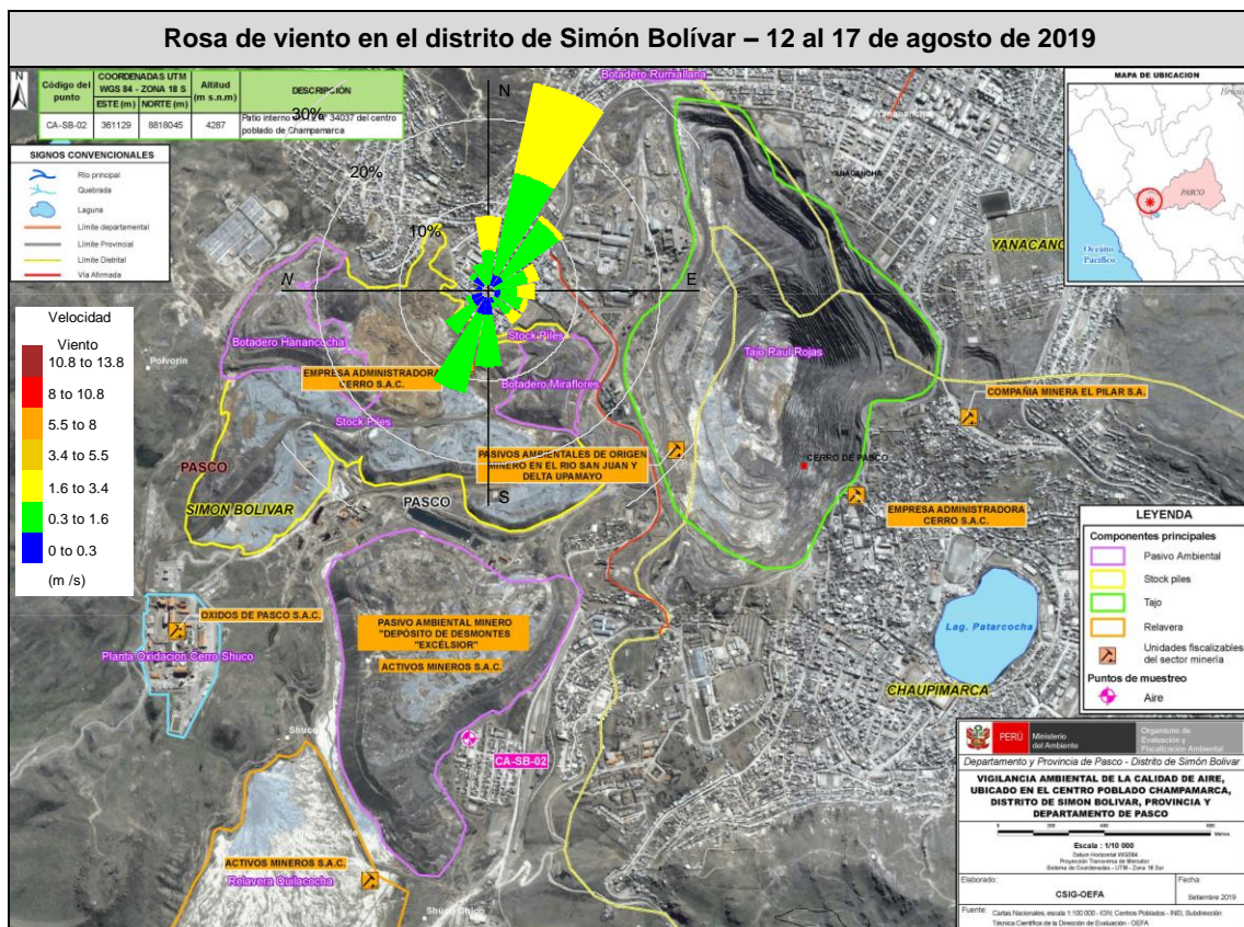
Figura 5.2. Ubicación de la estación meteorológica en el distrito de Simón Bolívar y rosa de vientos de los días 12 al 17 de agosto de 2019, respecto a la ubicación de la estación CA-SB-02. Referencia: Imágenes satelitales extraídas de Google Earth.
