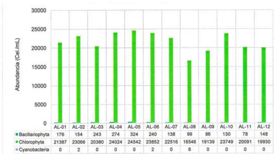
Gráfico N° 17. Abundancia de Fitoplancton
