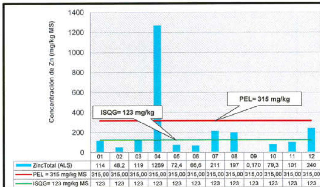
Gráfico N° 24. Concentraciones de zinc en sedimento
