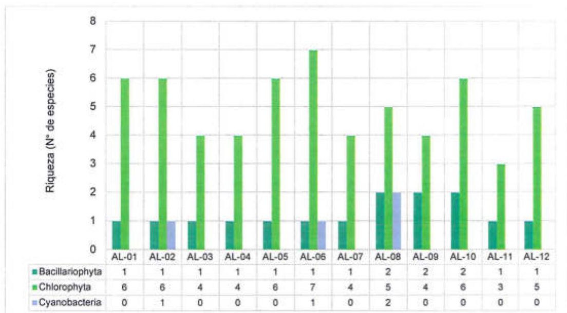
Gráfico N° 16. Riqueza de Fitoplancton
