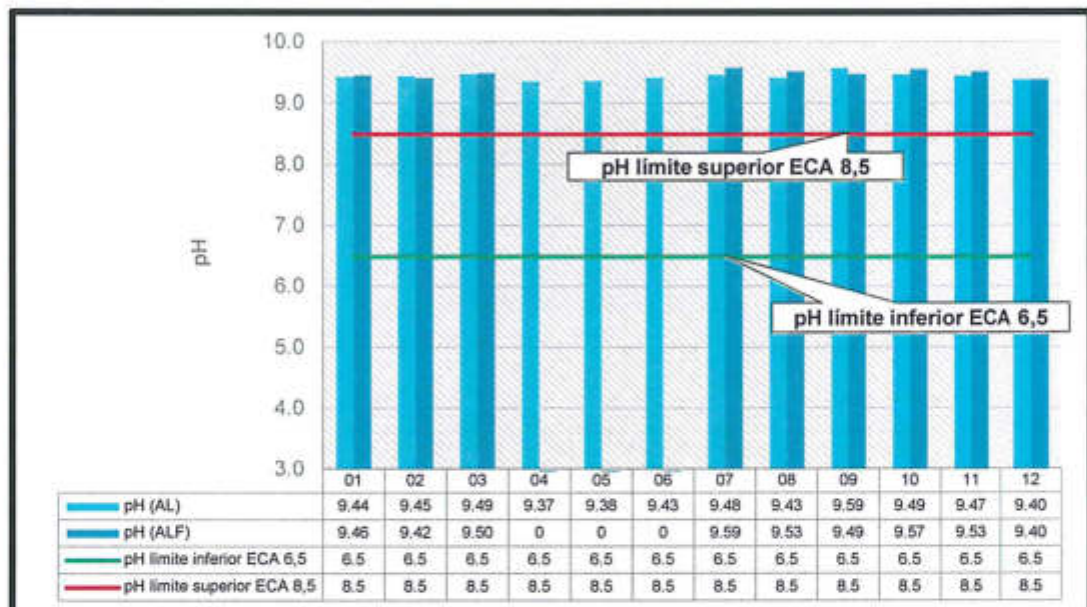
Gráfico N° 8. Niveles de pH
