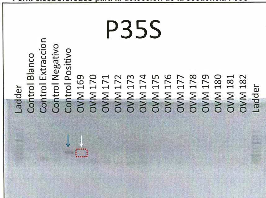
Figura N° 1 Perfil electroforético para la detección de la secuencia P35S
