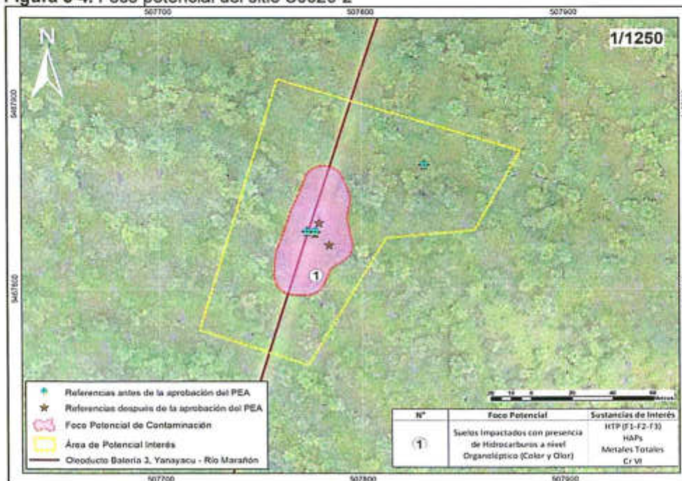
Figura 3-4. Foco potencial del sitio S0020-2
