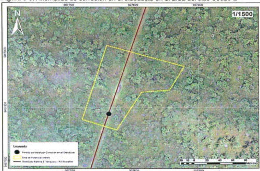
Figura 3-3. Anomalías de corrosión en el oleoducto en el área del sitio S0020-2
