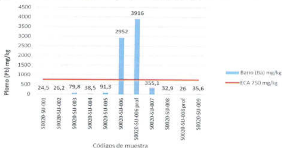
Figura 8-4. Concentraciones de bario (Ba) en el sitio S0020-2
