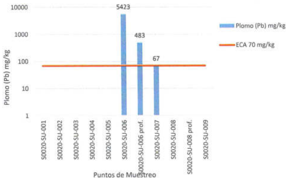
Figura 8-6. Concentraciones de plomo (Pb) en el sitio S0020-2
