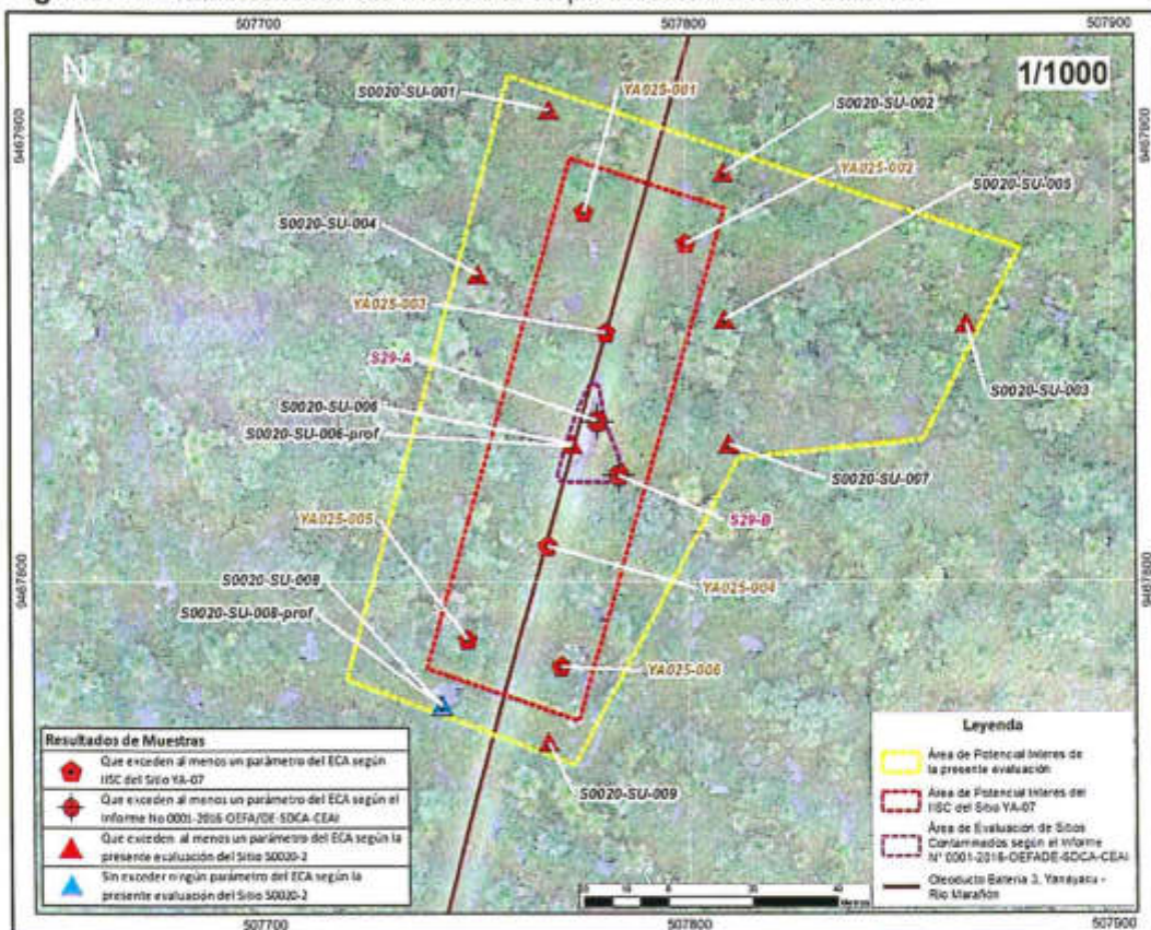
Figura 9-1. Resultados de las muestras disponibles en el sitio S0020-2
