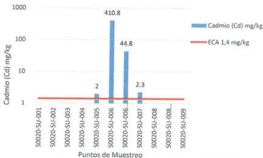
Figura 8-5. Concentraciones de cadmio (Cd) en el sitio S0020-2
