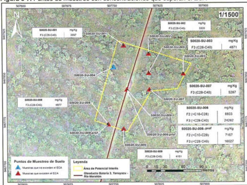
Figura 8-7. Puntos de muestreo con concentraciones que superan el ECA
