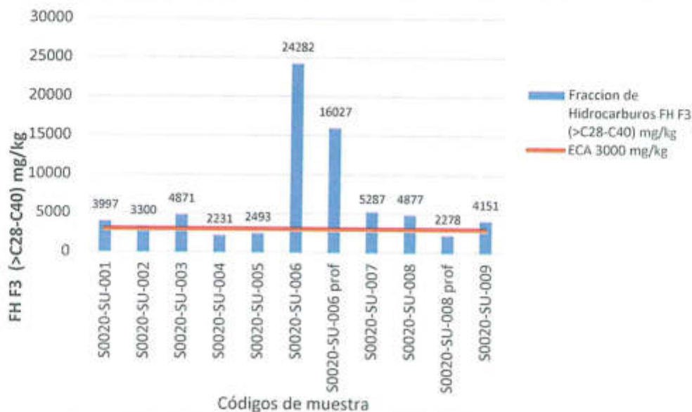
Figura 8-2. Concentraciones de fracción de hidrocarburos F3 en el sitio S0020-2
