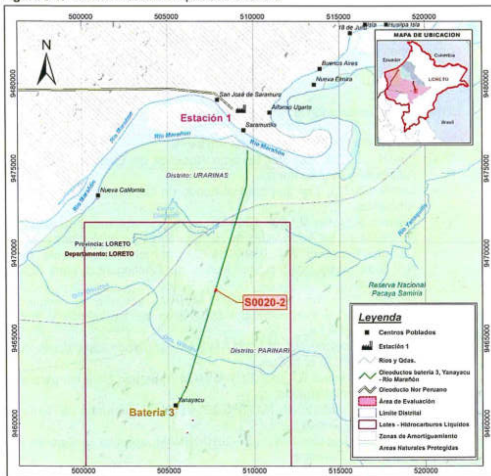
Figura 3-1. Ubicación del sitio impactado S0020-2
