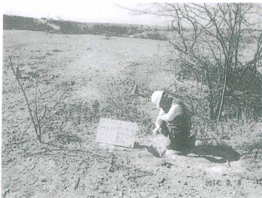
Fotografía N° 1. Toma de muestra de suelo en el punto F01867-SU01, ubicado a 1 m aproximadamente del Pozo T4238.
