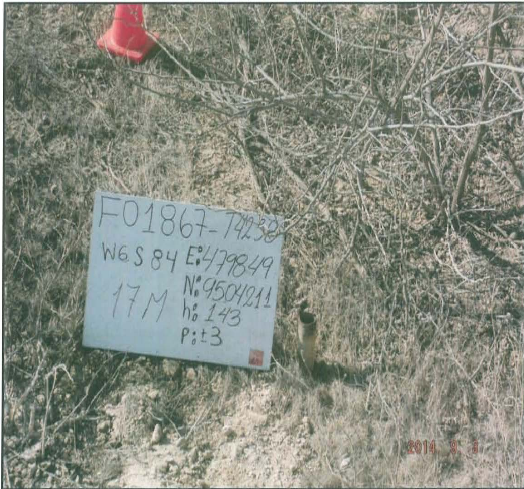
Fotografía N° 1. Se visualiza tubo de 2 plg que sobresale a una altura de 0,2 m desde la superficie del suelo.
