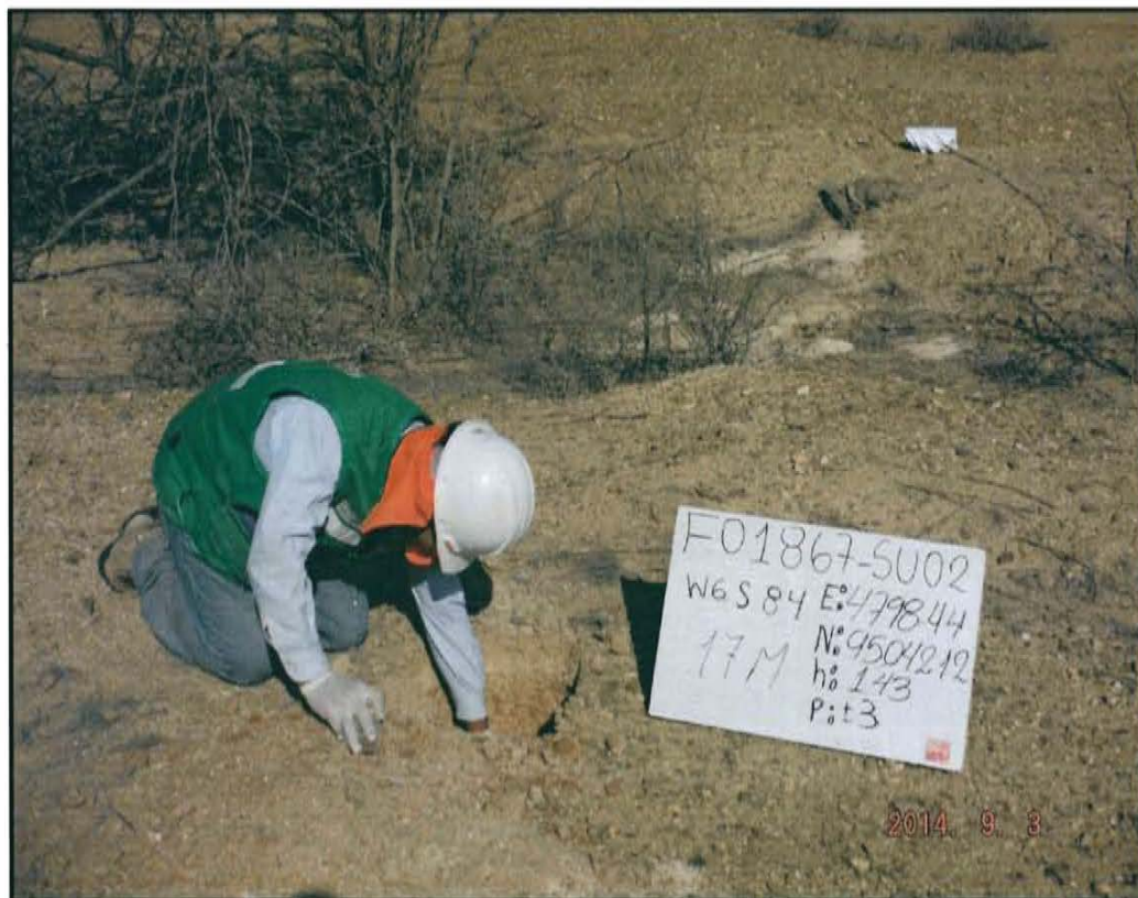
Fotografía N° 4. Muestra tomada aproximadamente a 3 m al oeste del pozo.
