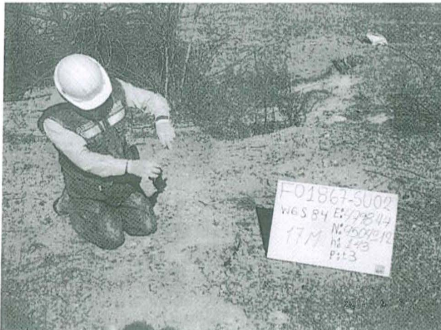
Fotografía N° 2. Toma de muestra de suelo en el punto F01867-SU02, ubicado a 3 m aproximadamente del Pozo T4238.
