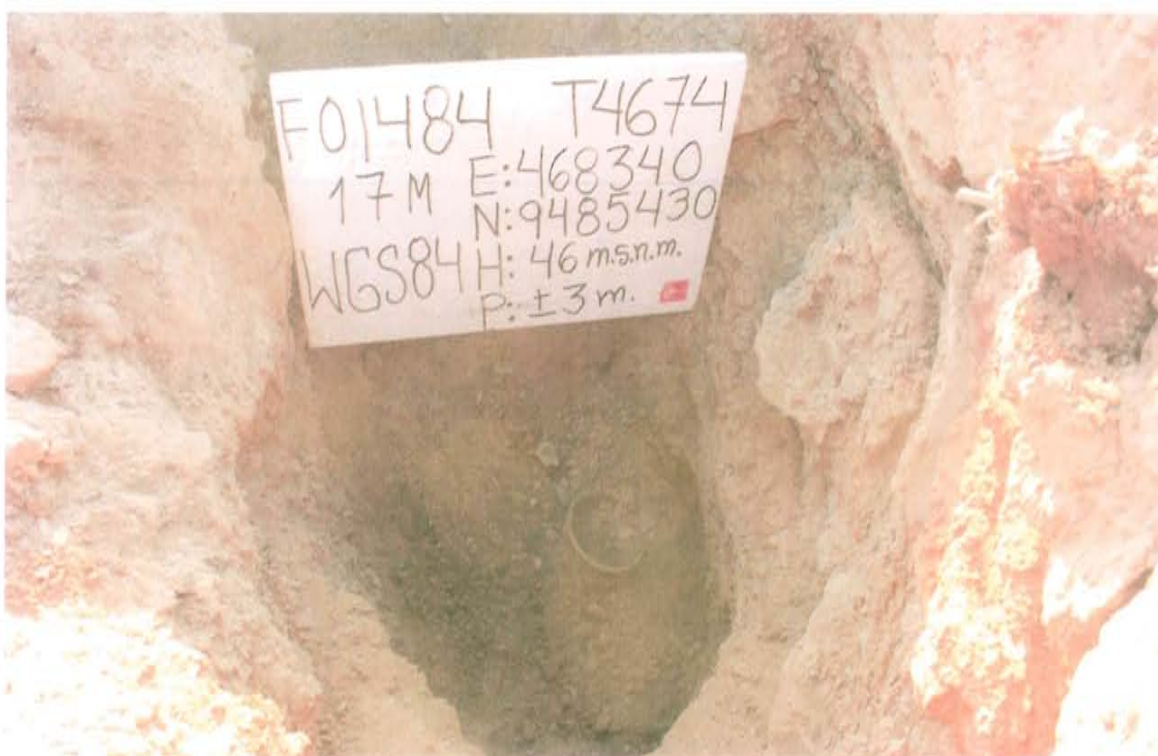
Fotografía N° 1. Identificación del pozo inactivo con código PERUPETRO T4674. Presenta casing cortado y apenas visible en el interior de una excavación, sin elementos de cierre, por lo que se considera abierto.
