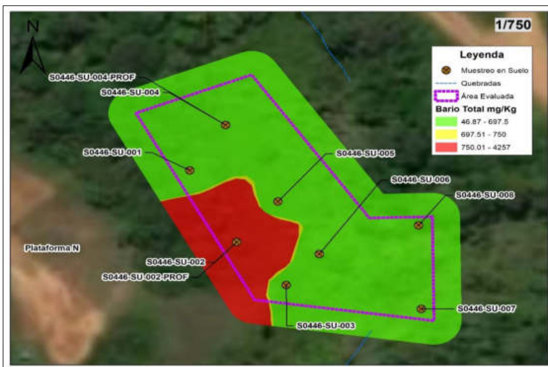
Figura 9.2. Modelamiento de la concentración de bario total para el sitio S0446
