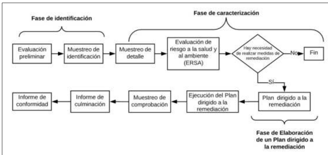
Figura 1.1. Flujograma de la gestión de sitios contaminados.
