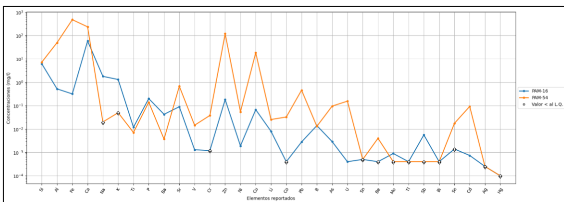
Figura 6.5. Concentraciones de metales en la prueba de lixiviación shake flask metales en muestras de residuos mineros
