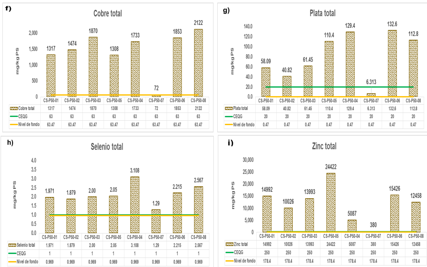
Figura 6.74. Concentraciones de f) cobre, g) plata, h) selenio y i) zinc en el API PAM 50 comparados con los valores de la guía canadiense de suelo, uso agrícola y valores del nivel de fondo
