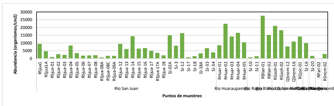
Figura 6.31. Abundancia total de organismos/cm 2 de perifiton vegetal en agosto de 2020
