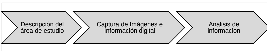
Figura 5.9. Secuencia de pasos para el análisis de la información
