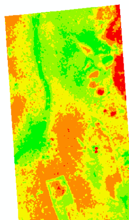
Figura 7.57. Índice de vegetación (NDVI y NDRE) de la formación vegetal césped con parches de bofedal del API PAM 20
