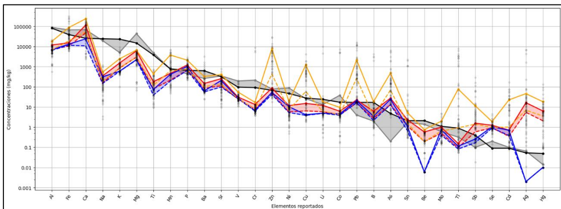
Figura 6.22. Diagrama spider de los umbrales de niveles de fondo hallados mediante los métodos y criterios de la media (línea roja), la mediana (línea azul) y diagrama de cajas y bigotes (línea amarilla), para la distribución de elementos en la subcuenca del río San Juan
