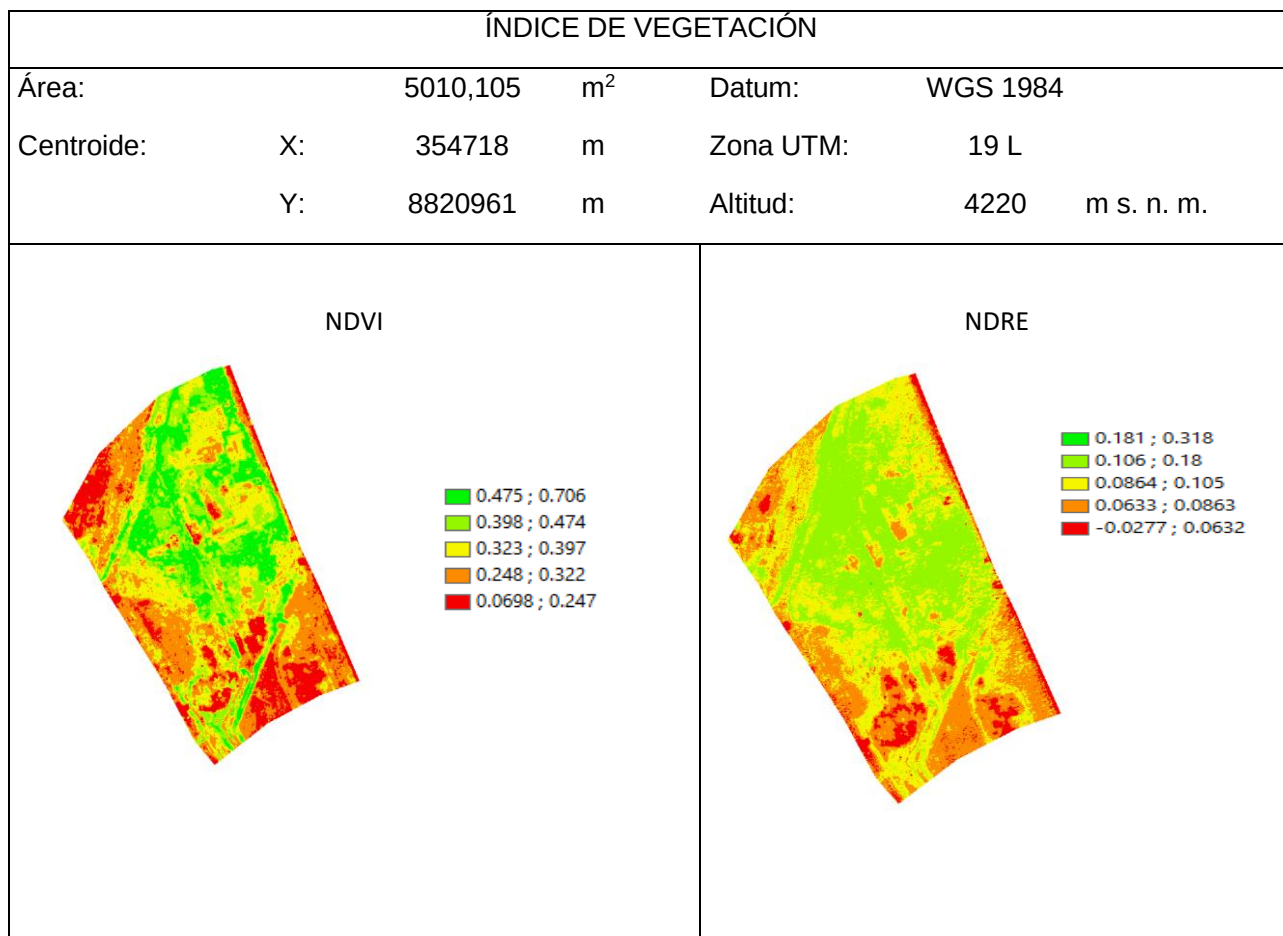
Figura 7.75. Índice de vegetación (NDVI y NDRE) de la formación vegetal bofedal con parches de césped del API PAM 22
