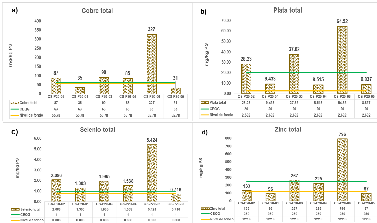
Figura 6.36. Concentraciones de a) cobre, b) plata, c) selenio y d) zinc en el API PAM 20, comparados con los valores de la guía canadiense de suelo, uso agrícola y valores del nivel de fondo
