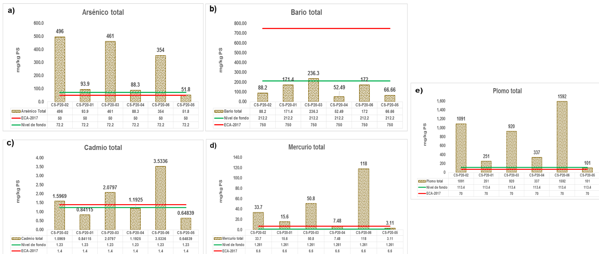
Figura 6.35. Concentraciones de a) arsénico, b) bario, c) cadmio, d) mercurio y e) plomo en el API PAM 20, comparados con los valores de los ECA para suelo 2017, uso agrícola y valores del nivel de fondo
