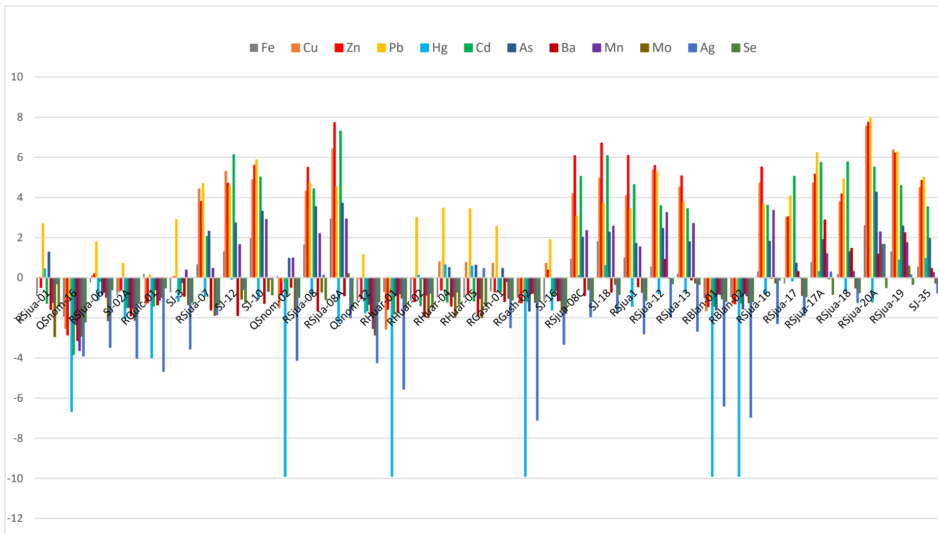
Figura 7.41. Índices de geo acumulación en los sedimentos del río San Juan y tributarios
