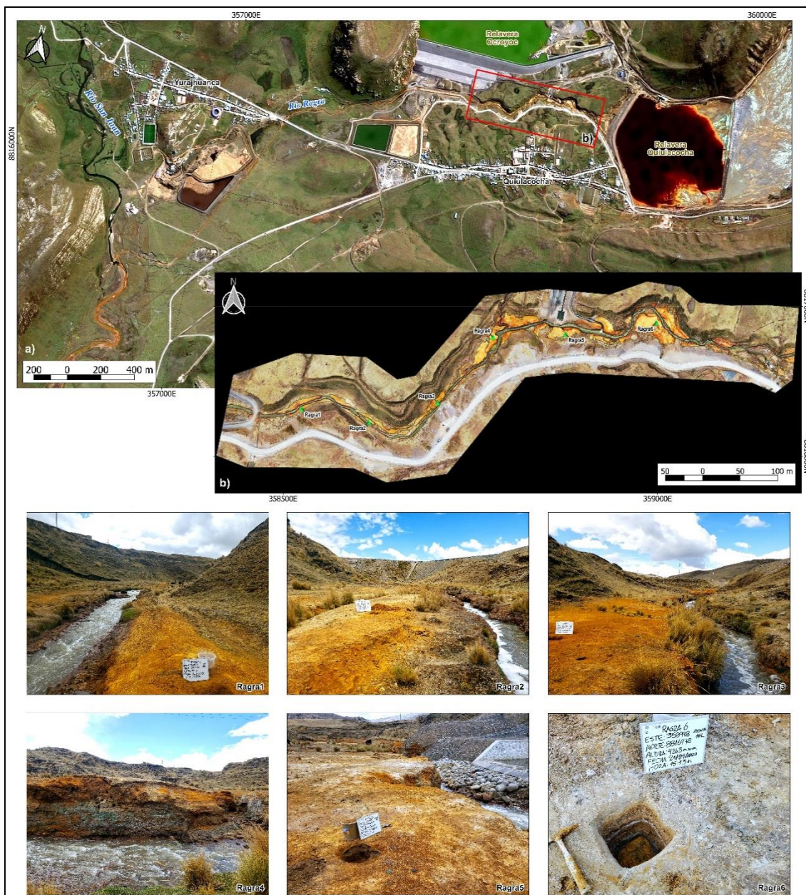
Figura 7.9. Sedimentos cuaternarios fluviales y fluvio-aluviales del río Ragra con residuos mineros
