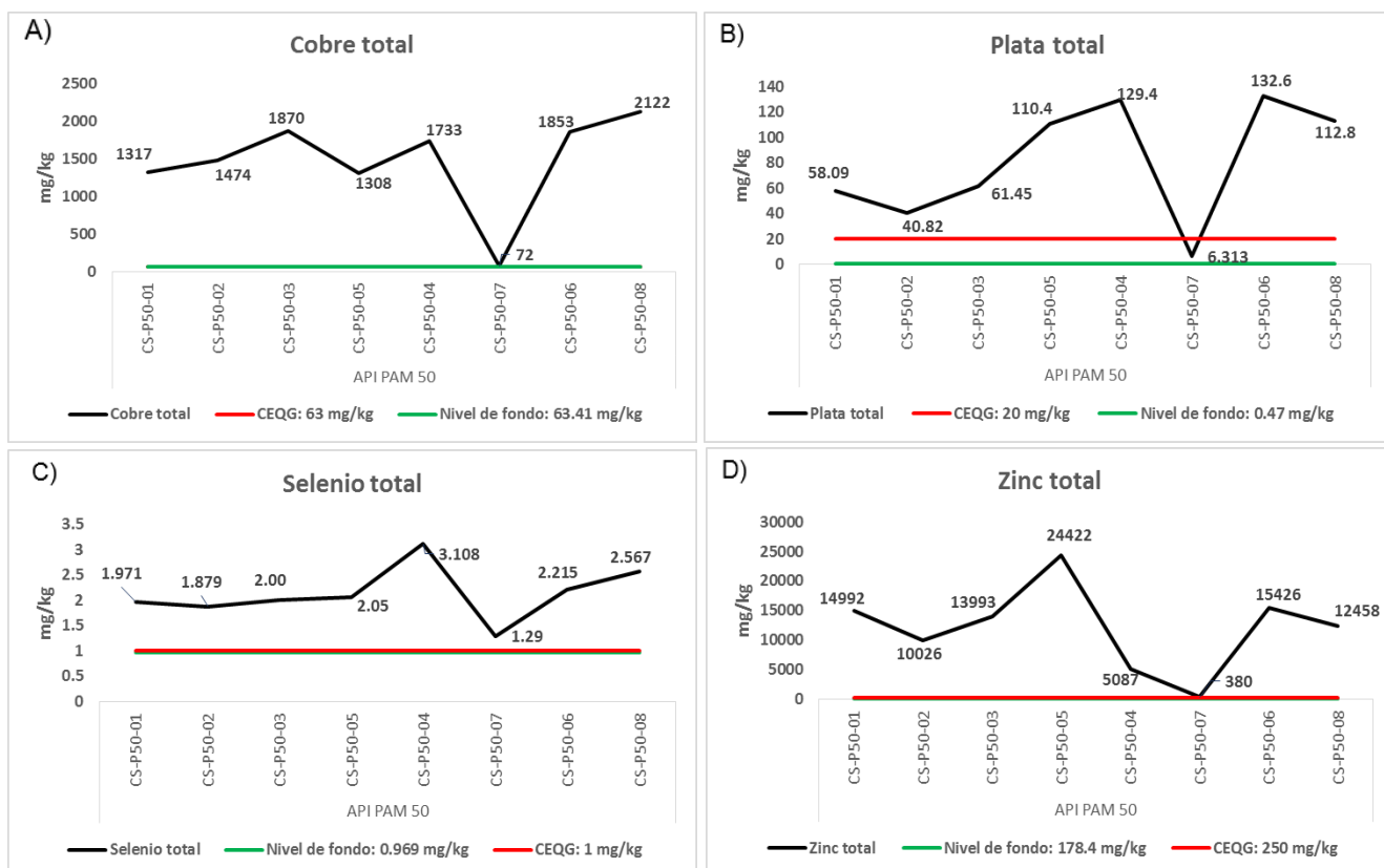
Figura 7.118. Concentraciones de A) cobre, B) plata, C) selenio y D) zinc en el API PAM 50, comparadas con los valores de la guía canadiense de suelo, uso agrícola y los valores del nivel de fondo
