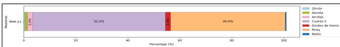
Figura 6.3. Resultado de análisis mineralógico por microscopía óptica, que muestra la distribución de los minerales reportados en PAM-23
