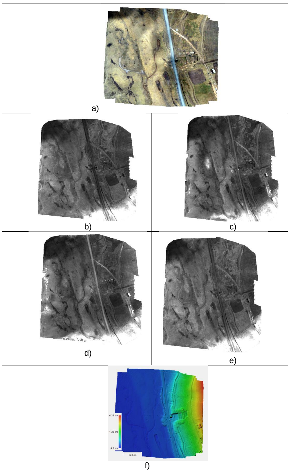
Figura 6.39. a) Ortofoto RGB, b) NIR c) Red, d) Green, e) Red Edge) y f) DEM del API PAM 20
