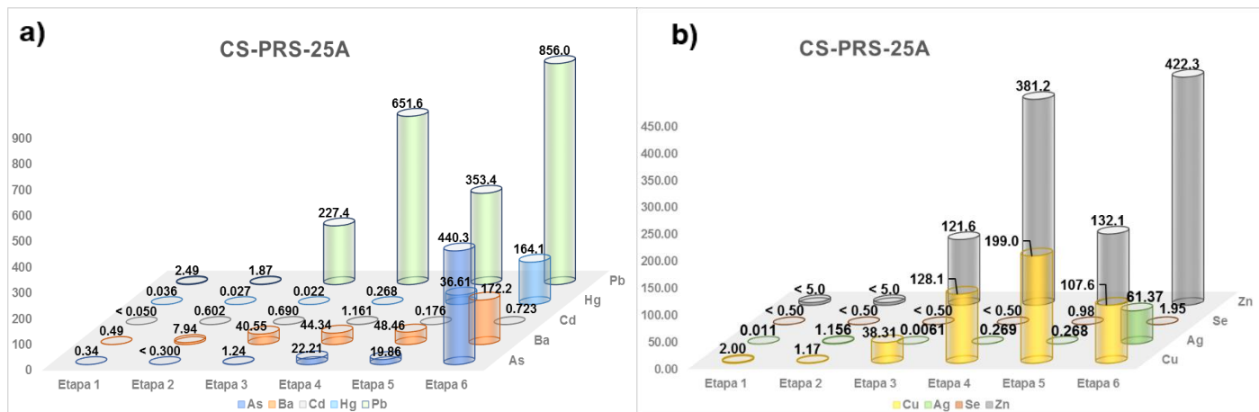
Figura 6.54. Disponibilidad por etapas de metales a) arsénico, bario, cadmio, mercurio y plomo, y b) cobre, plata, selenio y zinc, en el punto CS-PRS-25A (muestreo superficial) del API PRS
