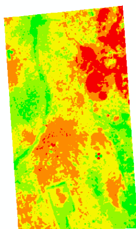
Figura 7.57. Índice de vegetación (NDVI y NDRE) de la formación vegetal césped con parches de bofedal del API PAM 20
