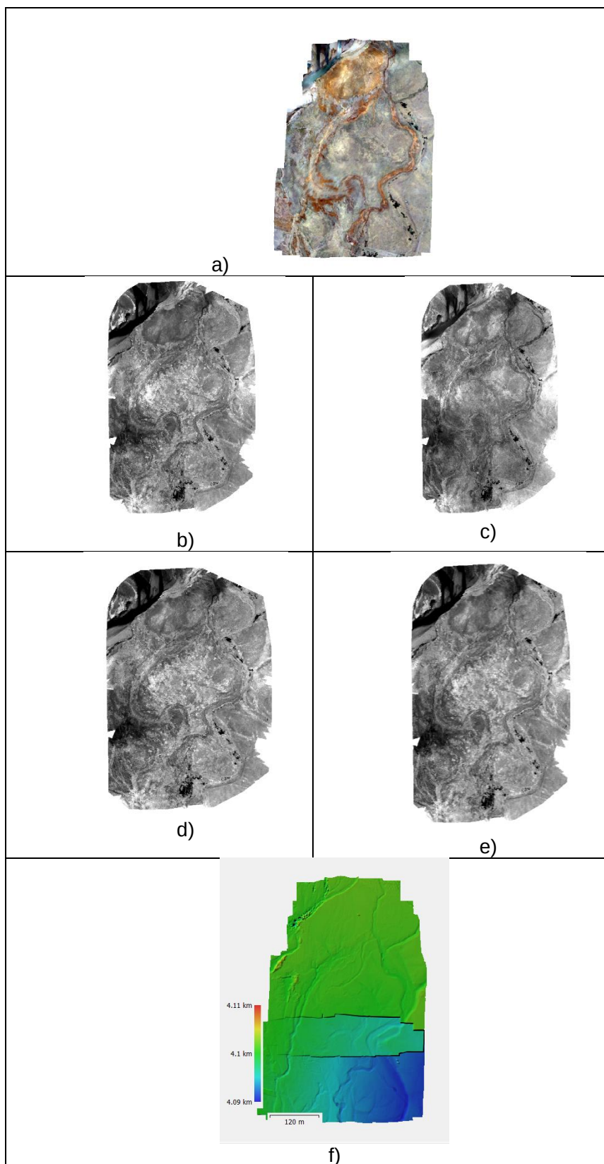
Figura 6.70. a) Ortofoto RGB, b) NIR c) Red, d) Green, e) Red Edge), y f) DEM del API DR
