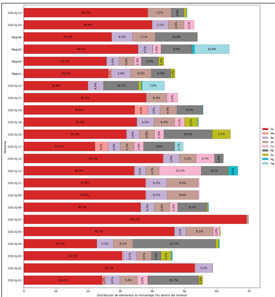
Figura 7.3. Distribución de elementos de interés de acuerdo a la presencia de minerales en traza, reportados en el análisis mineralógico por microscopia electrónica de barrido en muestras de roca (sedimentos fluviales y fluvio-aluviales de los ríos San Juan y Ragra respectivamente), ordenados desde la cabecera de subcuenca hacia el delta Upamayo
