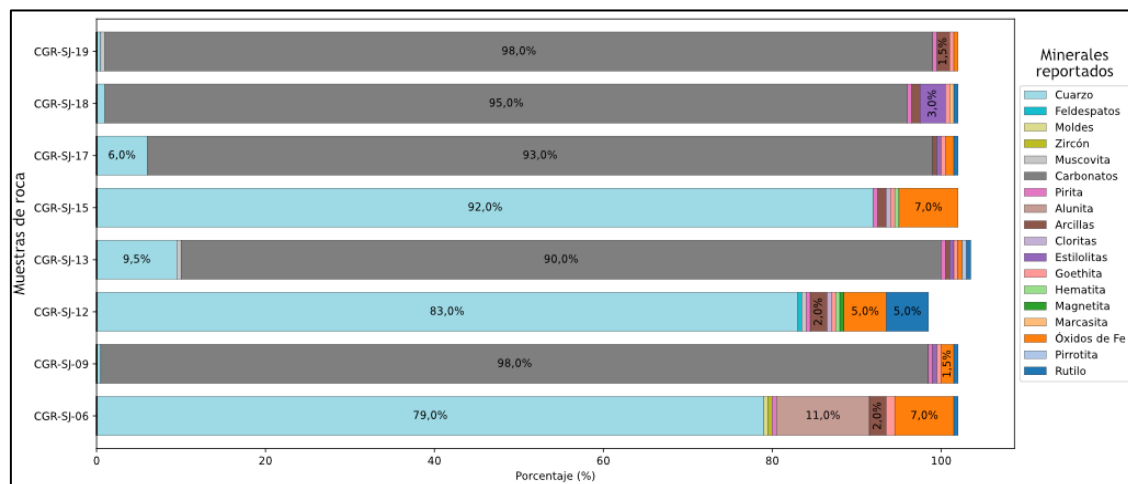
Figura 6.14. Resultado de análisis mineralógico por microscopia óptica, que muestra la distribución de los minerales reportados en muestras de roca
