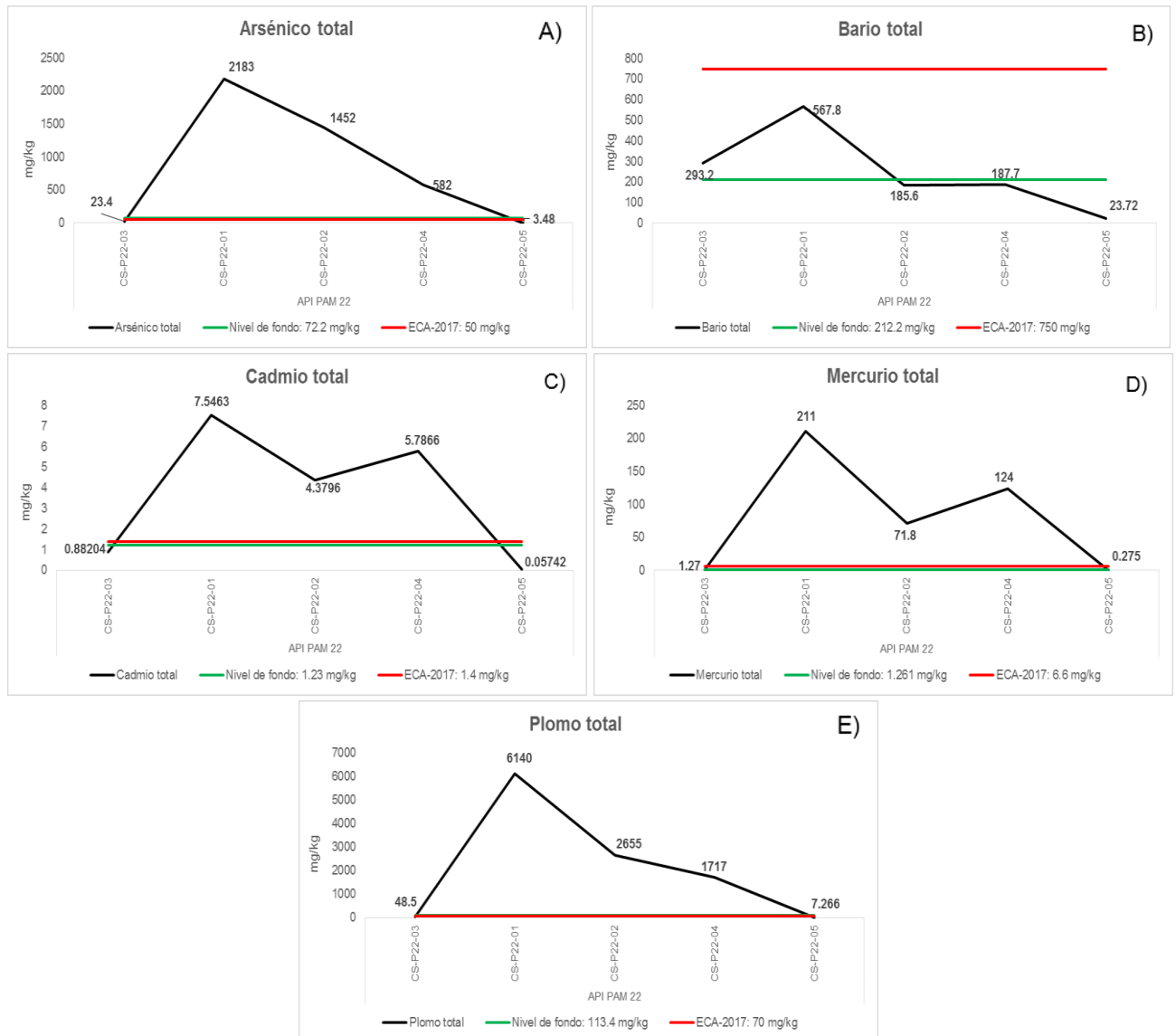
Figura 7.69. Concentraciones de A) arsénico, B) bario, C) cadmio, D) mercurio y E) plomo en el API PAM 22, comparadas con los valores de los ECA para suelo 2017, uso agrícola y valores de nivel de fondo
