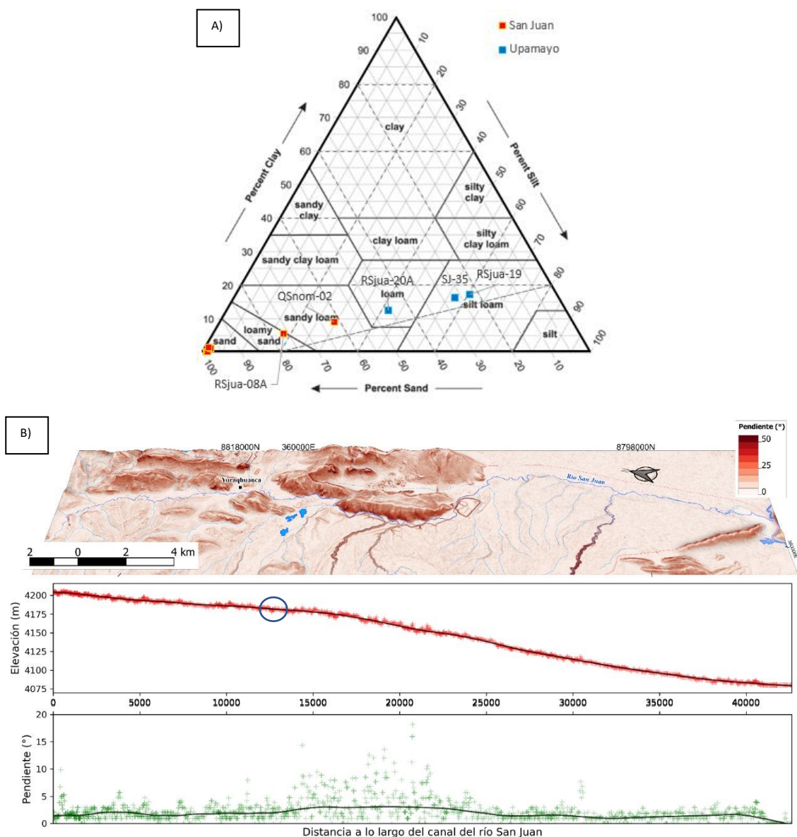
Figura 7.38. A) Textura arena arcillosa en el punto RSjua-08A, los puntos RSJuan-07, SJ-12, SJ-10, RSJuan-08 presentan textura arenosa, y B) mapa de pendientes y perfiles de elevación a lo largo del río San Juan, que muestra el suave relieve y las bajas pendientes dominantes de la zona de evaluación, lo que condiciona los desbordes del río San Juan en épocas de avenida extraordinarias
