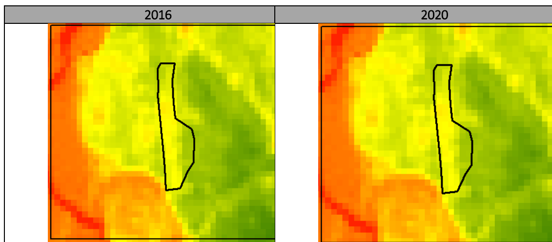
Figura 7.122. NDVI de las imágenes satelitales Sentinel 2A de abril para 2016 y de junio para 2020
