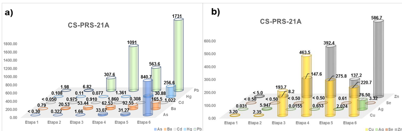
Figura 6.55. Disponibilidad por etapas de metales a) arsénico, bario, cadmio, mercurio y plomo, y b) cobre, plata, selenio y zinc, en el punto CS-PRS-21A (muestreo superficial) del API PRS
