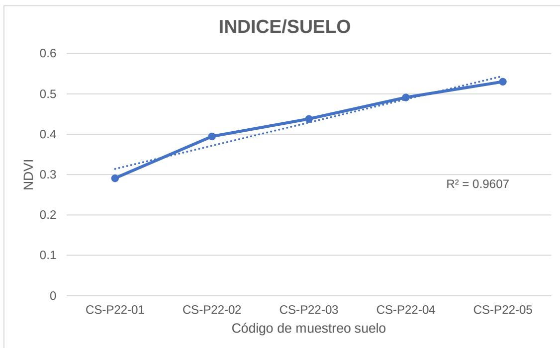
Figura 6.48. Índice de vegetación (NDVI) y muestreo de suelo
