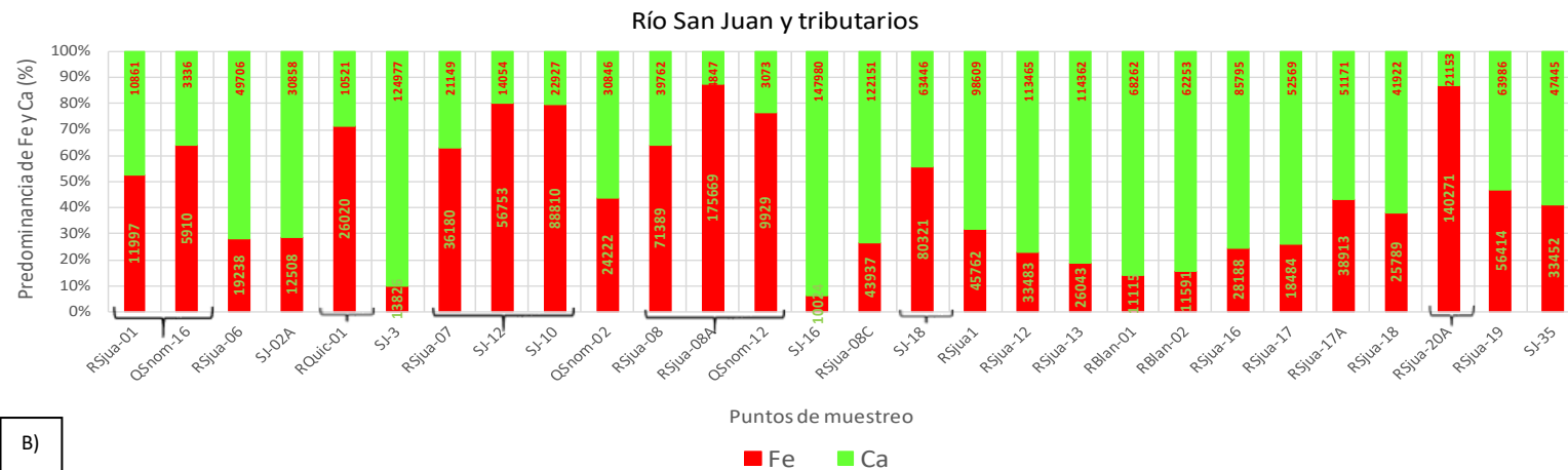
Figura 7.32. A) Comparación de las concentraciones de Fe, Al, As, Pb, Zn, Cd, Hg, Cu, Ni, Ca, Mn, Ba, Mo, Ag entre los sedimentos del río San Juan y sus tributarios, y B) predominancia de hierro y calcio (%)
