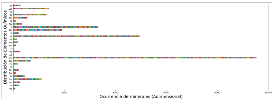
Figura 6.18. Distribución de elementos químicos según la ocurrencia de minerales a lo largo del río San Juan, según el análisis mineralógico por microscopia electrónica de barrido en roca (sedimentos fluviales y fluvio-aluviales de los ríos San Juan y Ragra respectivamente)
