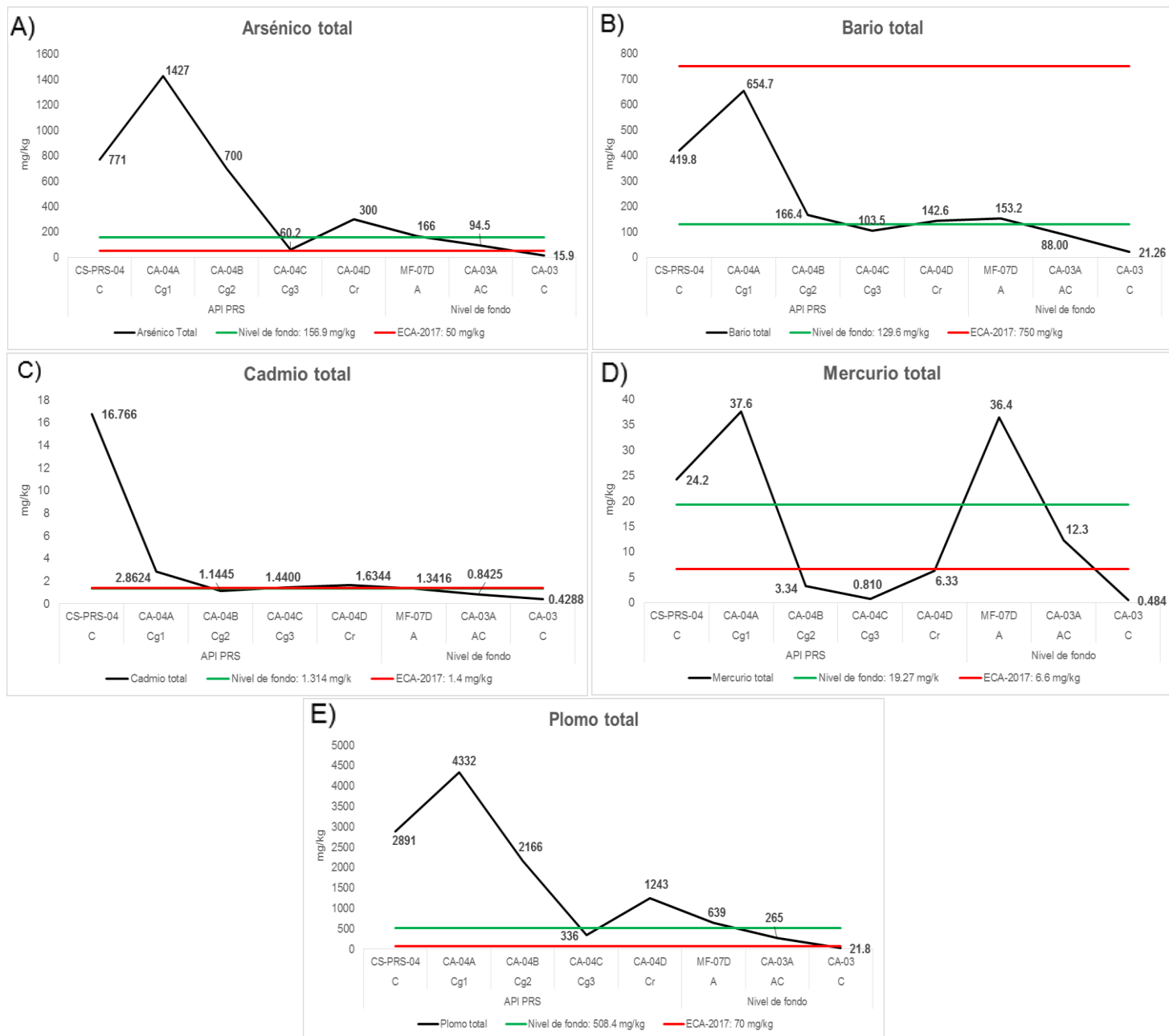
Figura 7.83. Concentraciones de A) arsénico, B) bario, C) cadmio, D) mercurio y E) plomo en calicatas del API PRS y del nivel de fondo D, comparadas con los valores de los ECA para suelo 2017, uso agrícola y los valores de nivel de fondo
