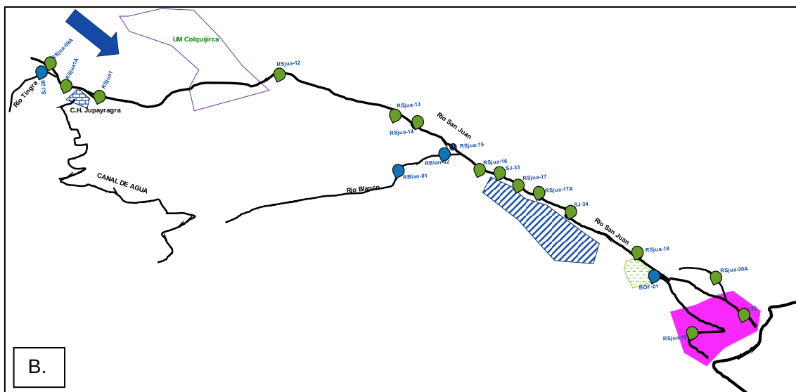
Figura 6.26. Representación gráfica del ICA-PE en el río San Juan y aportantes a) parte alta y B) parte baja.
