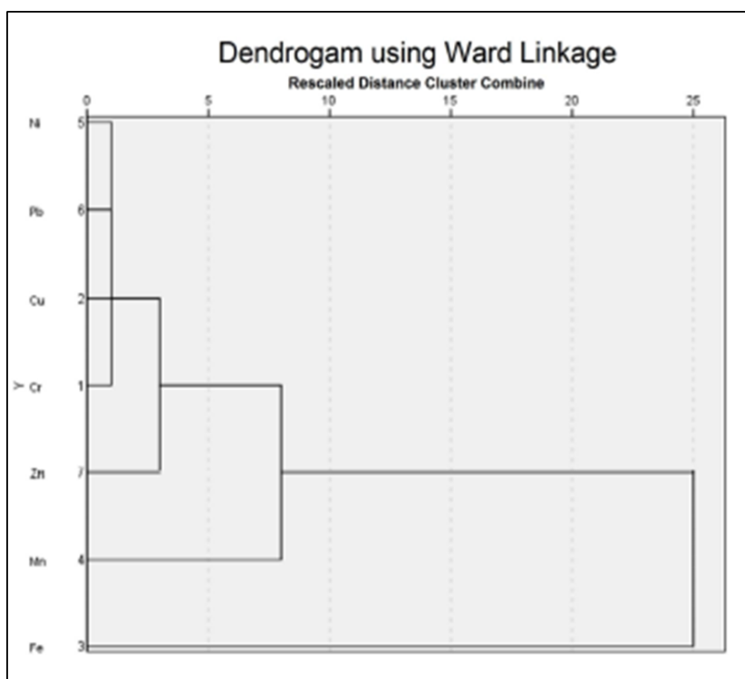
Figura 5.6. Dendrograma
