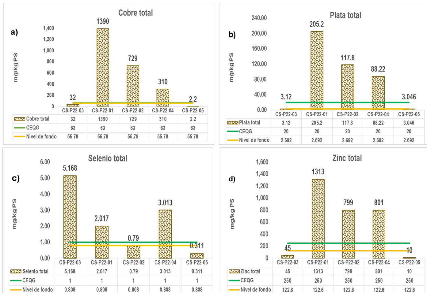
Figura 6.45. Concentraciones de a) cobre, b) plata, c) selenio y d) zinc en el API PAM 20, comparados con los valores de la guía canadiense de suelo, uso agrícola y valores del nivel de fondo
