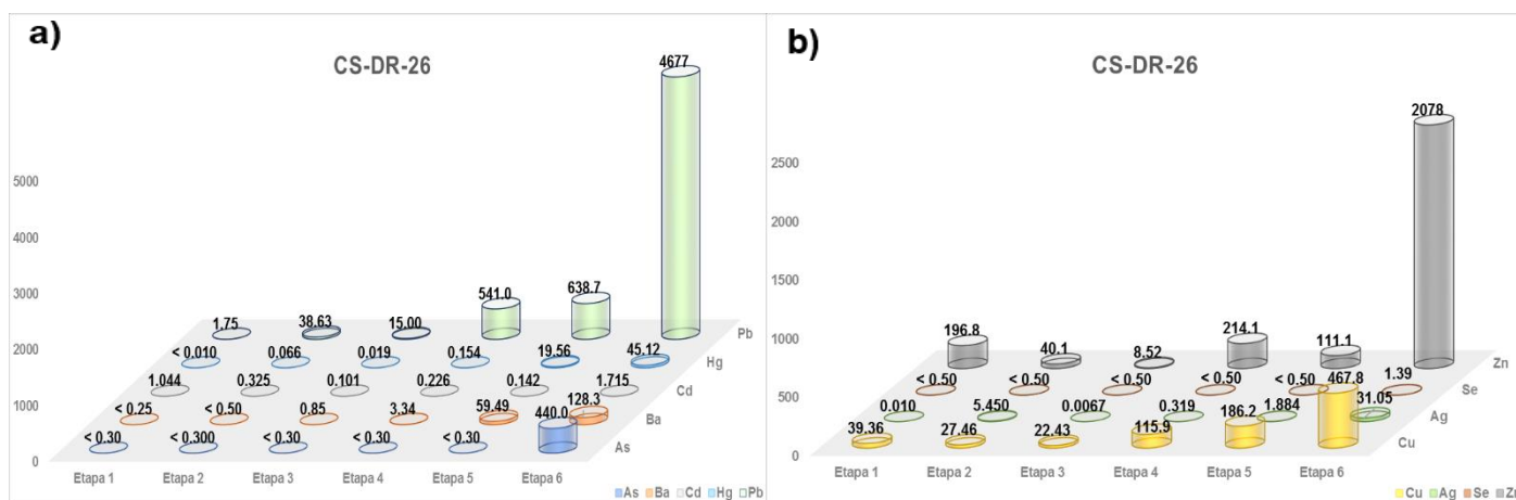
Figura 6.66. Disponibilidad por etapas de metales a) arsénico, bario, cadmio, mercurio y plomo; y b) cobre, plata, selenio y zinc, en el punto CS-DR-26 (muestreo superficial) del API DR
