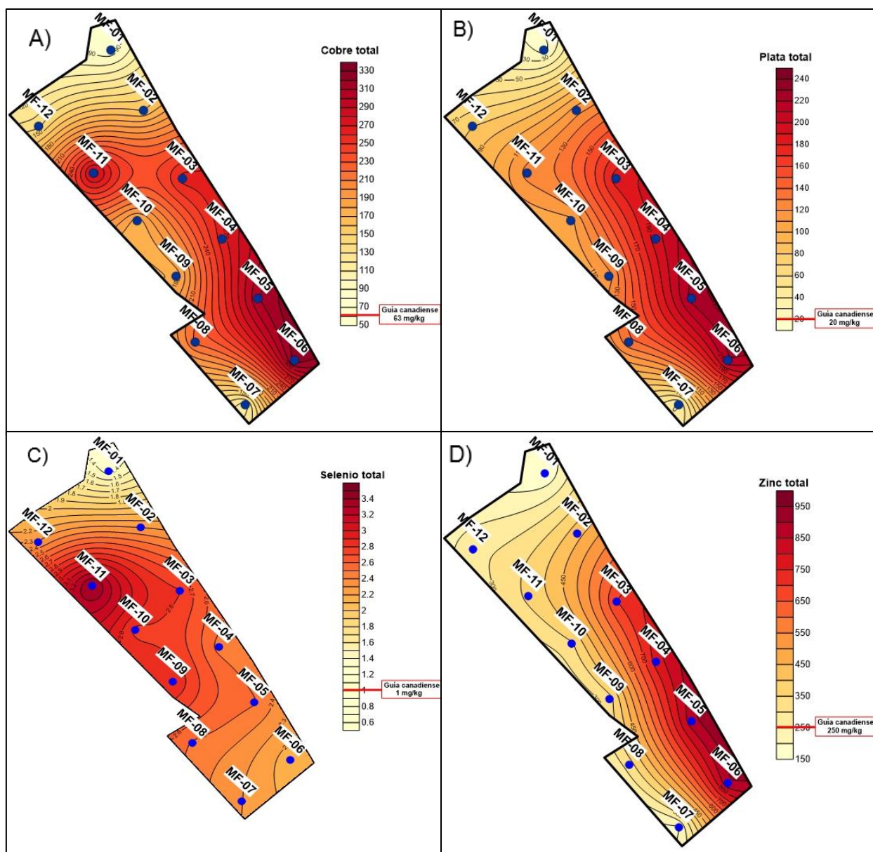
Figura 7.65. Distribución espacial de concentraciones de A) cobre, B) plata, C) selenio y D) zinc registradas en el API MF, comparadas con los valores de la guía canadiense, uso agrícola
