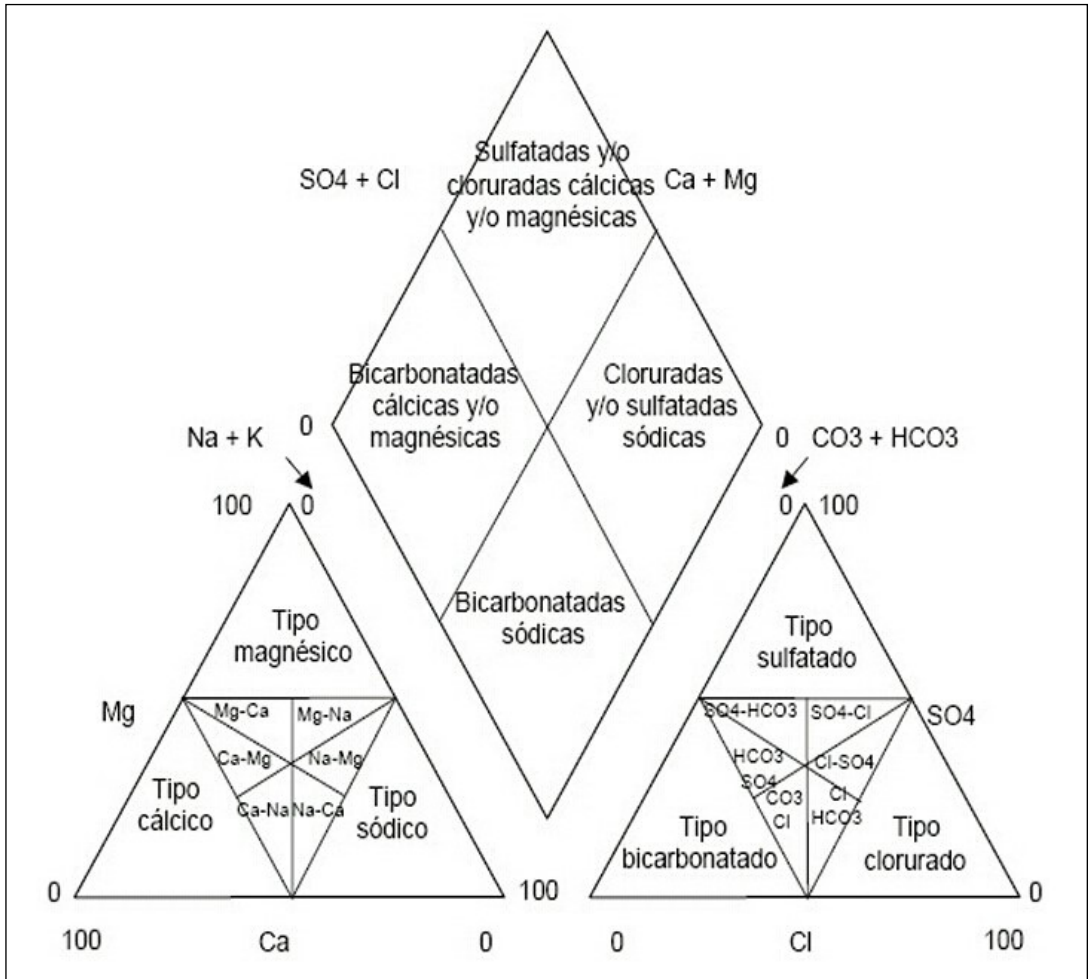
Figura 3 Diagrama de Piper.
