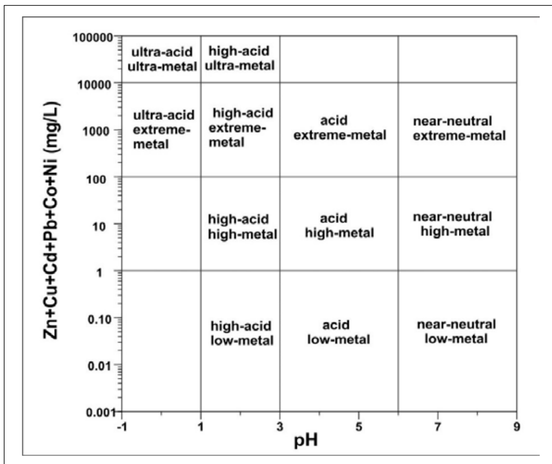
Figura 4 Diagrama de Ficklin.
