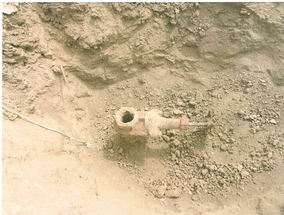
Fotografía N° 1. El Pozo T4257 fue ubicado con ayuda del detector de metales a 0,6 m aproximadamente, se observa tubería de reducción de 2,5 pulgadas la cual se encuentra abierta y expuesta al ambiente y una válvula lateral en estado de corrosión.
