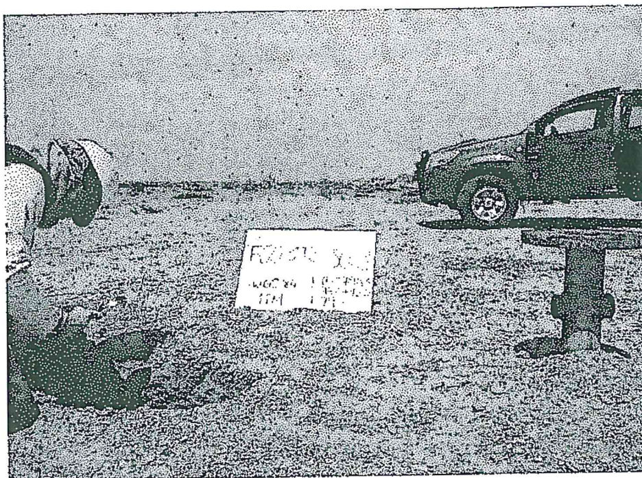
Fotografía N° 1. Toma de muestra de suelo en el punto F00392-SU01, ubicado a 1,36 m aproximadamente del Pozo T2673.
