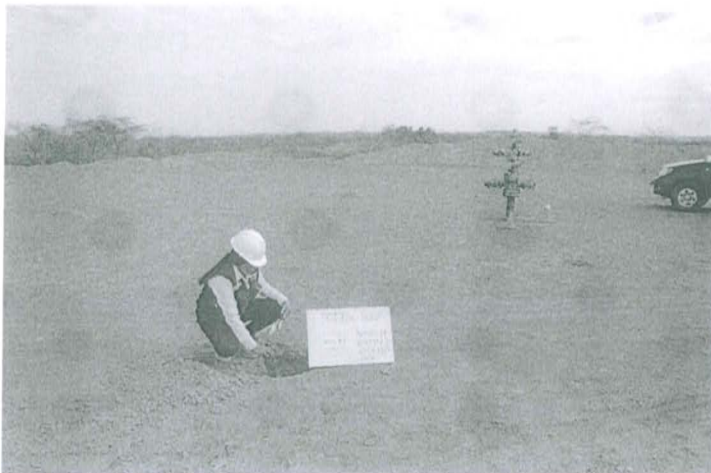
Fotografía N° 2. Toma de muestra de suelo en el punto F01706-SU02, ubicado a 6,5 m aproximadamente del Pozo T4212.
