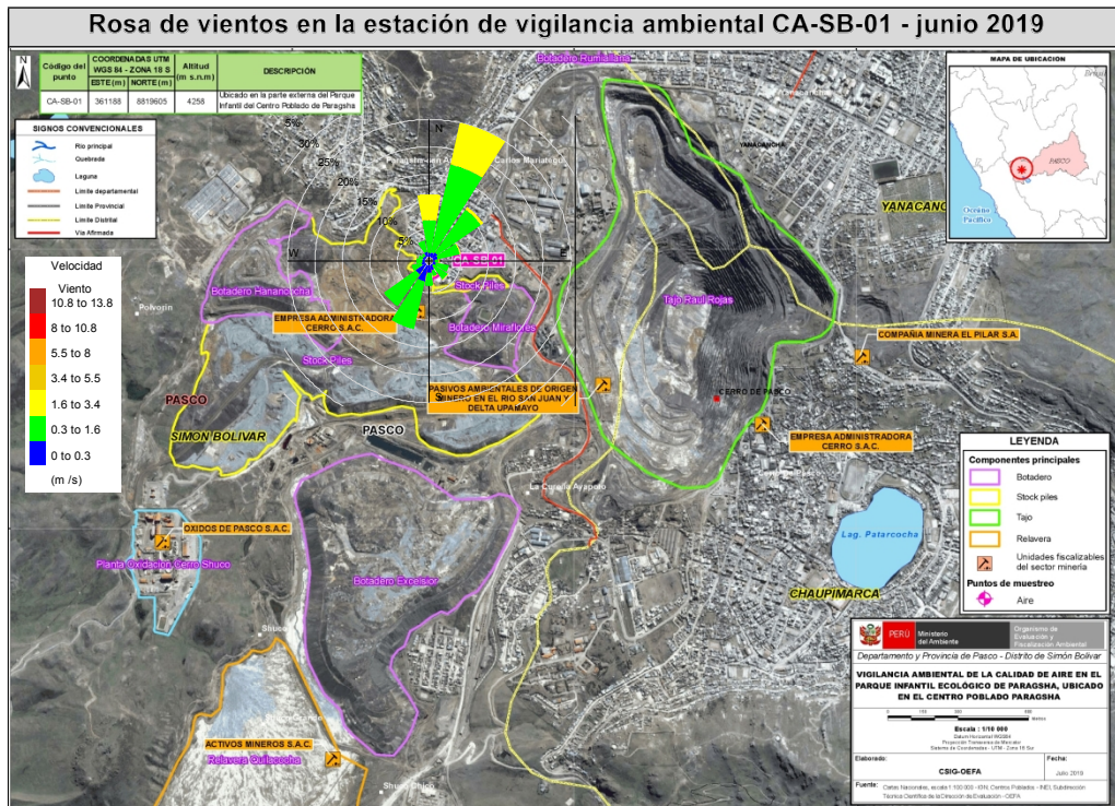
Figura 5.2. Ubicación de la estación de vigilancia ambiental CA-SB-01 y rosa de vientos en junio de 2019 Referencia: Imágenes satelitales extraídas de Google Earth.
