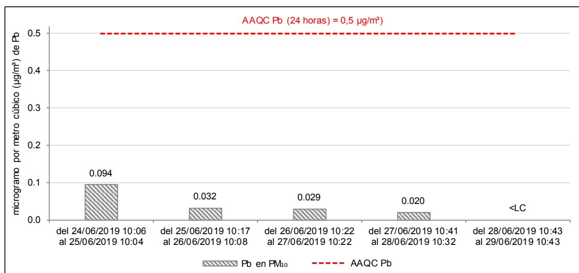
Figura 5.6. Concentraciones de plomo en material particulado con diámetro menor a 10 micras (Pb en PM 10 ) a 10°C y de 24 horas en junio 2019, de la estación de vigilancia ambiental de la calidad del aire CA-SB-01 comparadas de manera referencial con la normativa canadiense AAQC-2012.
