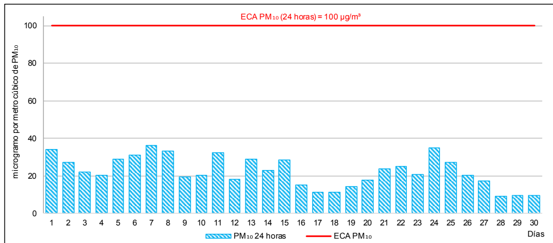
Figura 5.3. Concentraciones de 24 horas de PM 10 en la estación de vigilancia ambiental CA-SB-01, junio de 2019.
