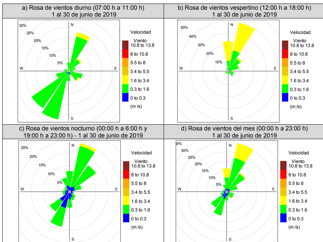
Figura 5.1. Representación gráfica de las rosas de vientos en la estación de vigilancia ambiental CA-SB-01, en junio de 2019 a) en horario diurno, b) en horario vespertino, c) en horario nocturno, d) en todas las horas del mes
