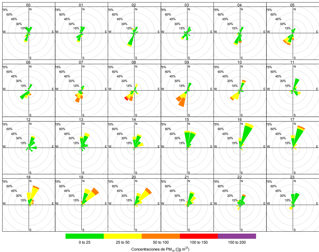
Figura 5.5. Rosas de concentración por horas de PM 10 en la estación de vigilancia CA-SB-01, desde las 00:00 horas hasta las 23:00 horas, en junio de 2019
