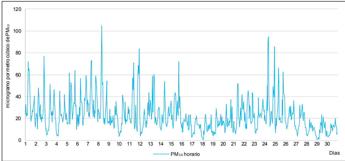
Figura 5.4. Concentraciones horarias de PM 10 en la estación de vigilancia ambiental CA-SB-01 en junio de 2019.
