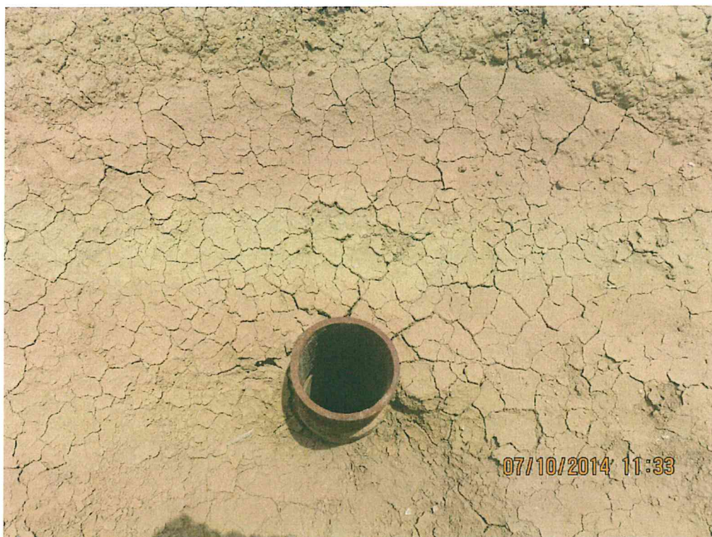
Fotografía N° 1. Vista pozo T1945, se observa el casing corroído y abierto al ambiente.
