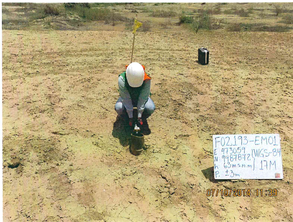
Fotografía N° 4. Vista de la medición de emisiones en el punto F02193-EM01, ubicado en boca de pozo T1945.
