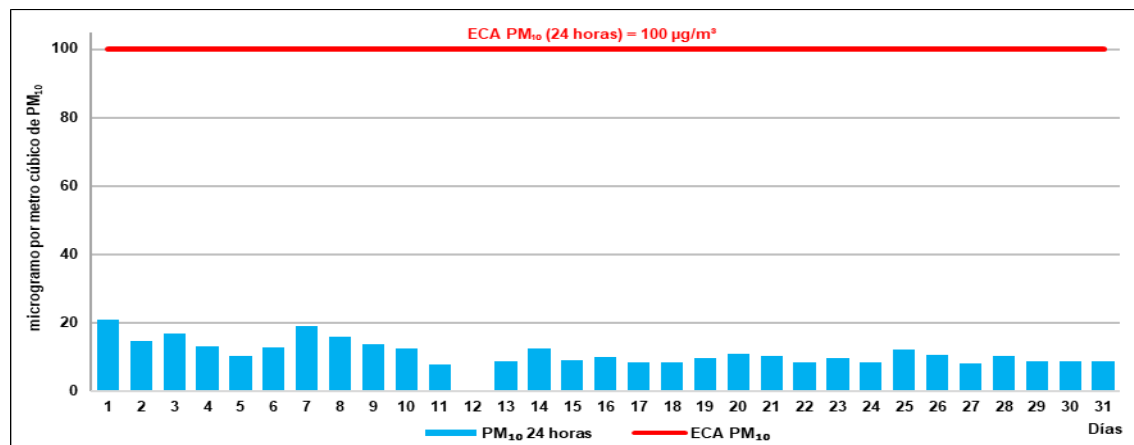
Figura 5.3. Concentraciones de 24 horas de PM 10 en la estación de vigilancia ambiental CA-SB-01, enero de 2019.
