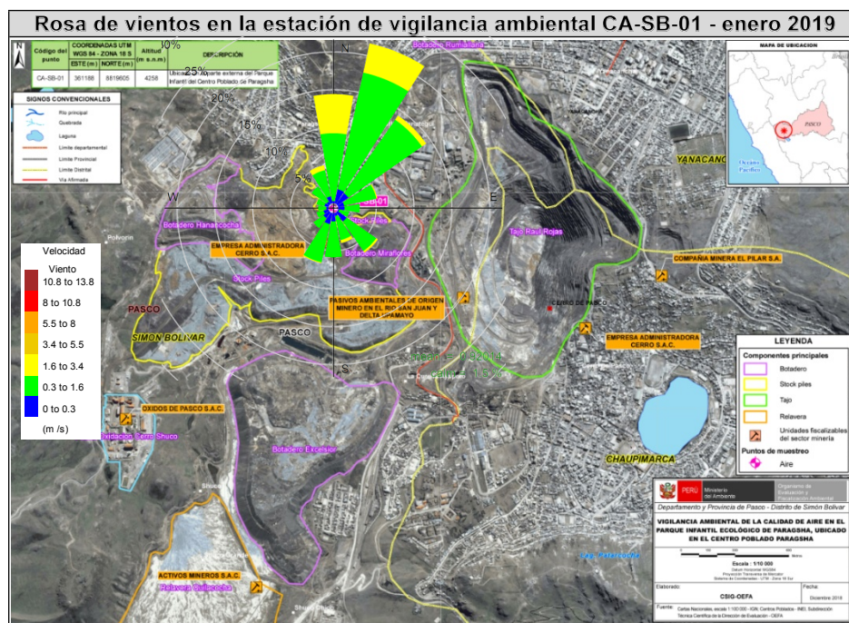
Figura 5.2. Ubicación de la estación de vigilancia ambiental CA-SB-01 y rosa de vientos de enero 2019.
