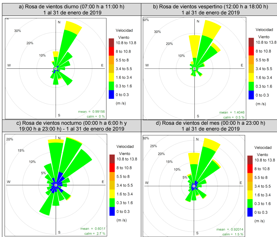
Figura 5.1. Representación gráfica de las rosas de vientos en la estación de vigilancia ambiental CA-SB-01, del 1 al 31 de enero a) en horario diurno, b) en horario vespertino, c) en horario nocturno, d) en todas las horas del mes.
