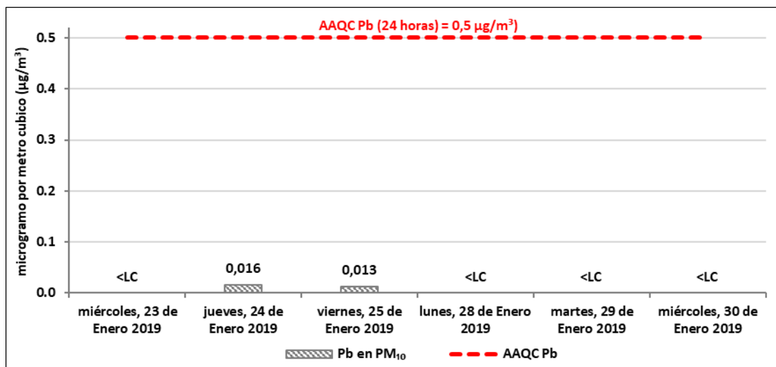
Figura 5.7. Concentraciones de plomo en material particulado con diámetro menor a 10 micras (Pb en \text{PM}_{10} ) a 10^\circ\text{C} y de 24 horas en la estación de vigilancia ambiental de la calidad del aire CA-SB-01 comparadas de manera referencial con la normativa canadiense AAQC-2012.
