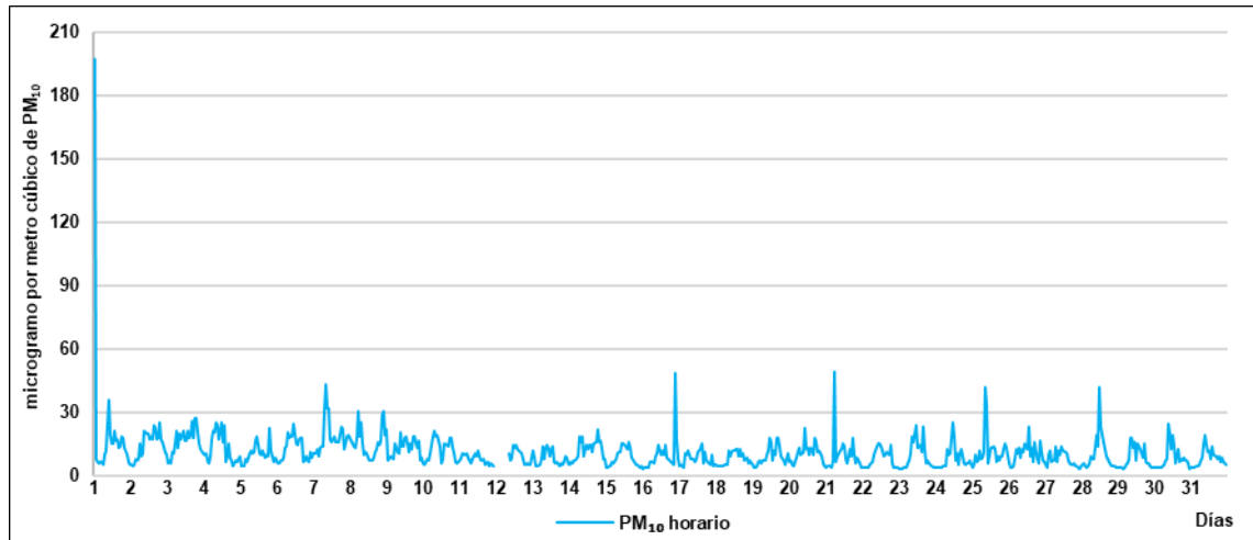
Figura 5.4. Concentraciones horarias de PM 10 en la estación de vigilancia ambiental CA-SB-01, enero de 2019.
