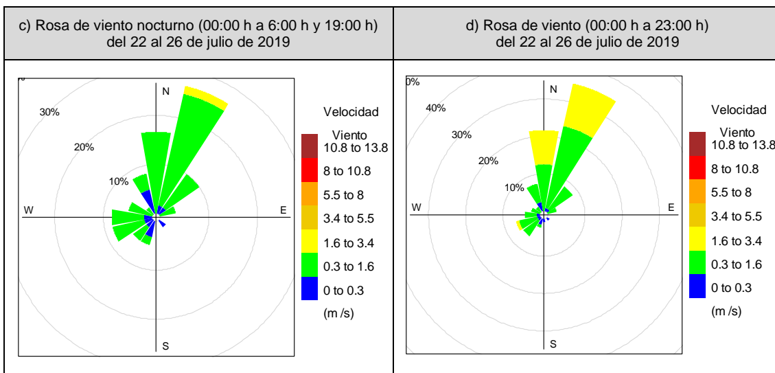
Figura 5.1. Rosas de vientos en el distrito de Simón Bolívar de 22 al 26 de julio de 2019 a) en horario diurno, b) en horario vespertino, c) en horario nocturno, d) en todas las horas.
