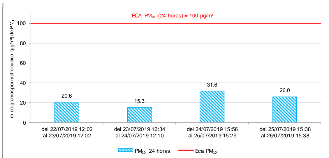
Figura 5.3. Concentraciones de 24 horas de PM 10 en la estación de vigilancia ambiental CA-SB-02, del 22 al 26 de julio de 2019.
