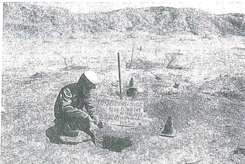
Fotografía N° 2. Toma de muestra de suelo en el punto F01498-SU02, aproximadamente a 3 m al Norte del Pozo NN3-VII y a una profundidad de 0,35 m a 0,45 m de la superficie del suelo.
