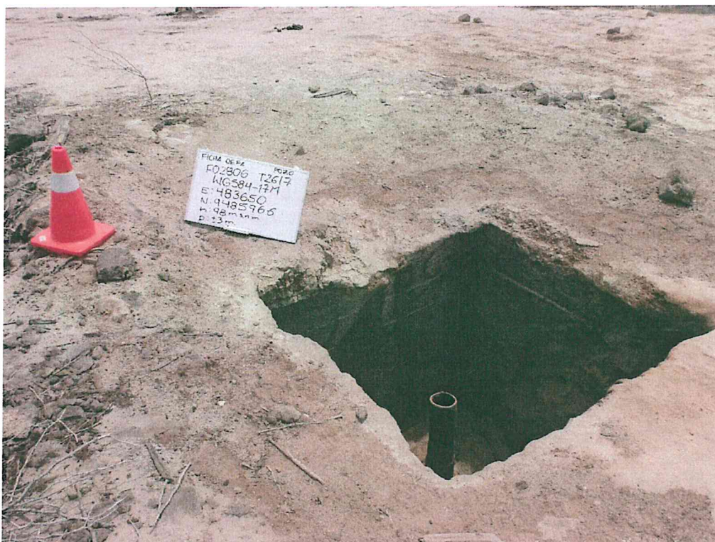
Fotografía N° 1. Identificación del pozo inactivo con código PERUPETRO T2617. Presenta casing descubierta en el interior de una excavación de sección rectangular.
