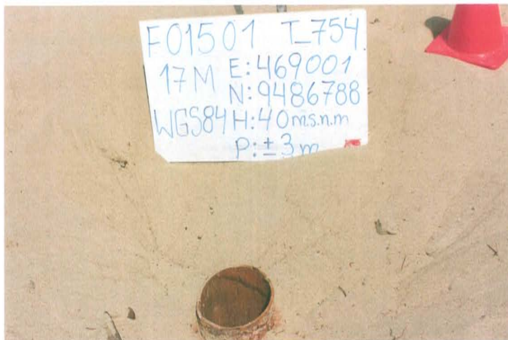
Fotografía N° 1. Pozo T_754, presenta casing corroído y abierto.
