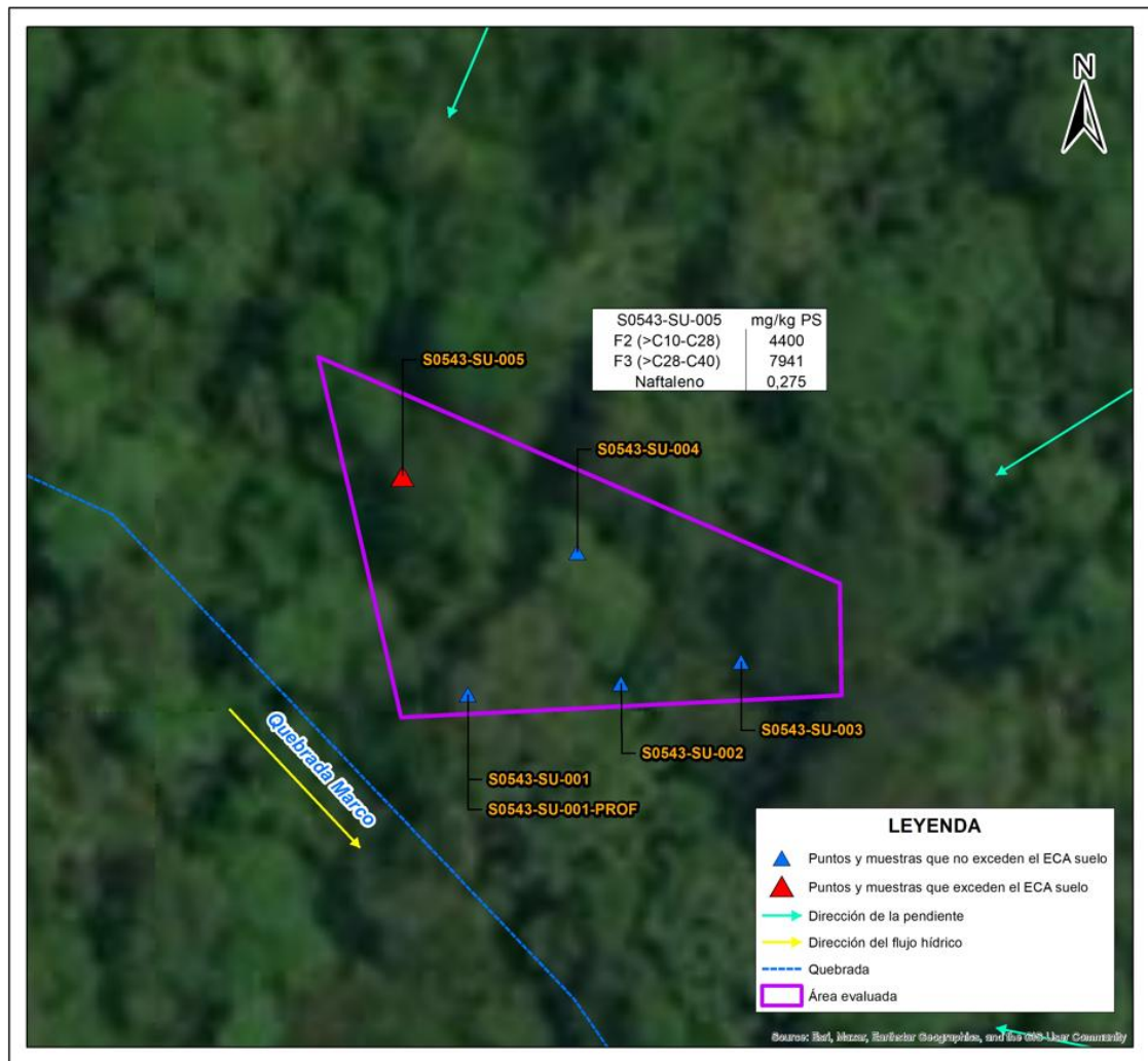
Figura 8.7. Muestras que superan los ECA suelo, uso agrícola en al menos un parámetro en el sitio S0543
