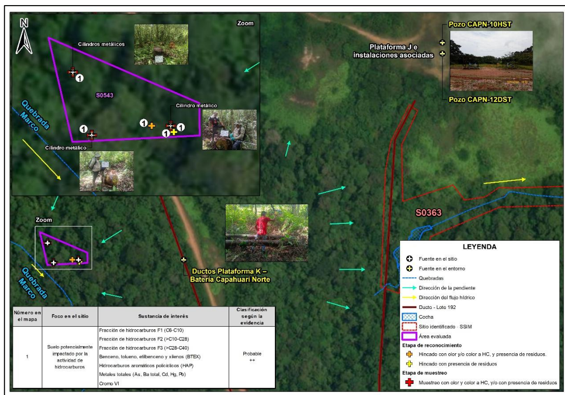
Figura 7.3. Ubicación de las posibles fuentes y focos de contaminación para el sitio S0543 HC: Hidrocarburos.
