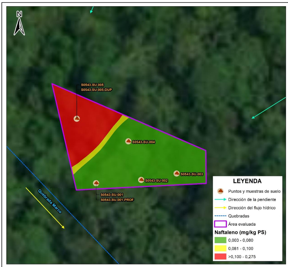
Figura 8.6. Distribución espacial horizontal de concentraciones de naftaleno en suelo del sitio S0543
