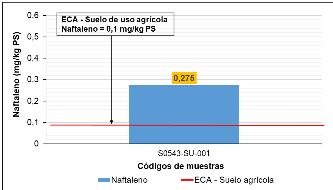
Figura 8.5. Resultados de naftaleno de las muestras de suelo en el sitio S0543
