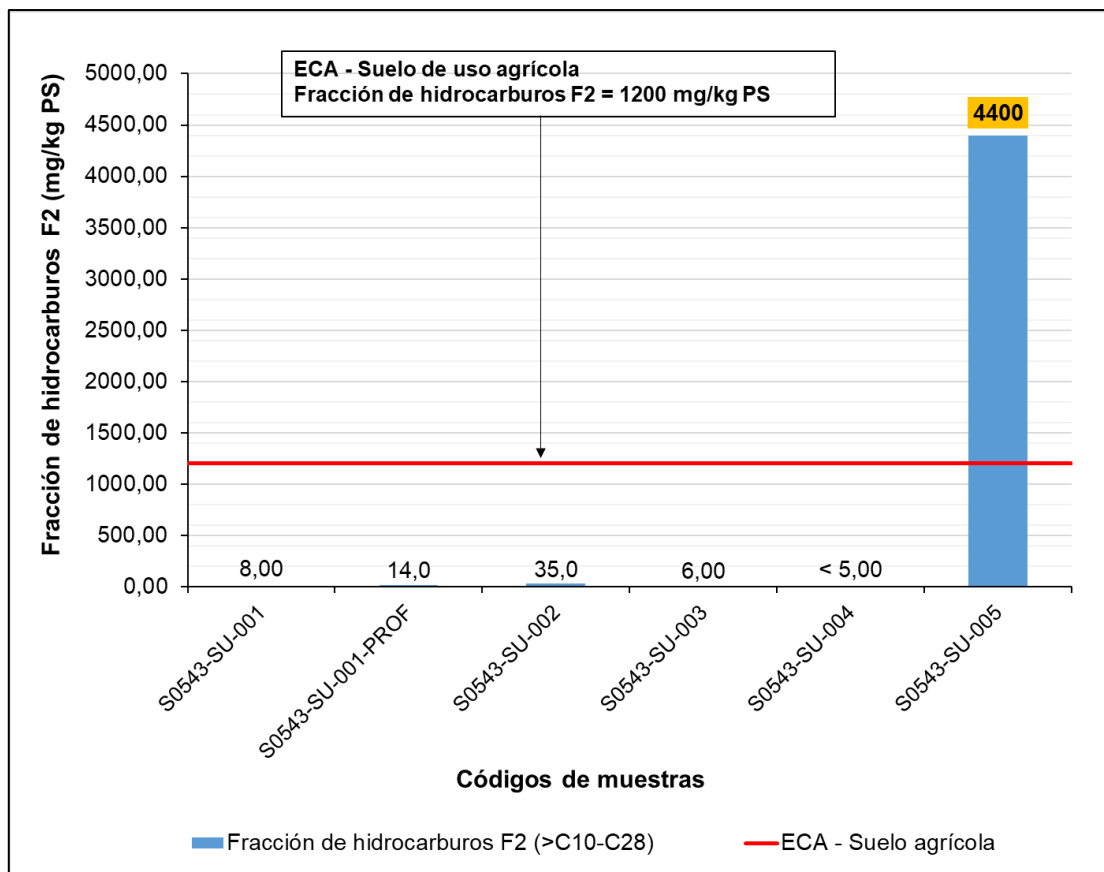
Figura 8.1. Resultados de fracción de hidrocarburos F2 de las muestras de suelo en el sitio S0543
