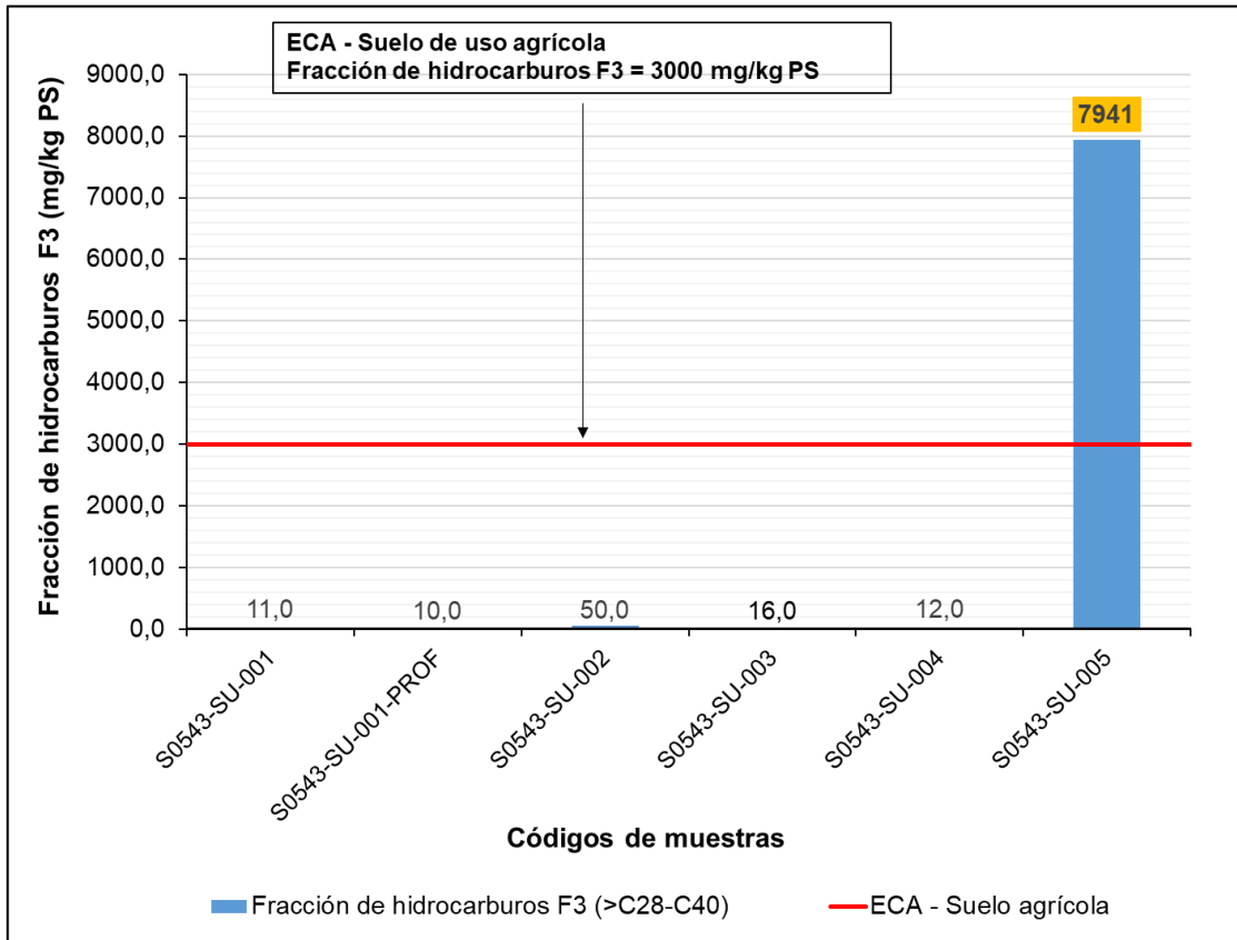
Figura 8.3. Resultados de fracción de hidrocarburos F3 de las muestras de suelo en el sitio S0543
