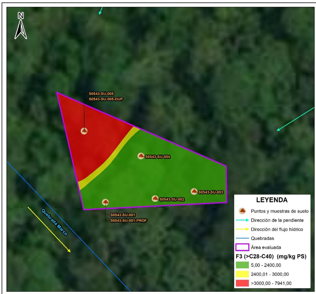
Figura 8.4. Distribución espacial horizontal de concentraciones de fracción de hidrocarburos F3 en suelo del sitio S0543
