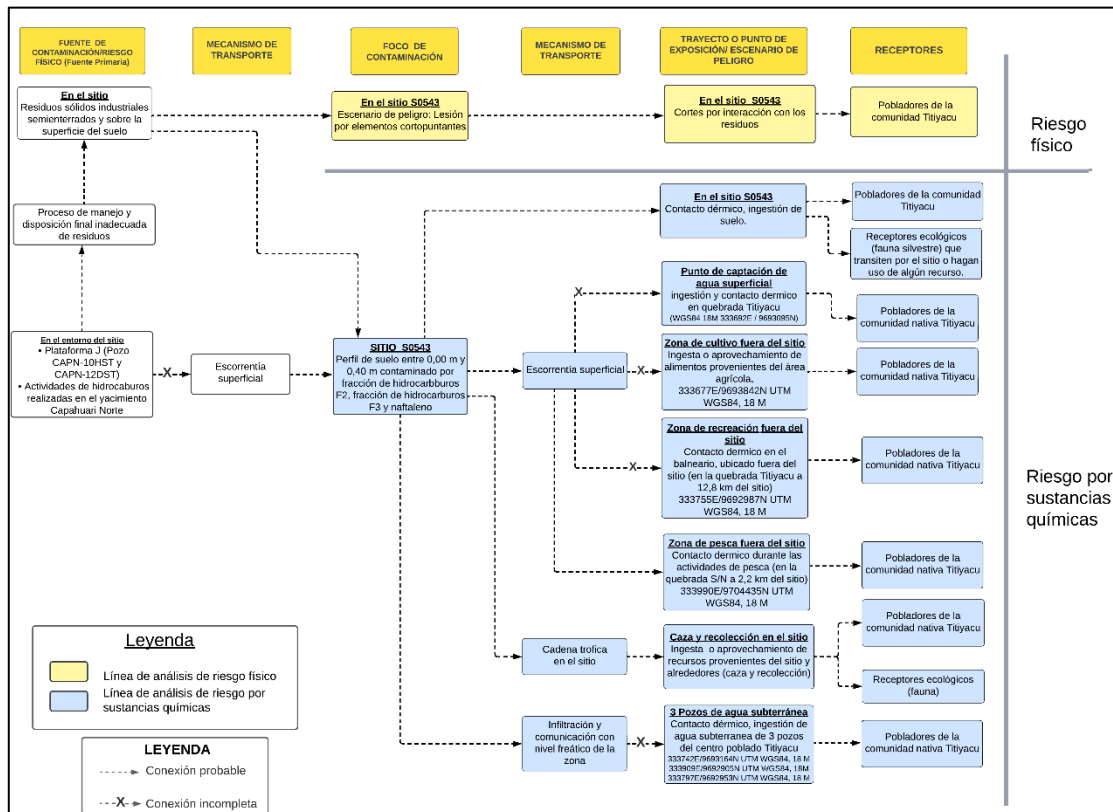
Figura 9.3. Esquema del modelo conceptual inicial para el sitio S0543
