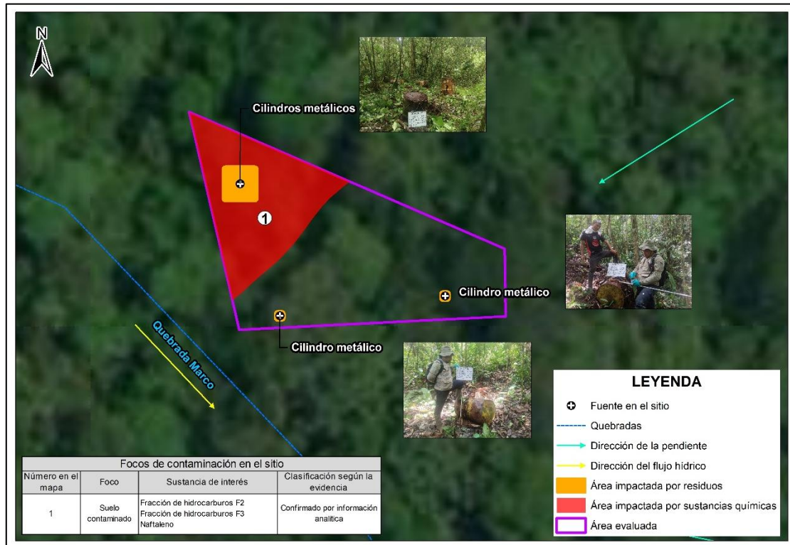
Figura 8.9. Fuentes y focos potenciales de contaminación para el sitio S0543
