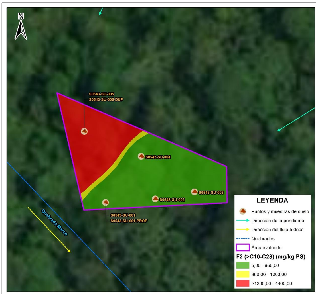
Figura 8.2. Distribución espacial horizontal de concentraciones de fracción de hidrocarburos F2 en suelo del sitio S0543
