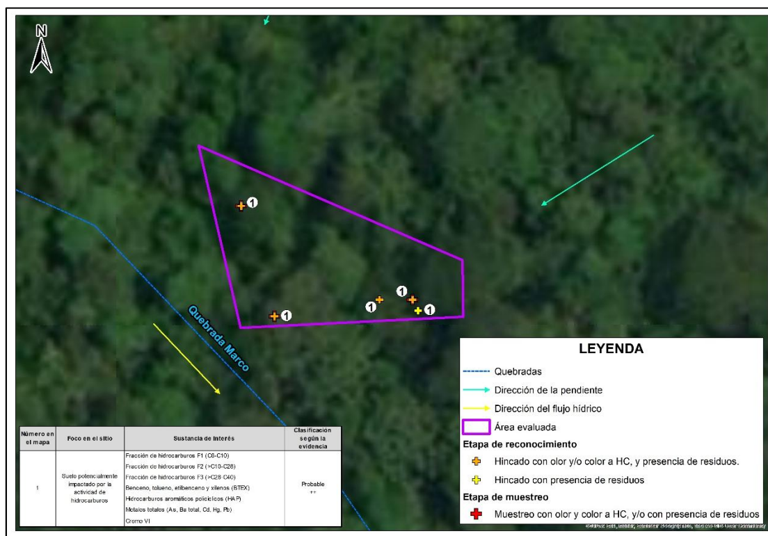
Figura 3.3. Posibles focos de contaminación en el sitio S0543 HC: Hidrocarburos.
