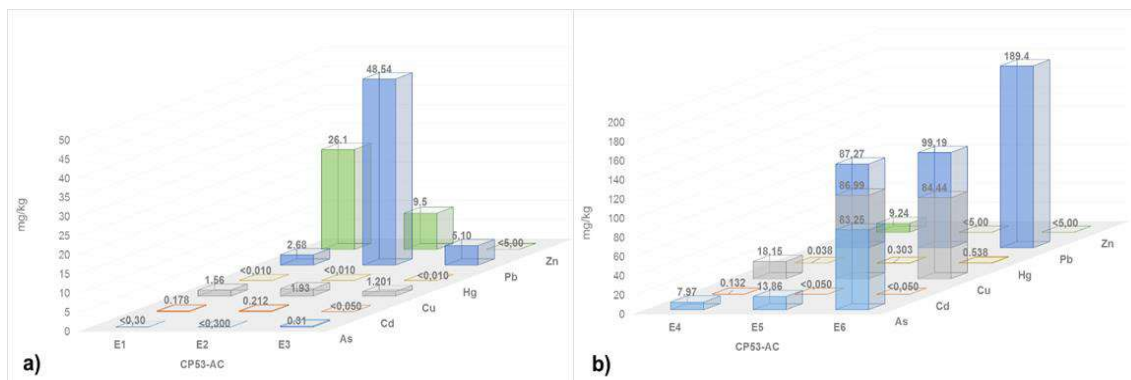
Figura 6.96. Extracción secuencial de metales por la metodología de Tessier, a) extracción 1, 2 y 3; y b) extracción 4, 5 y 6 en el punto CP53-AC
