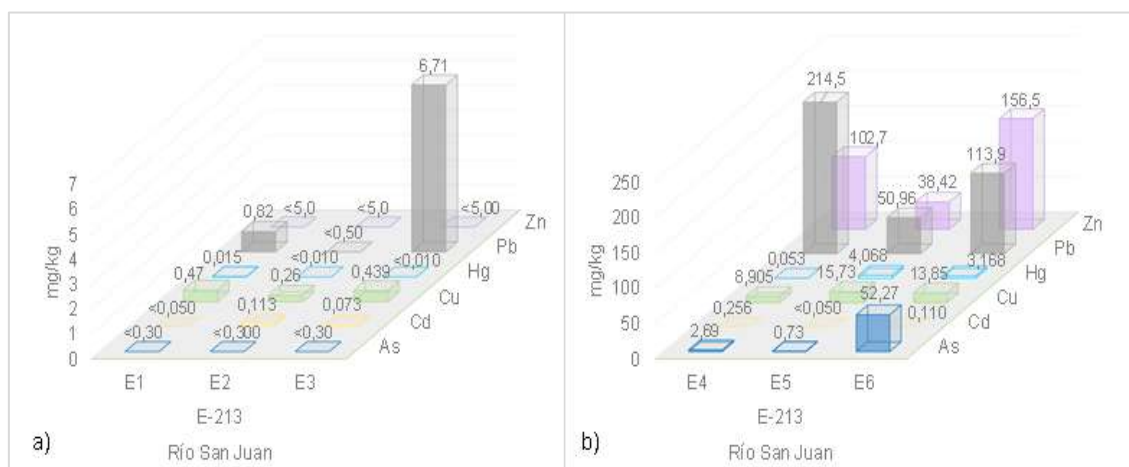
Figura 6.53. Resultados de metales (arsénico, cadmio, cobre, mercurio, plomo y zinc) por extracción Tessier del punto E-213 en a) extracciones E1, E2 y E3; y b) extracciones E4, E5 y E6 – agosto 2020
