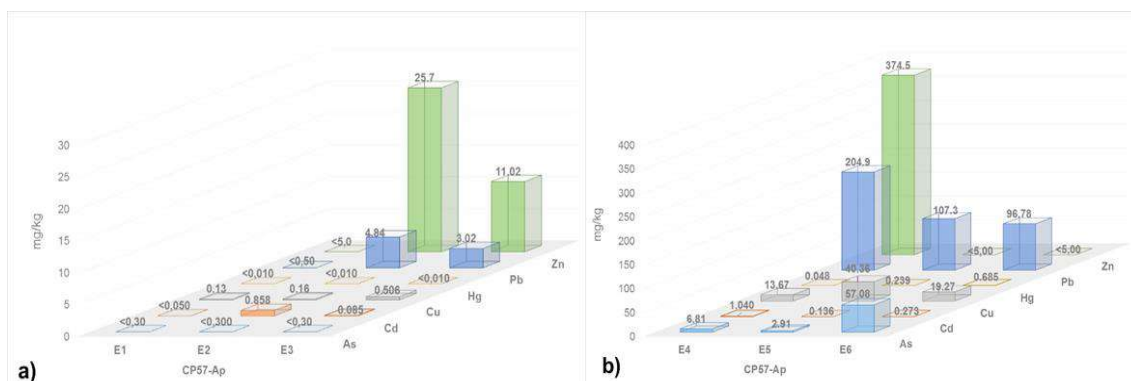
Figura 6.113. Extracción secuencial de metales por la metodología de Tessier, a) extracción 1, 2 y 3; y b) extracción 4, 5 y 6 en la muestra CP57-Ap
