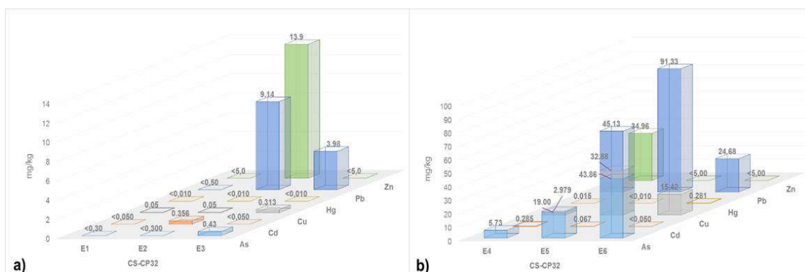
Figura 6.93. Extracción secuencial de metales por la metodología de Tessier, a) extracción 1, 2 y 3; y b) extracción 4, 5 y 6 en la muestra CS-CP32
