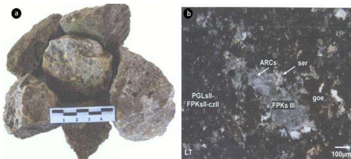
Figura 6.43. Análisis mineralógico por microscopía óptica de la muestra ROxP-1 a) vista macroscópica b) vista microscópica de matriz granular de plagioclasas II, feldespatos potásicos II y cuarzo II, (PGLsII-FPKsII-czII). Con cavidades que han sido rellenadas por feldespatos potásicos III (FPKs III) alterados por sericita (ser) y arcillas (ARCs), con impregnaciones de goethita (goe)
