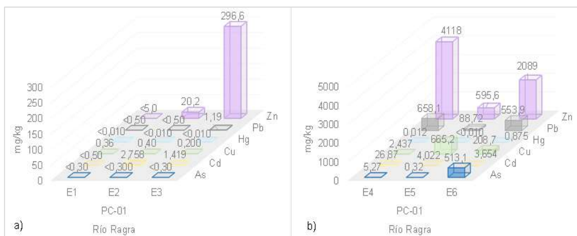
Figura 6.51. Resultados de metales (arsénico, cadmio, cobre, mercurio, plomo y zinc) por extracción Tessier del punto PC-01 en a) extracciones E1, E2 y E3; y b) extracciones E4, E5 y E6 – agostos 2020
