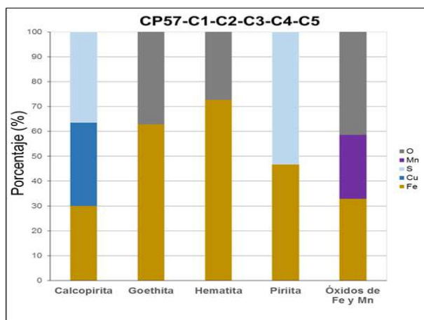
Figura 6.119. MEB de la muestra CP57 (horizontes ^C1, ^C2, ^C3, ^C4 y ^C5) extraída de la calicata CS-CP57-CAL en suelos del centro poblado de Paragsha ubicado próximo al botadero Miraflores
