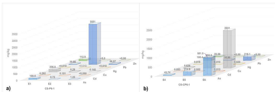
Figura 6.106. Extracción secuencial de metales por la metodología de Tessier, a) extracción 1, 2 y 3; y b) extracción 4, 5 y 6 en la muestra CS-CP6-1
