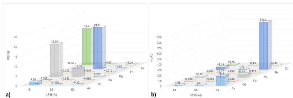
Figura 6.111. Extracción secuencial de metales por la metodología de Tessier, a) extracción 1, 2 y 3; y b) extracción 4, 5 y 6 en la muestra CP35-Ap
