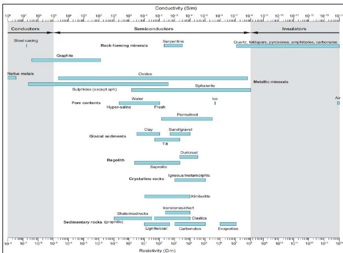
Figura 5.4. Resistividad y conductividad característica de distintos materiales
