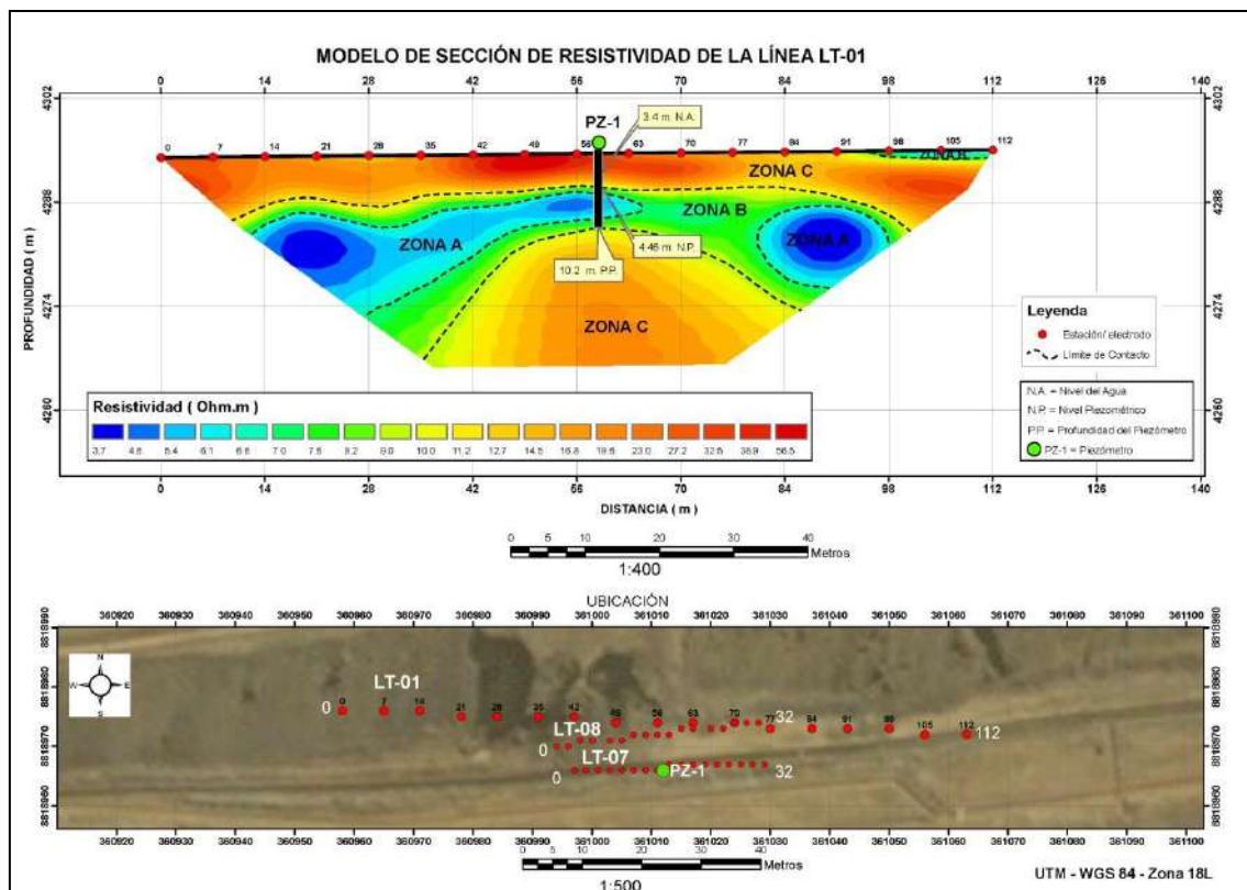
Figura 6.18. Línea de tomografía de resistividad eléctrica LT-01
