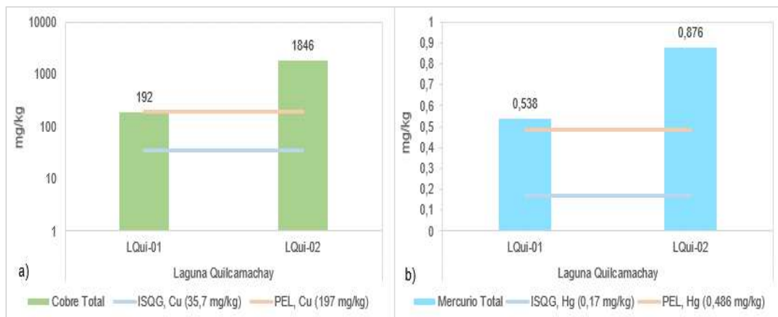
Figura 6.55. Resultados de metales en sedimento, comparados referencialmente con los valores ISQG y PEL de la CEQG-SQG en a) cobre y b) mercurio
