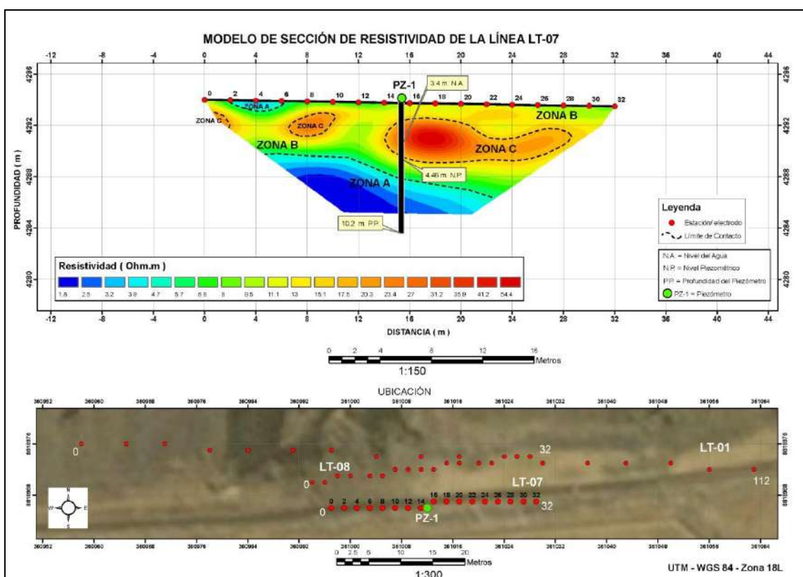
Figura 6.19. Línea de tomografía de resistividad eléctrica LT-07
