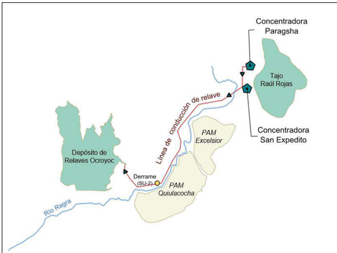
Figura 7.32. Esquema de ubicación de la línea de conducción de relaves
