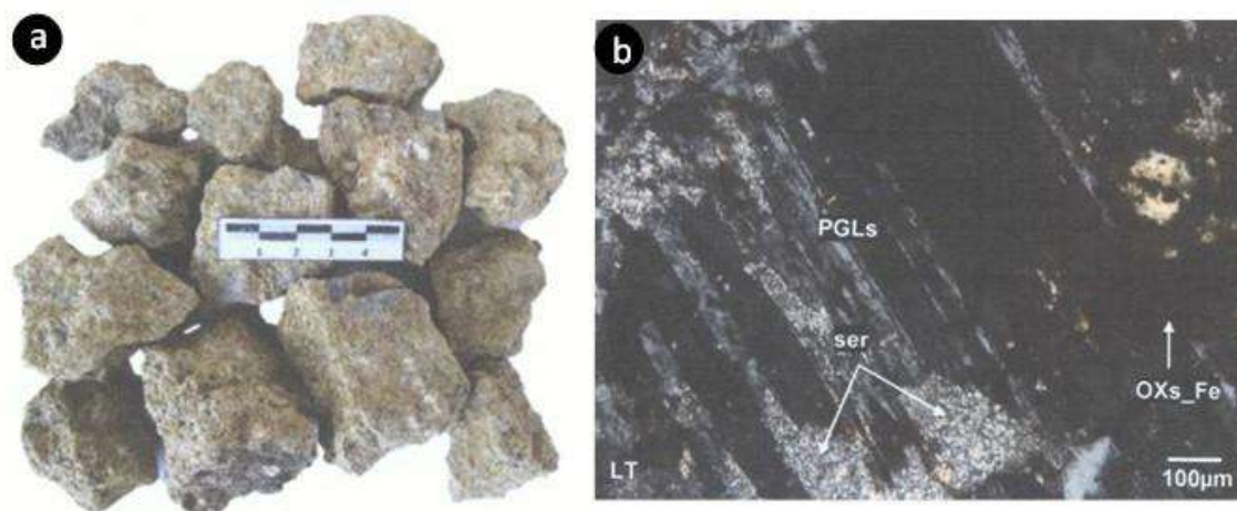
Figura 6.45. Análisis mineralógico por microscopía óptica de la muestra ROxP-3 a) vista macroscópica y b) vista microscópica de fragmentos de cristales de plagioclasas (PGLs) alterados por agregados de sericita (ser) y con impregnaciones de óxidos de hierro (OXs_Fe).
