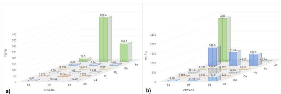
Figura 6.114. Extracción secuencial de metales por la metodología de Tessier, a) extracción 1, 2 y 3; y b) extracción 4, 5 y 6 en la muestra CP59-OA
