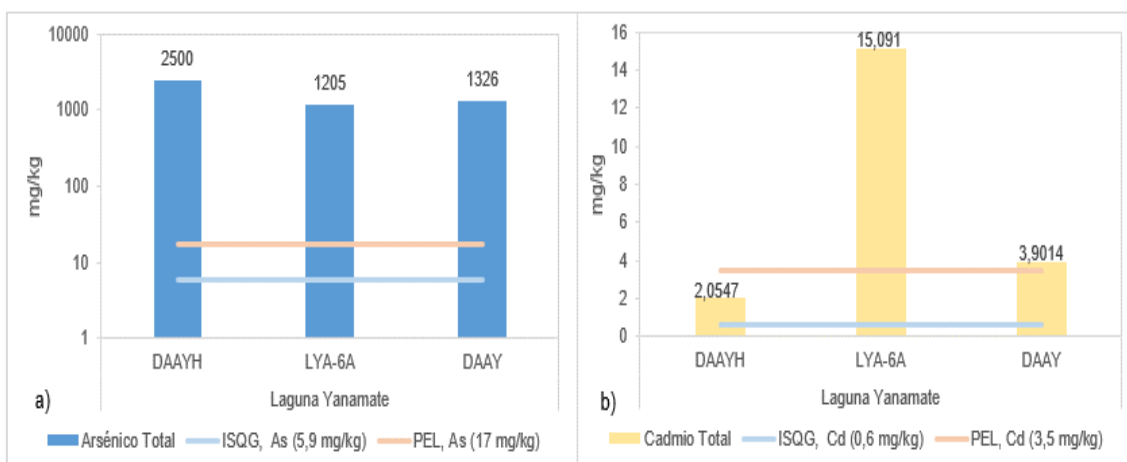
Figura 6.57. Resultados de metales en sedimento, comparados referencialmente con los valores ISQG y PEL de la CEQG-SQG en a) arsénico y b) cadmio
