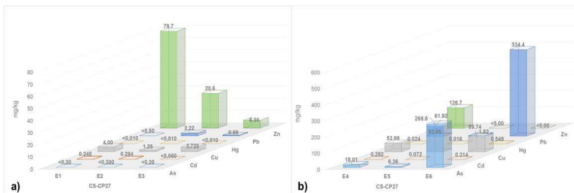
Figura 6.109. Extracción secuencial de metales por la metodología de Tessier, a) extracción 1, 2 y 3; y b) extracción 4, 5 y 6 en la muestra CS-CP27
