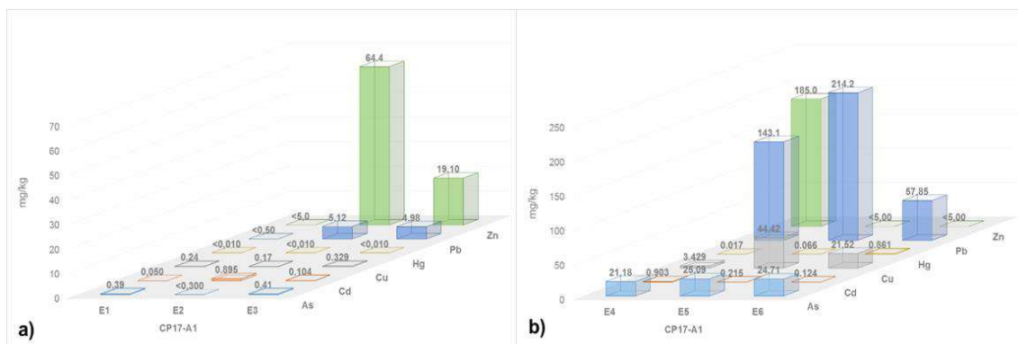
Figura 6.91. Extracción secuencial de metales por la metodología de Tessier, a) extracción 1, 2 y 3; y b) extracción 4, 5 y 6 en la muestra CP17-A1
