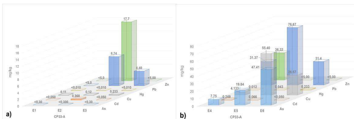
Figura 6.94. Extracción secuencial de metales por la metodología de Tessier, a) extracción 1, 2 y 3; y b) extracción 4, 5 y 6 en la muestra CP33-A
