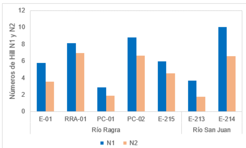
Figura 6.67. Números de Hill N1 y N2 de microalgas – agosto 2020
