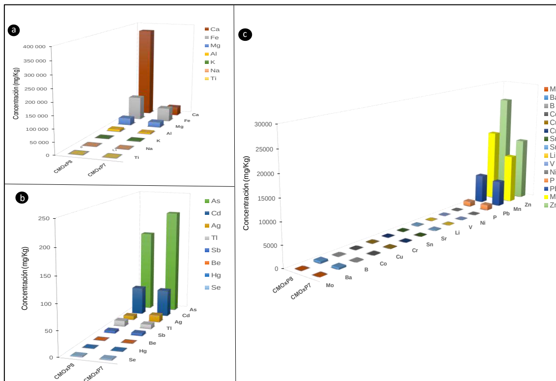
Figura 6.4. Metales totales de material botadero de desmonte Rumiallana en a) elemento mayores b) elemento menores y c) elementos traza
