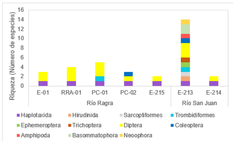
Figura 6.70. Composición y riqueza de macroinvertebrados bentónicos – agosto 2020
