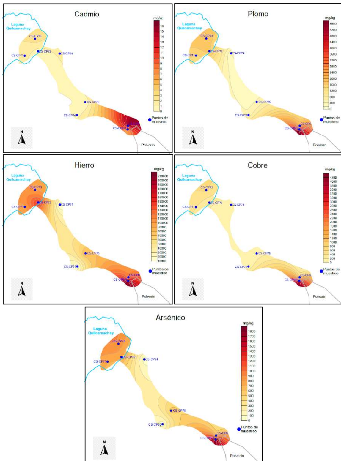
Figura 7.4. Distribución espacial de las concentraciones de a) cadmio, b) plomo, c) hierro, d) cobre, y e) arsénico
