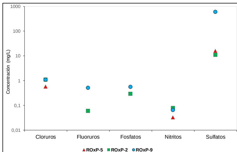
Figura 6.37. Shake Flask aniones en ROxP-5, ROxP2 y ROxP9
