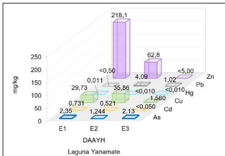
Figura 7.41. Metales biodisponibles en el depósito de aguas ácidas Yanamate
