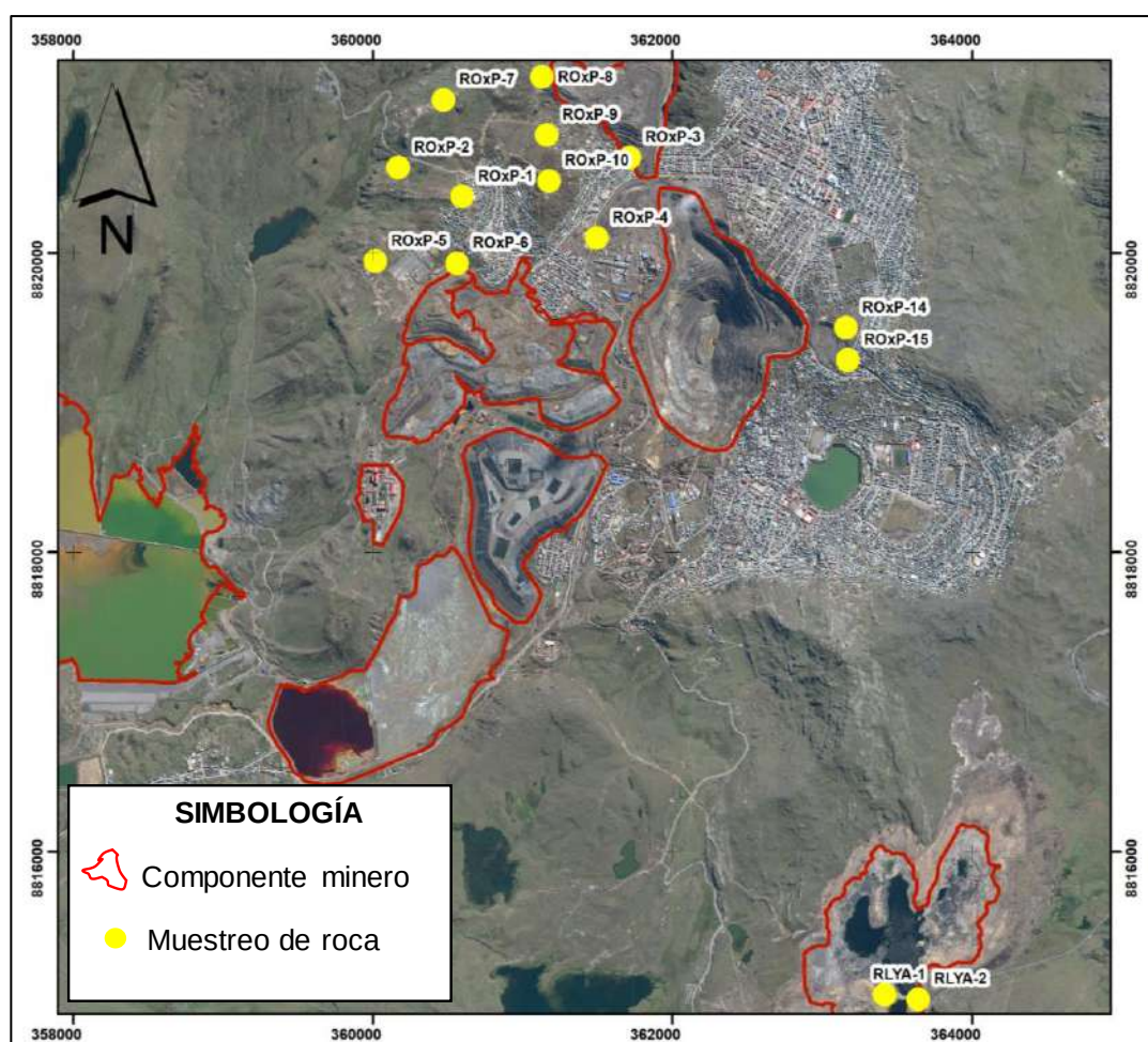
Figura 5.6. Distribución de puntos del muestreo de roca
