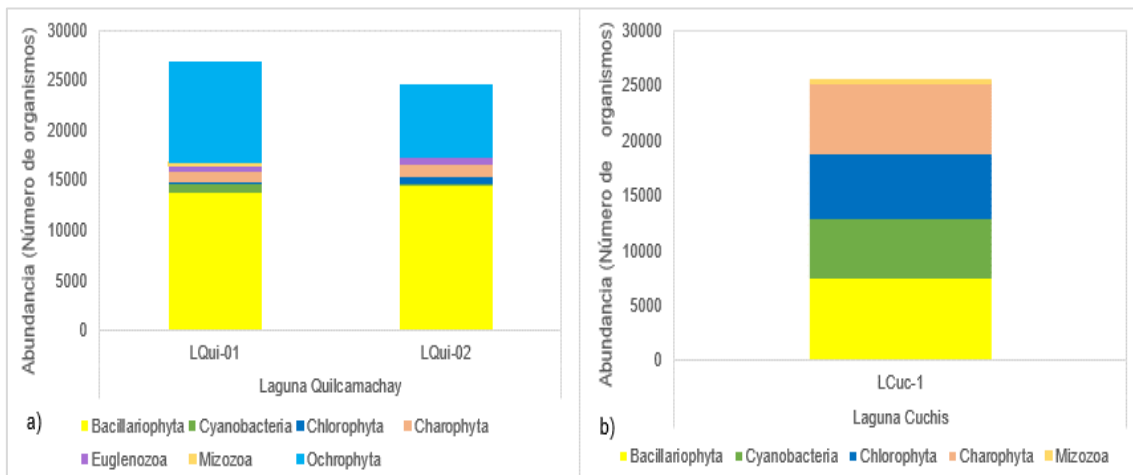
Figura 6.76. Abundancia de microalgas en a) laguna Quilcamachay y b) laguna Cuchis – agosto 2020
