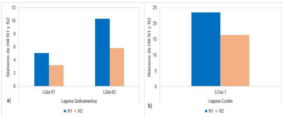
Figura 6.77. Números de Hill N1 y N2 de microalgas en a) laguna Quilcamachay y b) laguna Cuchis – agosto 2020
