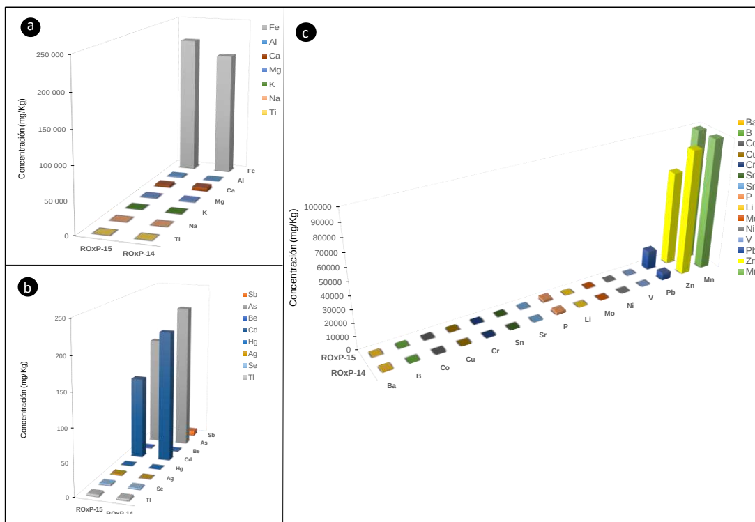
Figura 6.31. Metales totales en el ámbito de la Planta de Óxidos a) elementos mayores b) elementos menores c) elementos traza
