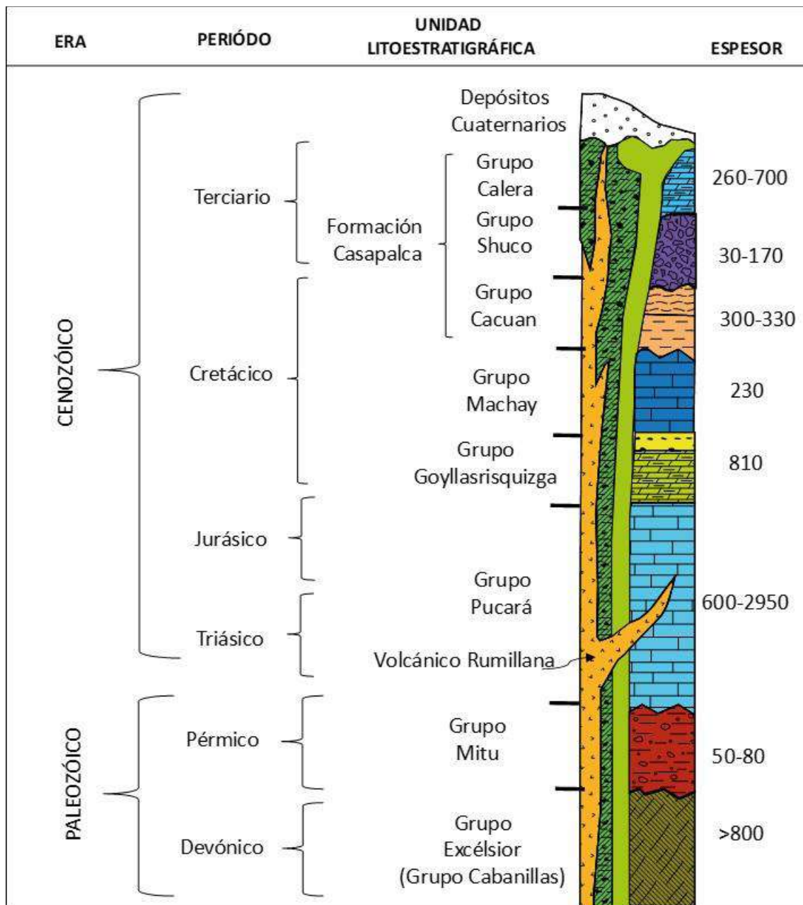
Figura 6.22. Columna estratigráfica que muestra las unidades litoestratigráficas en el ámbito de la UF Cerro de Pasco
