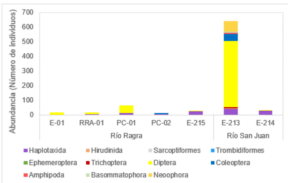
Figura 6.71. Abundancia de macroinvertebrados bentónicos – agosto 2020
