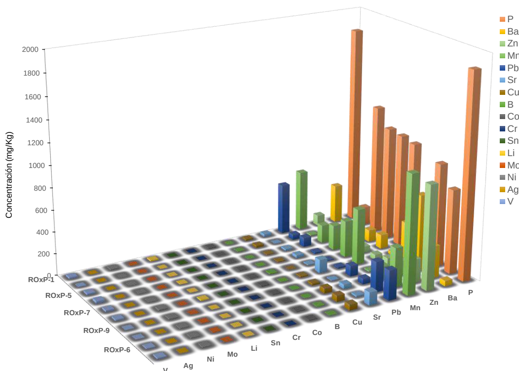
Figura 6.35. Metales totales en la UF Cerro de Pasco para los elementos traza
