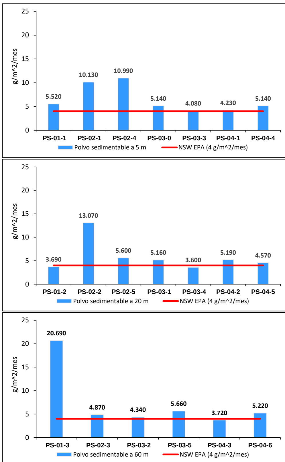
Figura 6.88. Concentración de polvo sedimentable g/m 2 /mes a) 5 m, b) 20 m y 60 m) de distancia componentes evaluados
