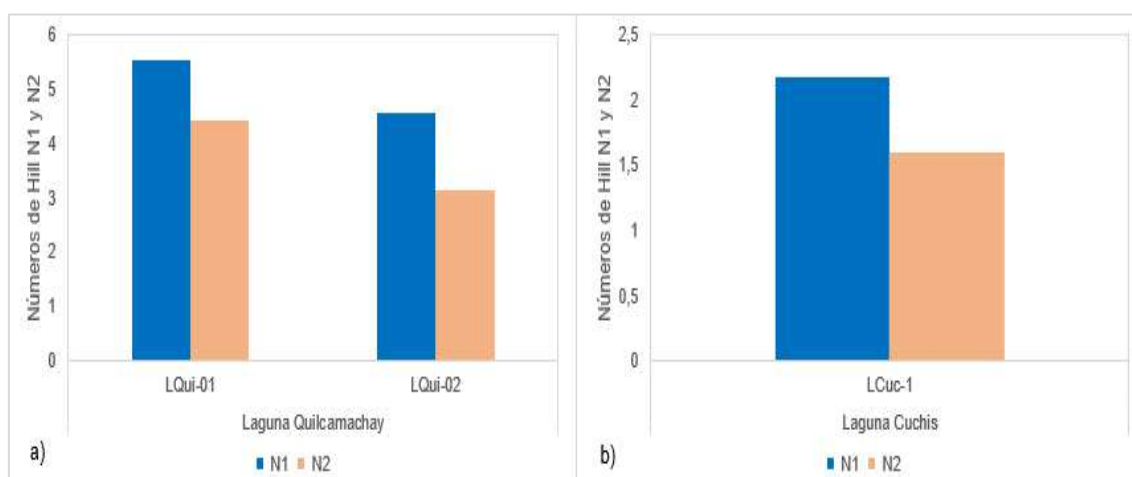
Figura 6.81. Números de Hill N1 y N2 de macroinvertebrados bentónicos en a) laguna Quilcamachay y b) laguna Cuchis – agosto 2020
