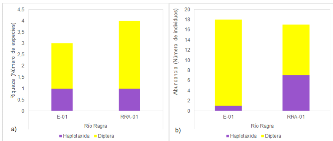
Figura 7.52. a) Composición y riqueza de macroinvertebrados bentónicos, y b) Abundancia de macroinvertebrados bentónicos – agosto 2020
