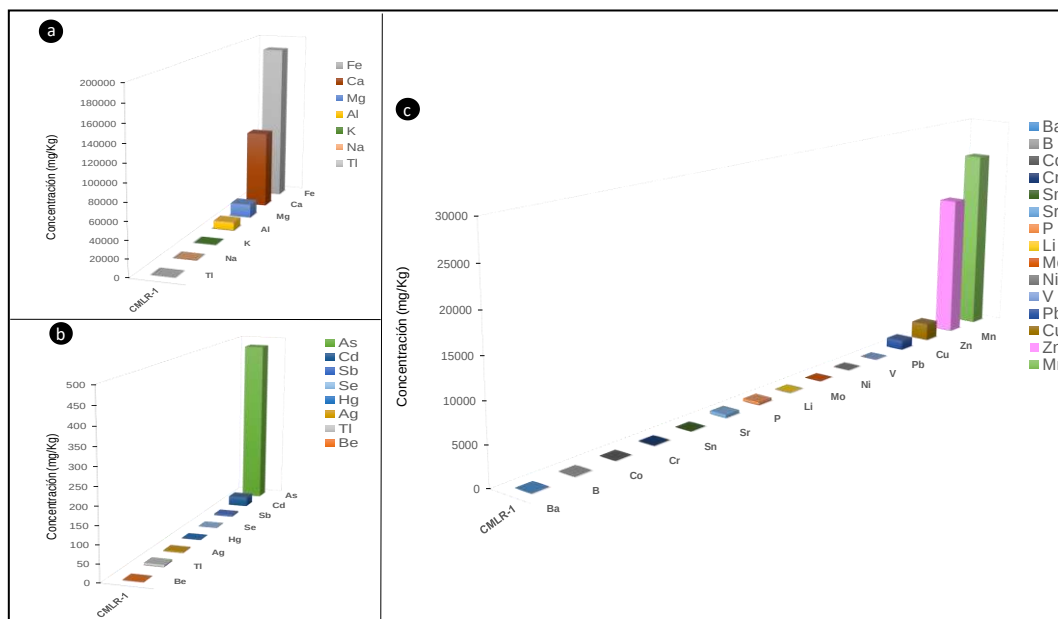
Figura 6.5. Metales totales en el canal de contención de la línea de relave San Expedito en a) elemento mayores b) elemento menores y c) elementos traza
