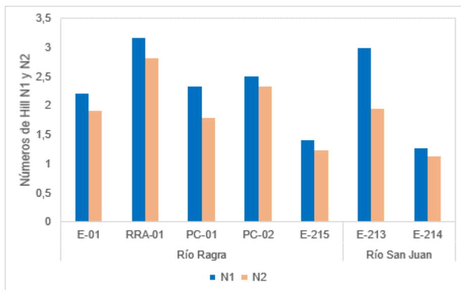
Figura 6.72. Números de Hill N1 y N2 de macroinvertebrados bentónicos – agosto 2020
