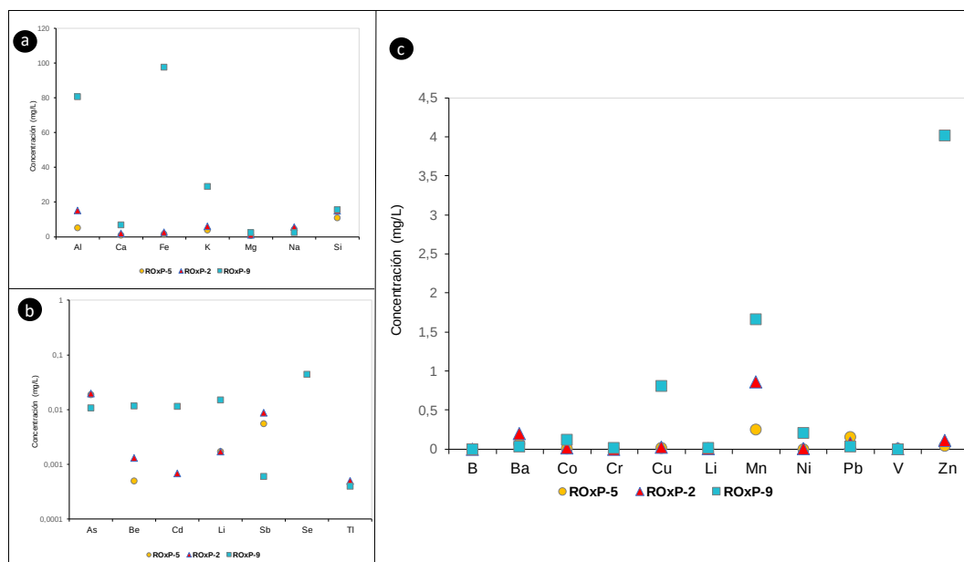
Figura 6.38. Shake Flask metales en las muestras ROxP-5, ROxP-2 y ROxP-9
