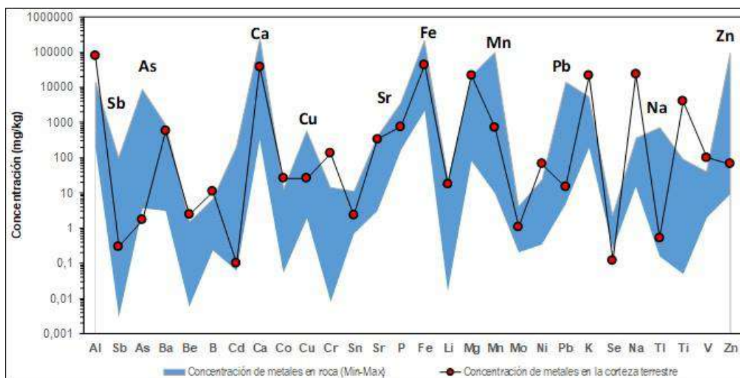
Figura 6.36. Comparación de las concentraciones de elementos mayores, menores y traza de las muestras ROxP-1 a ROxP-15 y RLYA-1 y RLYA-2 comparados con los valores de corteza continental propuesta por Wedepohl (1984)
