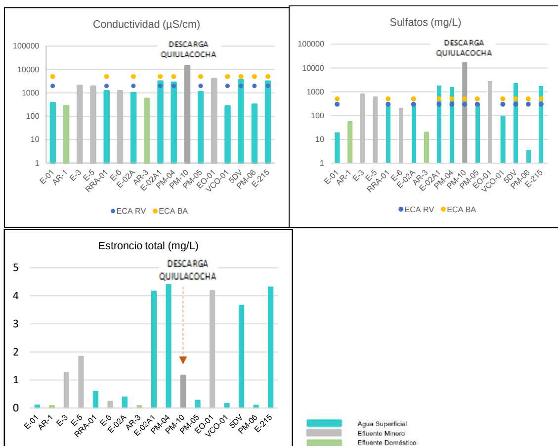
Figura 7.43. Concentración de los parámetros conductividad eléctrica, sulfatos, manganeso total y estroncio en las estaciones de agua superficial E-01, RRA-01, E-02A, E-02A-1, PM-04, PM-10, PM-05, EO-01, VCO-01, 5DV, PM-06 y E-215 y en los efluentes AR-1, E-3, E-5, E-6, AR-3, y EO-01.
