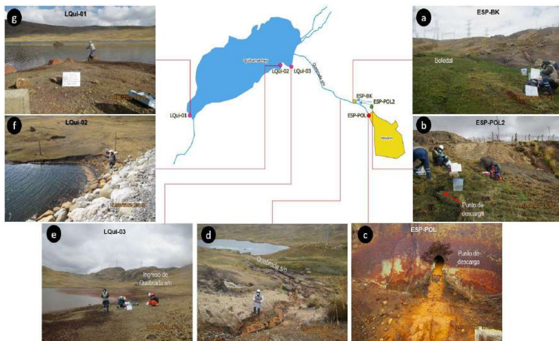
Figura 7.1. Secuencia de fotografías que muestran el flujo de agua desde su origen en el polvorín hasta la laguna Quicamachay, a) mezcla de aguas ESP-BK, b) punto de descarga ESP-POL2, c) punto de descarga ESP-POL, d) flujo de aguas acidas en quebrada s/n, e) f) y g) , puntos de muestreo en laguna Quicamachay.
