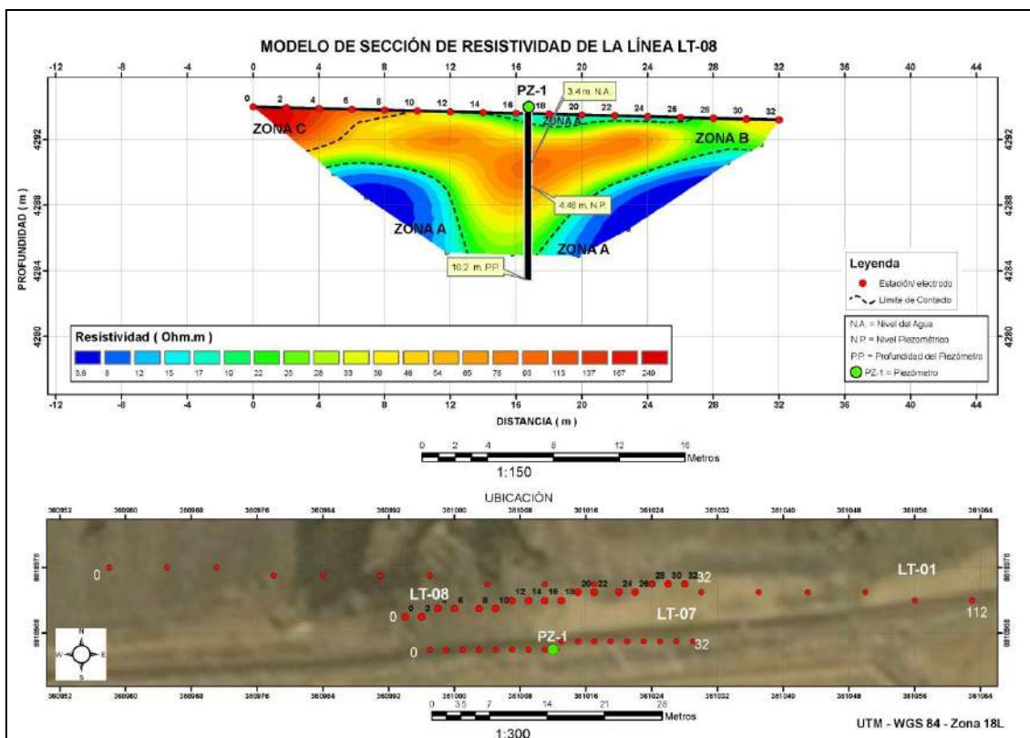
Figura 6.20. Línea de tomografía de resistividad eléctrica LT-08
