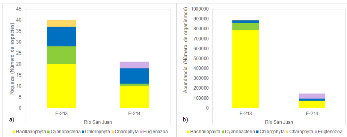
Figura 7.50. Composición de las microalgas en a) riqueza y b) abundancia
