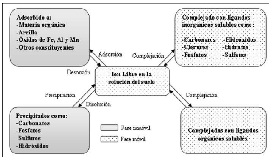
Figura 7.30. Procesos y componentes del suelo que controlan la movilidad de los metales pesados
