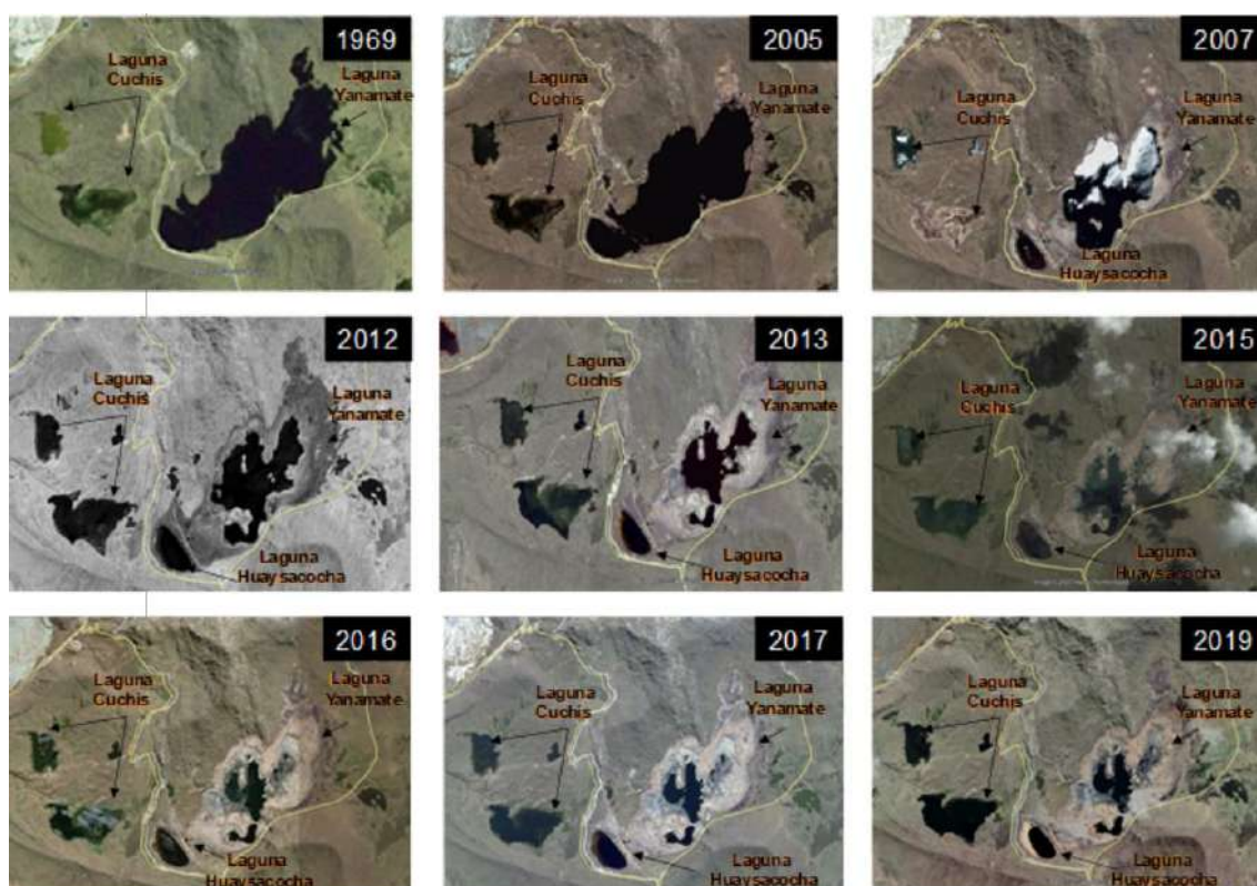
Figura 7.37. Análisis multitemporal de los años 1969, 2005, 2007, 2012, 2013, 2015, 2016, 2017 y 2019 en el ámbito de influencia del depósito de aguas ácidas Yanamate y Huaysacocha, y lagunas Cuchis
