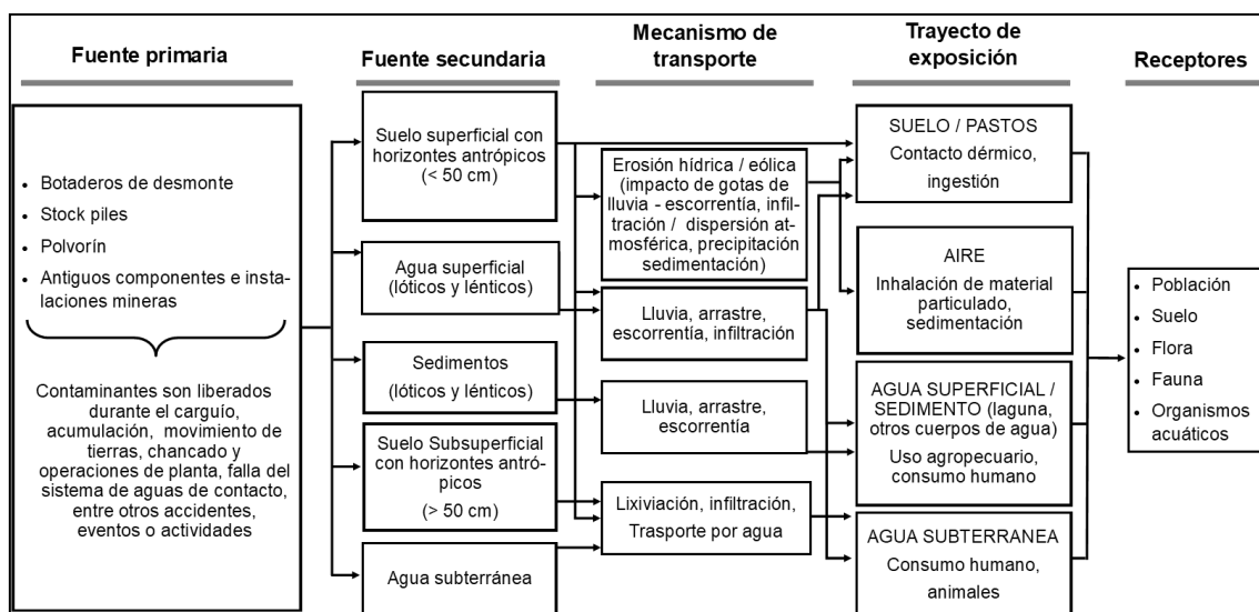
Figura 5.13. Modelo conceptual inicial propuesto para la presente evaluación del suelo
