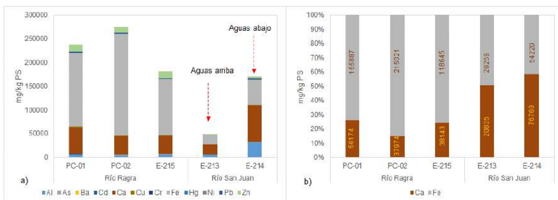
Figura 7.46. a) Comparación de las concentraciones de metales en los sedimentos de los ríos San Juan y Ragra y b) Predominancia de hierro y calcio (%)
