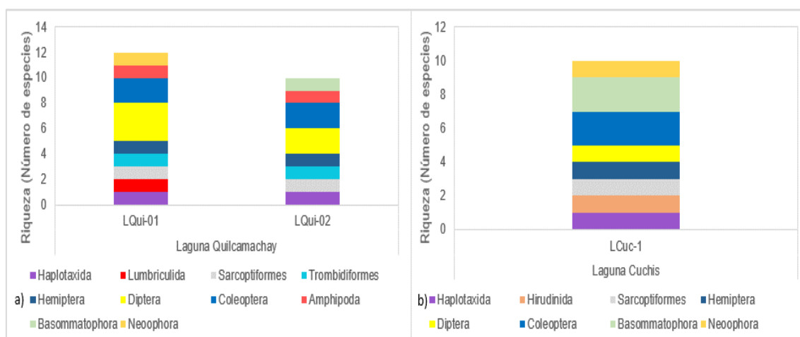
Figura 6.79. Composición y riqueza de macroinvertebrados bentónicos en a) laguna Quilcamachay y b) laguna Cuchis
