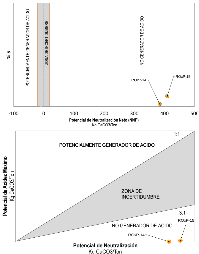
Figura 6.41. ABA en las muestras ROxP-14 y ROxP-15, según el primer y segundo criterio de evaluación
