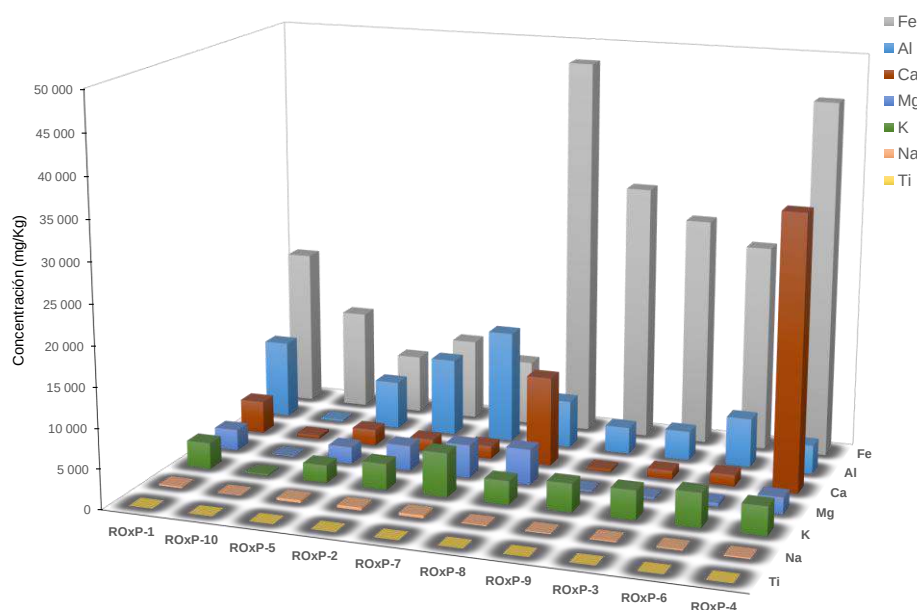
Figura 6.33. Metales totales en la UF Cerro de Pasco para los elementos mayores
