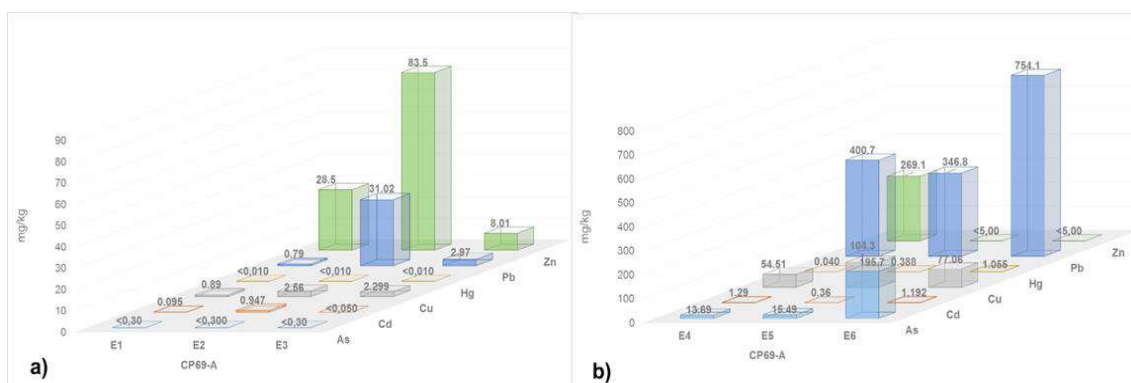
Figura 6.116. Extracción secuencial de metales por la metodología de Tessier, a) extracción 1, 2 y 3; y b) extracción 4, 5 y 6 en la muestra CP69-A
