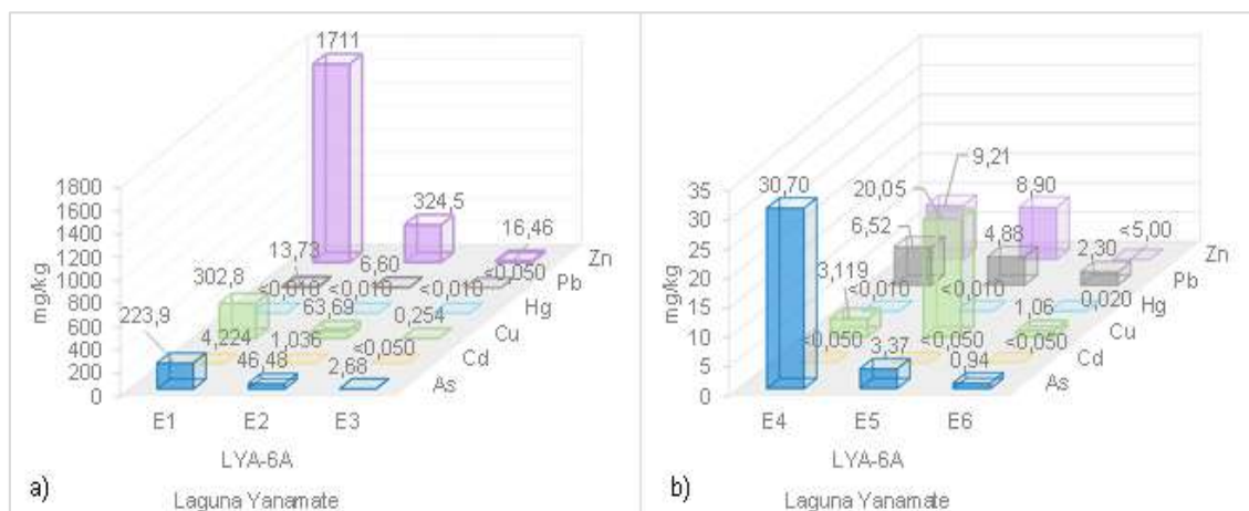
Figura 6.62. Resultados de metales (arsénico, cadmio, cobre, mercurio, plomo y zinc) por extracción Tessier del punto LYA-6A en a) extracciones E1, E2 y E3; y b) extracciones E4, E5 y E6 – agosto 2020
