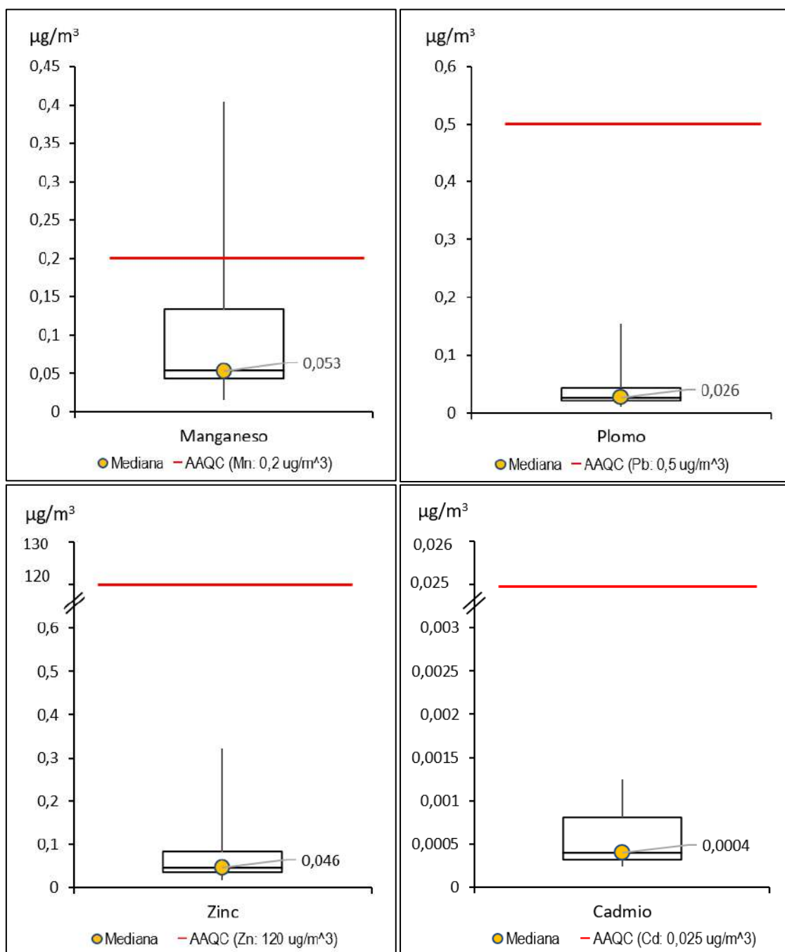
Figura 6.86. Concentración de metales en \text{PM}_{10} en el punto de monitoreo CA-SB-01, comparada referencialmente con la norma AAQC; evaluados del 06/08/2020 al 16/08/2020
