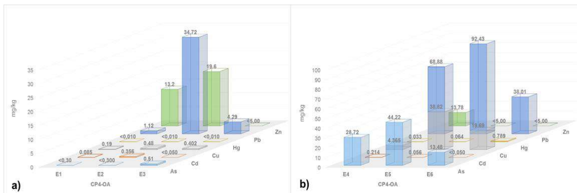
Figura 6.90. Extracción secuencial de metales por la metodología de Tessier, a) extracción 1, 2 y 3; y b) extracción 4, 5 y 6 en la muestra CP4-OA
