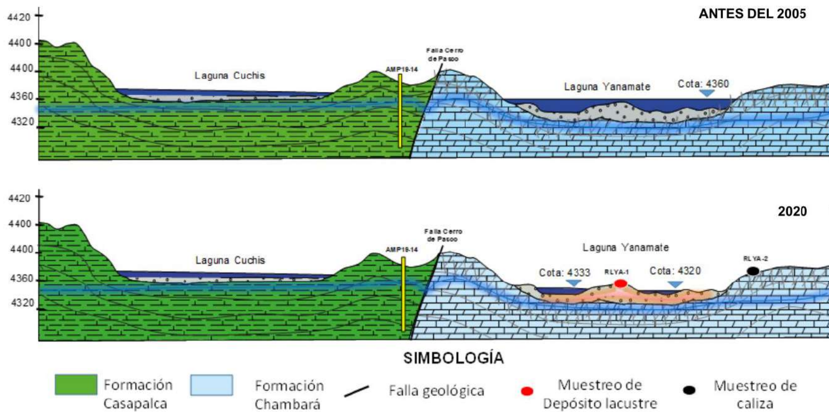
Figura 7.38. Perfil esquemático que muestra la litología del depósito de aguas ácidas Yanamate en el 2005 (cota 4360) y al 2020 (cota 4333 y 4320) mostrando los relictos de sedimentos lacustres alterados
