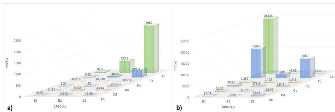
Figura 6.115. Extracción secuencial de metales por la metodología de Tessier, a) extracción 1, 2 y 3; y b) extracción 4, 5 y 6 en la muestra CP60-Ap
