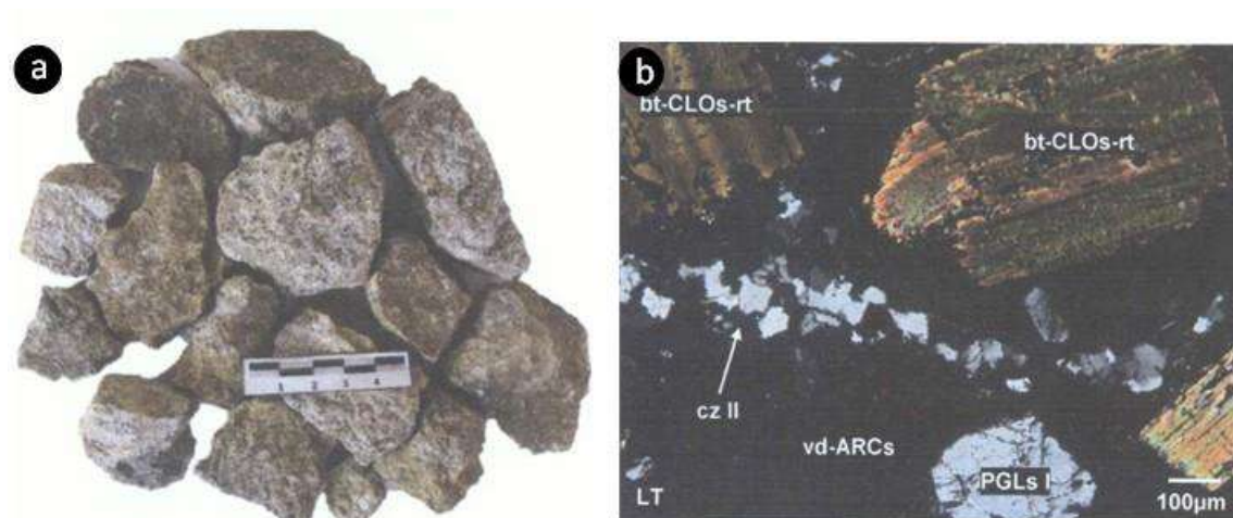
Figura 6.44. Análisis mineralógico por microscopía óptica de la muestra ROxP-2 a) vista macroscópica y b) vista microscópica de fenocristales de plagioclasas I (PGLs I) y de biotita alterados por cloritas y rutilo (btCLOs-rt). En una matriz de vidrio alterado por arcillas (vd-ARGs). Además, se aprecian finas venillas cortas rellenas por agregados de cristales de cuarzo II
