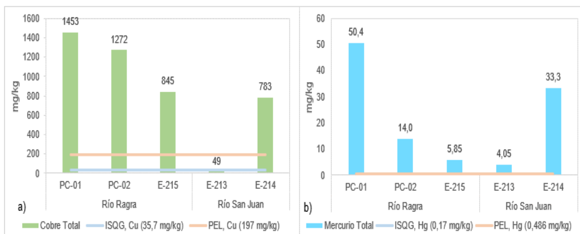
Figura 6.49. Resultados de metales en sedimento, comparados referencialmente con los valores ISQG y PEL de la CEQG-SQG en a) cobre y b) mercurio – agosto 2020
