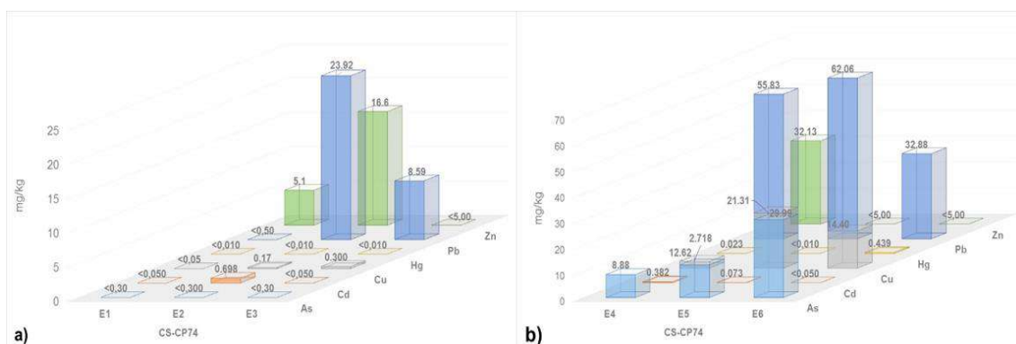
Figura 6.97. Extracción secuencial de metales por la metodología de Tessier, a) extracción 1, 2 y 3; y b) extracción 4, 5 y 6 en el punto CS-CP74
