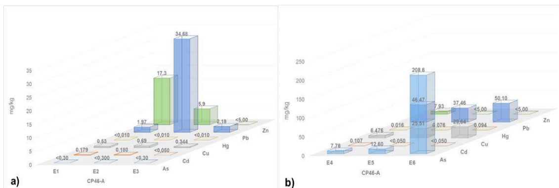
Figura 6.95. Extracción secuencial de metales por la metodología de Tessier, a) extracción 1, 2 y 3; y b) extracción 4, 5 y 6 en la muestra CP46-A
