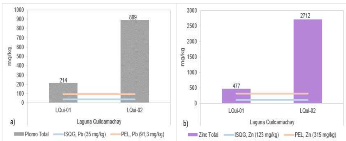
Figura 6.56. Resultados de metales en sedimento, comparados referencialmente con los valores ISQG y PEL de la CEQG-SQG en a) plomo y b) zinc
