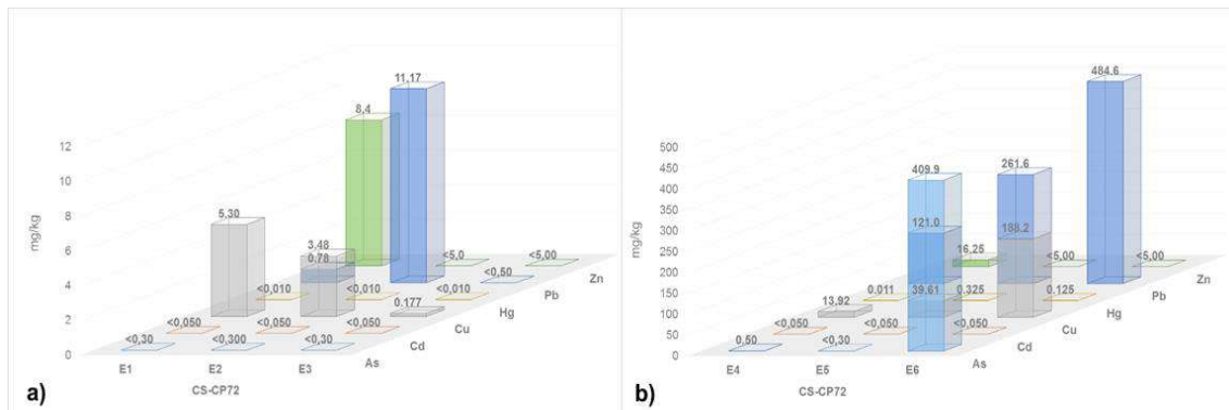
Figura 6.107. Extracción secuencial de metales por la metodología de Tessier, a) extracción 1, 2 y 3; y b) extracción 4, 5 y 6 en la muestra CS-CP72
