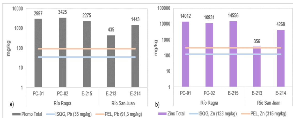
Figura 6.50. Resultados de metales en sedimento, comparados referencialmente con los valores ISQG y PEL de la CEQG-SQG en a) plomo y b) zinc – agosto 2020
