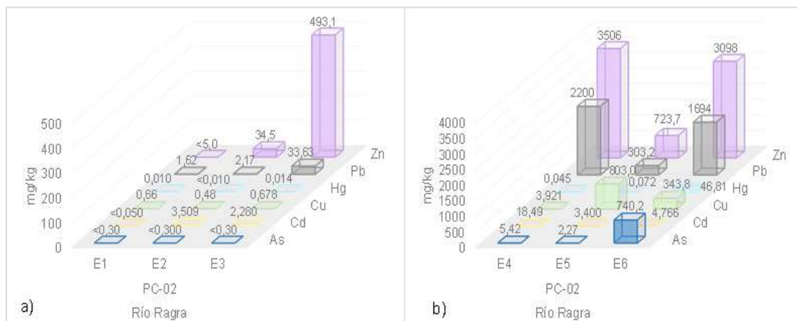
Figura 6.52. Resultados de metales (arsénico, cadmio, cobre, mercurio, plomo y zinc) por extracción Tessier del punto PC-02 en a) extracciones E1, E2 y E3; y b) extracciones E4, E5 y E6 – agosto 2020
