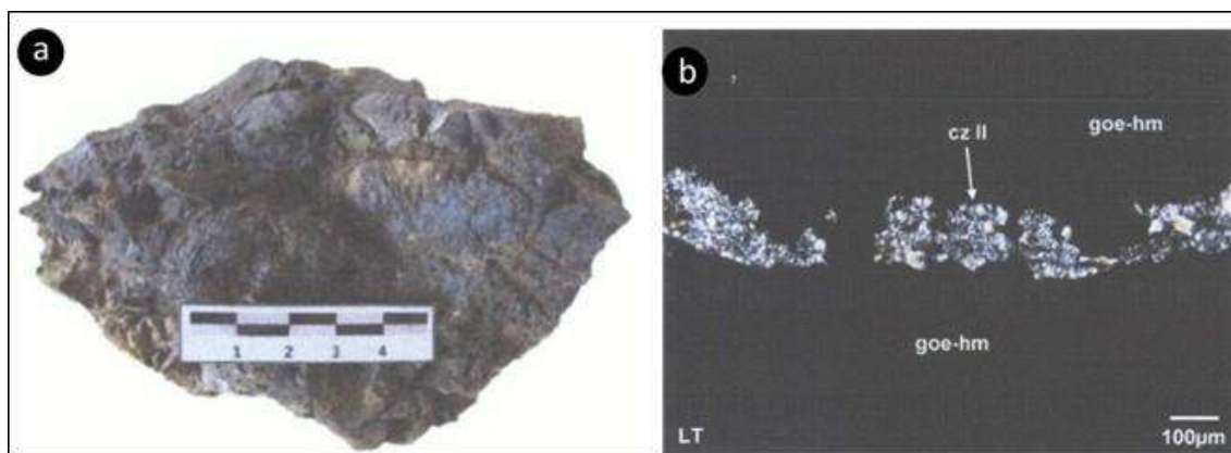
Figura 6.47. Análisis mineralógico por microscopía óptica de la muestra ROxP-15 a) vista macroscópica y b) vista microscópica de matriz, venas y fracturas rellenas por agregados de goethita y hematita (goe-hm) asociados con agregados de pequeños cristales de cuarzo II (cz II) en sus a intersticios.
