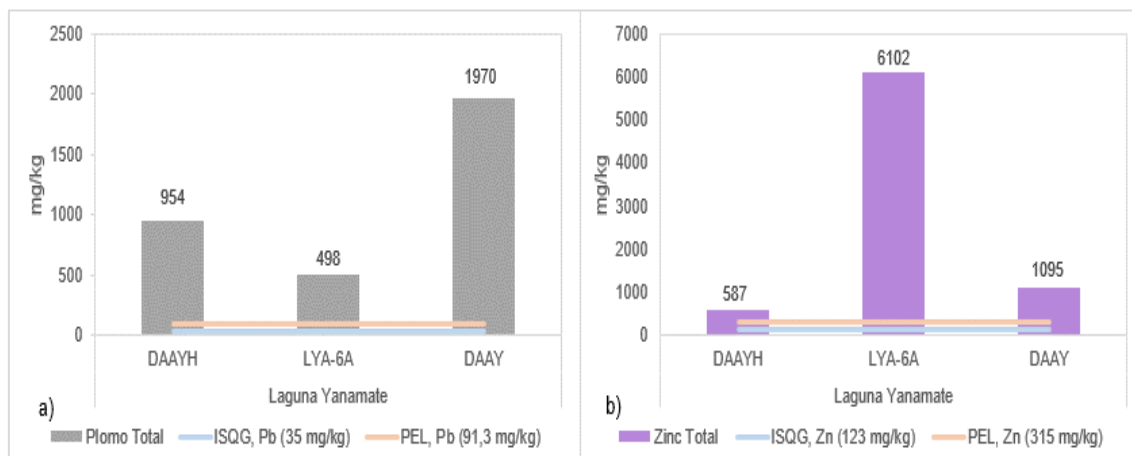
Figura 6.59. Resultados de metales en sedimento, comparados referencialmente con los valores ISQG y PEL de la CEQG-SQG en a) plomo y b) zinc
