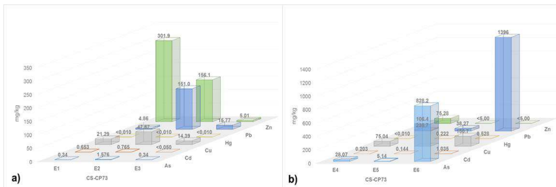
Figura 6.108. Extracción secuencial de metales por la metodología de Tessier, a) extracción 1, 2 y 3; y b) extracción 4, 5 y 6 en la muestra CS-CP73
