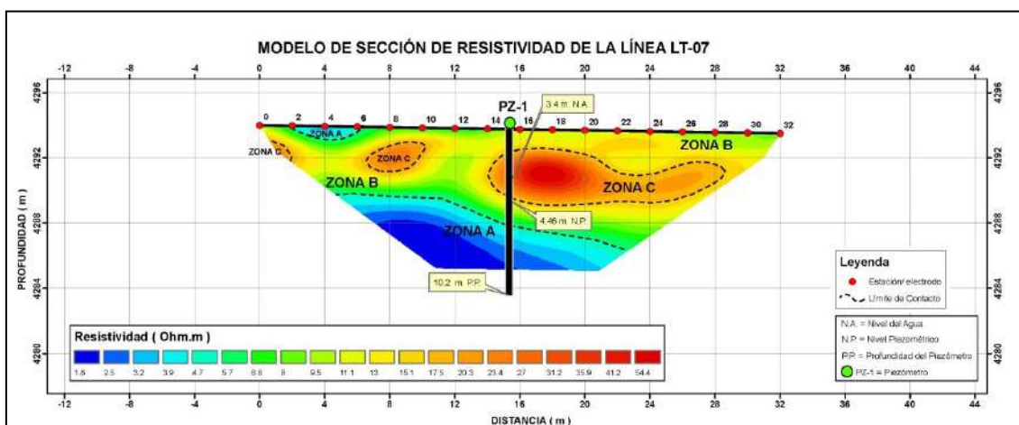
Figura 7.11. Esquema de ubicación de la línea LT-07 y modelo de sección de resistividades mostrando zonas saturadas
