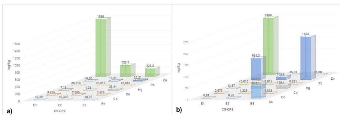
Figura 6.105. Extracción secuencial de metales por la metodología de Tessier, a) extracción 1, 2 y 3; y b) extracción 4, 5 y 6 en la muestra CS-CP6
