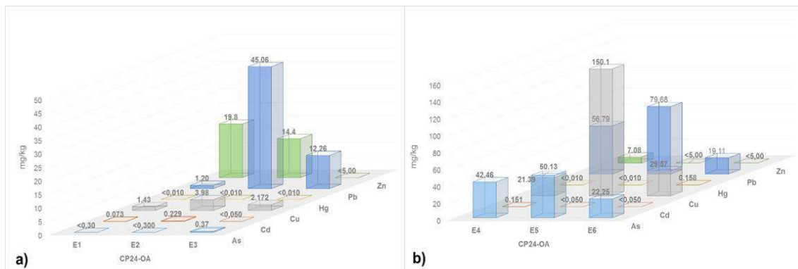
Figura 6.92. Extracción secuencial de metales por la metodología de Tessier, a) extracción 1, 2 y 3; y b) extracción 4, 5 y 6 en la muestra CP24-OA
