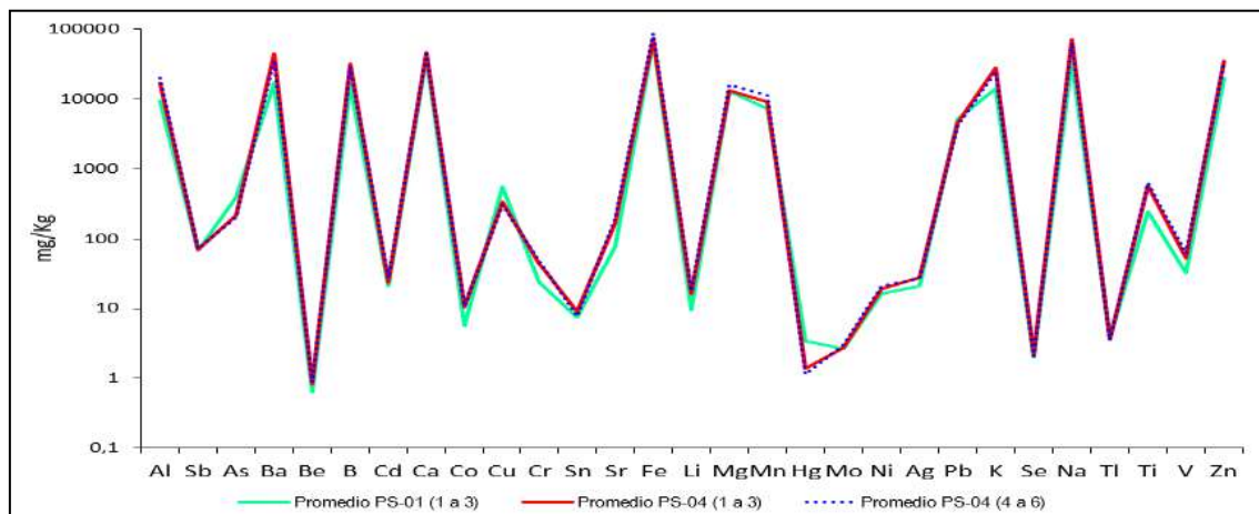
Figura 7.20. Concentración promedio de metales en material particulado sedimentable frente a la planta Paragsha, parque infantil Paragsha y estadio Paragsha,
