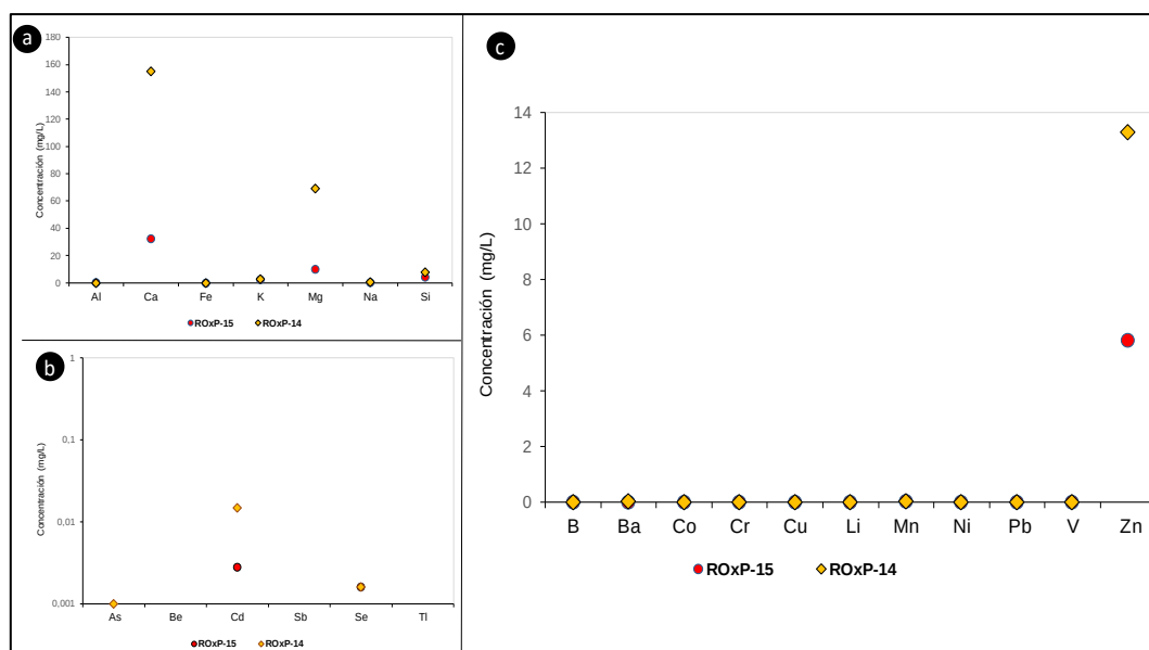
Figura 6.40. Shake Flask metales en las muestras ROxP-15 y ROxP-14
