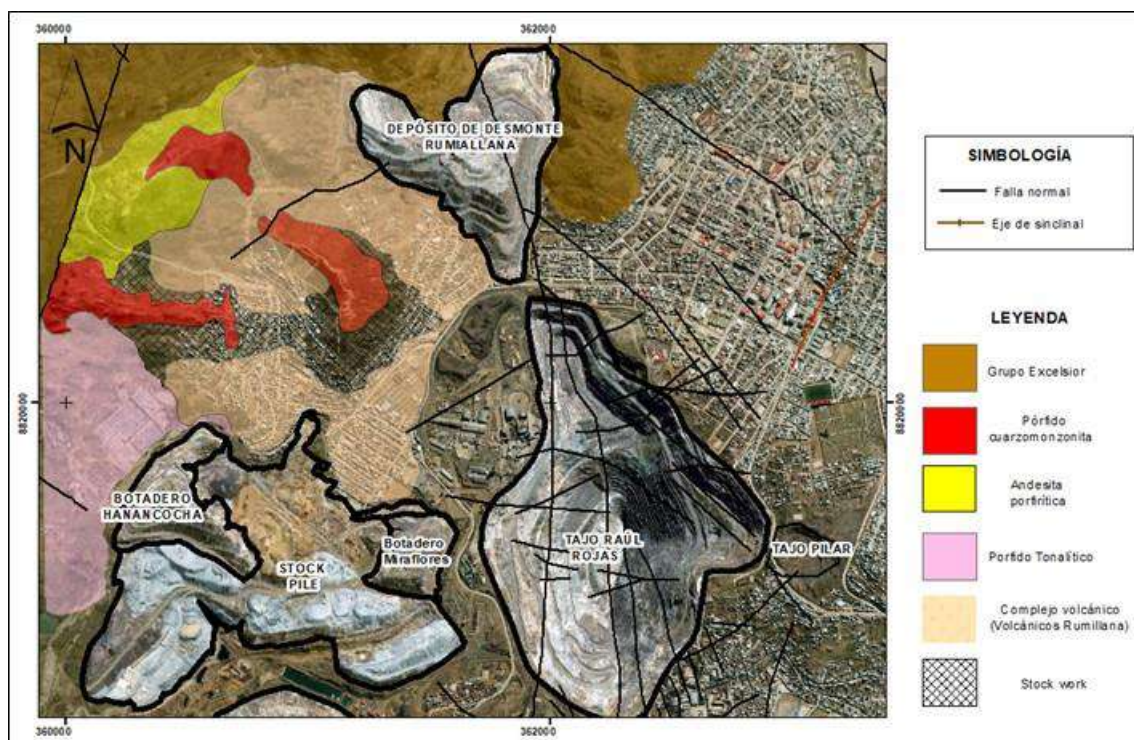
Figura 6.23. Plano geológico local de UF Cerro de Pasco
