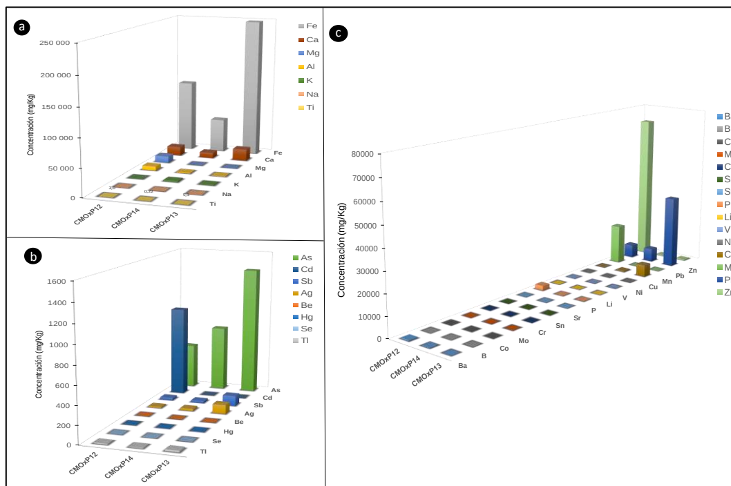
Figura 6.3. Metales totales de material del tajío Raúl Rojas en a) elemento mayores b) elemento menores y c) elementos traza
