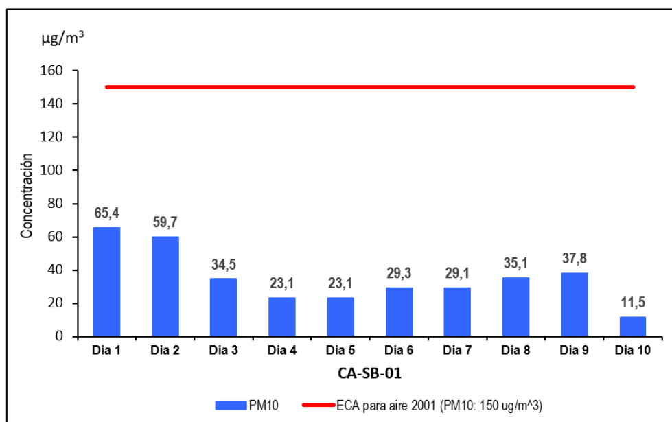
Figura 6.85. Concentración diaria de PM 10 en el punto de monitoreo CA-SB-01 comparada con los ECA para aire 2001
