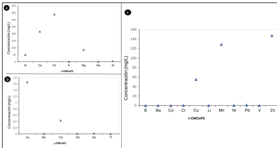
Figura 6.7. Shake Flask metales en el depósito de desmonte Miraflores en relación a los a) elementos mayores y b) elementos menores y c) elementos traza
