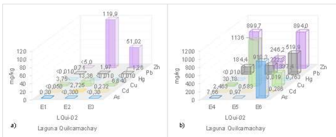
Figura 6.60. Resultados de metales (arsénico, cadmio, cobre, mercurio, plomo y zinc) por extracción Tessier del punto LQui-02 en a) extracciones E1, E2 y E3; y b) extracciones E4, E5 y E6 – agosto 2020
