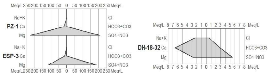
Figura 7.12. Graficas de Stiff de los piezómetros PZ-1 y DH-18-02, y punto de agua residual ESP-3
