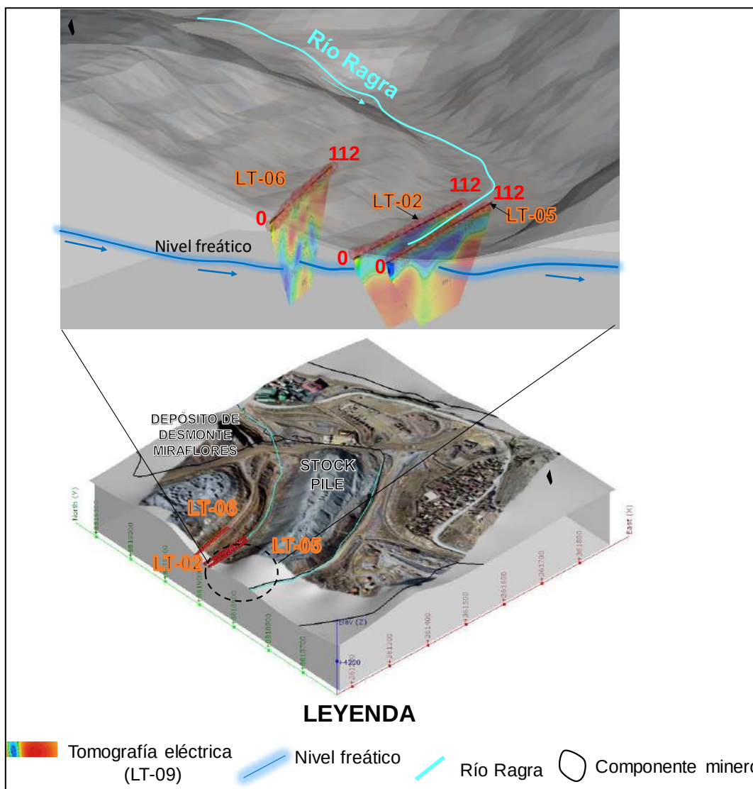
Figura 7.10. Secuencia de líneas de tomografía de resistividad eléctrica, mostrando zonas saturadas en LT-02 y LT-05
