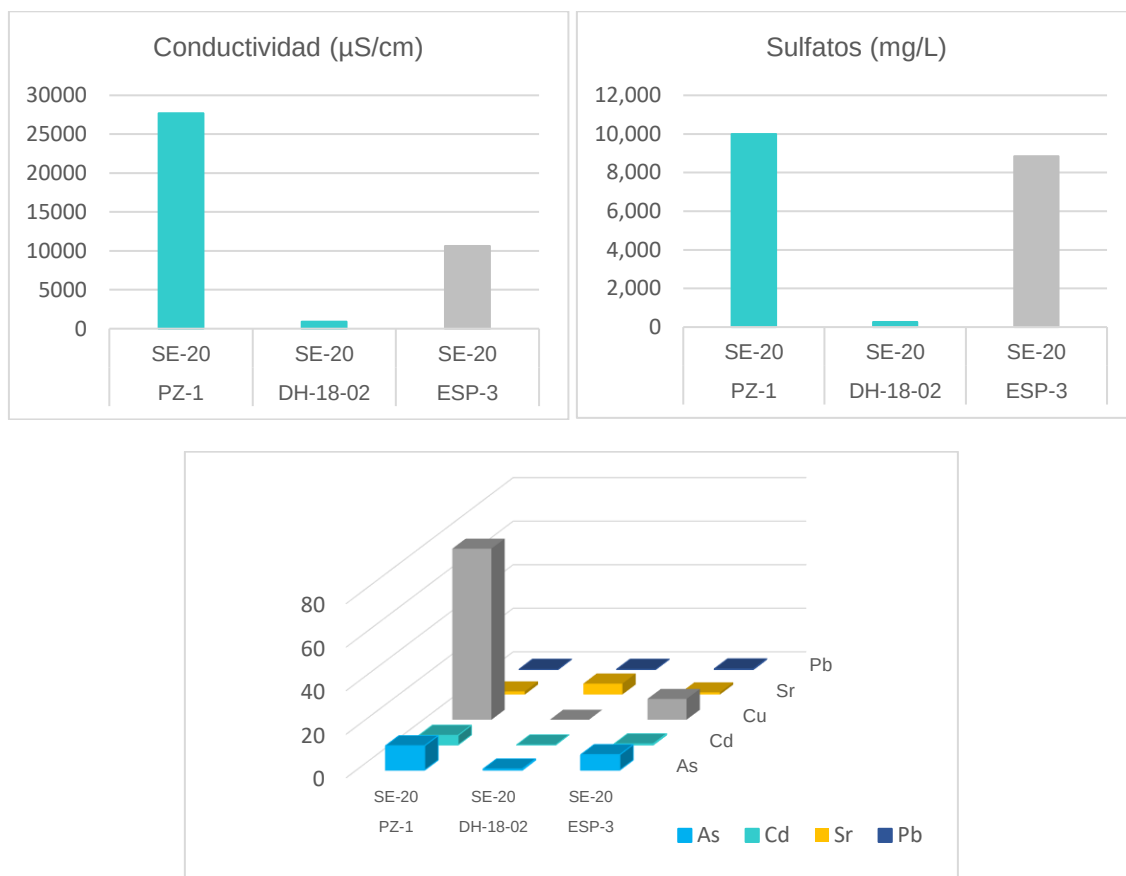
Figura 7.13. Resultados de a) conductividad, b) sulfatos y c) metales en agua subterránea (PZ-1 y DH-18-02) y agua residual (ESP-3)
