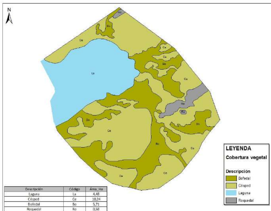
Figura 6.126. Cobertura vegetal de área sobrevolada
