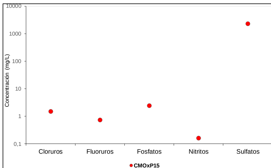
Figura 6.8. Shake Flask aniones en el material aledaño al tajo Raúl Rojas
