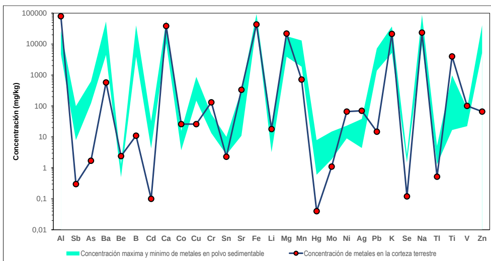
Figura 6.89. Concentración máxima y mínima de metales en polvo sedimentable comparados con la concentración promedio de metales en la corteza terrestre
