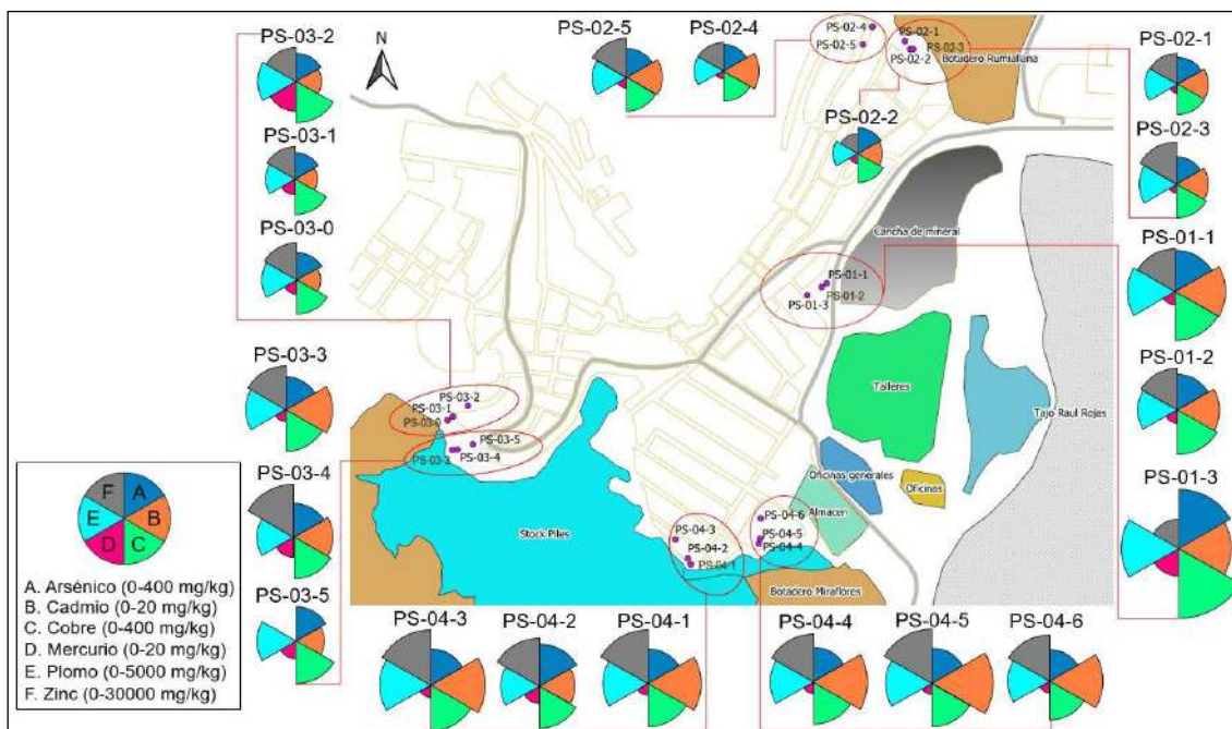
Figura 7.16. Distribución de las concentraciones de metales en material particulado sedimentable para arsénico, zinc, plomo, cadmio, cobre y mercurio, evaluados en el ámbito de la UF Cerro de Pasco
