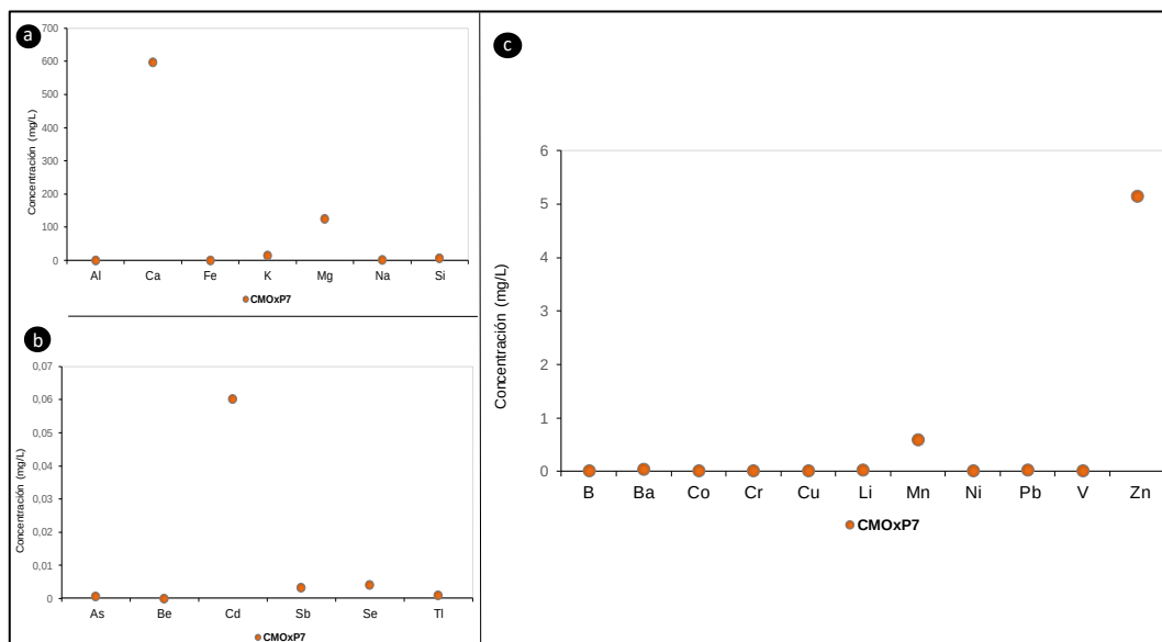
Figura 6.13. Shake Flask metales en el depósito de desmonte Rumiallana en relación a los a) elementos mayores y b) elementos menores y c) elementos traza
