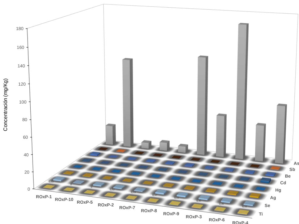
Figura 6.34. Metales totales en la UF Cerro de Pasco para los elementos menores
