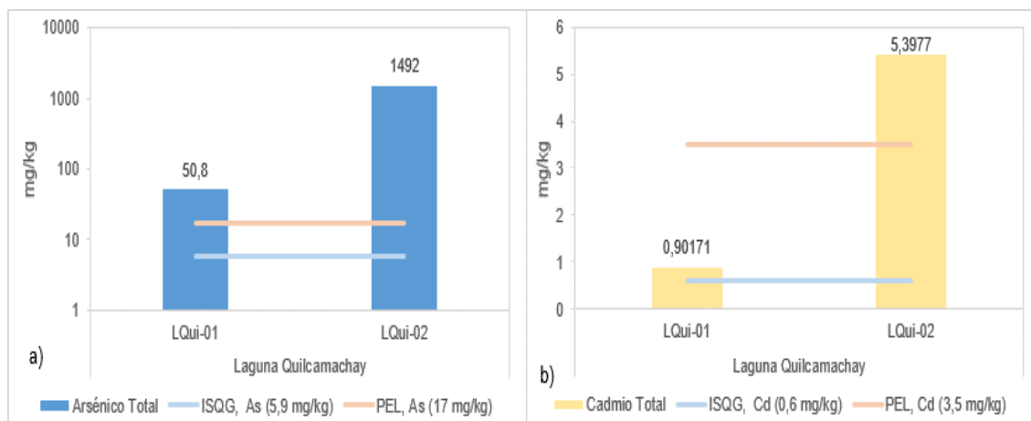
Figura 6.54. Resultados de metales en sedimento, comparados referencialmente con los valores ISQG y PEL de la CEQG-SQG en a) arsénico y b) cadmio
