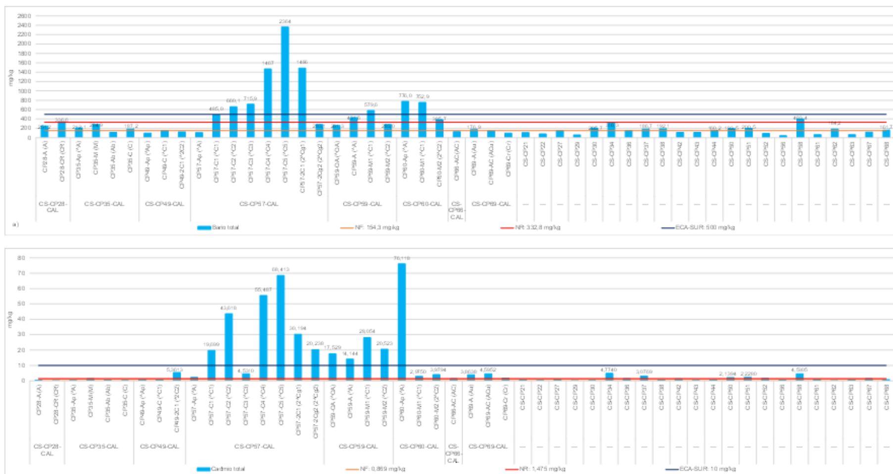
Figura 6.101. Concentraciones de a) bario total y b) cadmio total comparadas con ECA para suelos de uso residencial (ECA-SUR), nivel de fondo (NF) y nivel de referencia (NR)
