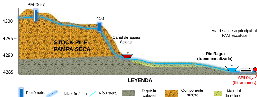
Figura 7.14. Esquema conceptual del comportamiento hidrodinámico del stock pile Pampa Seca y canal de aguas ácidas
