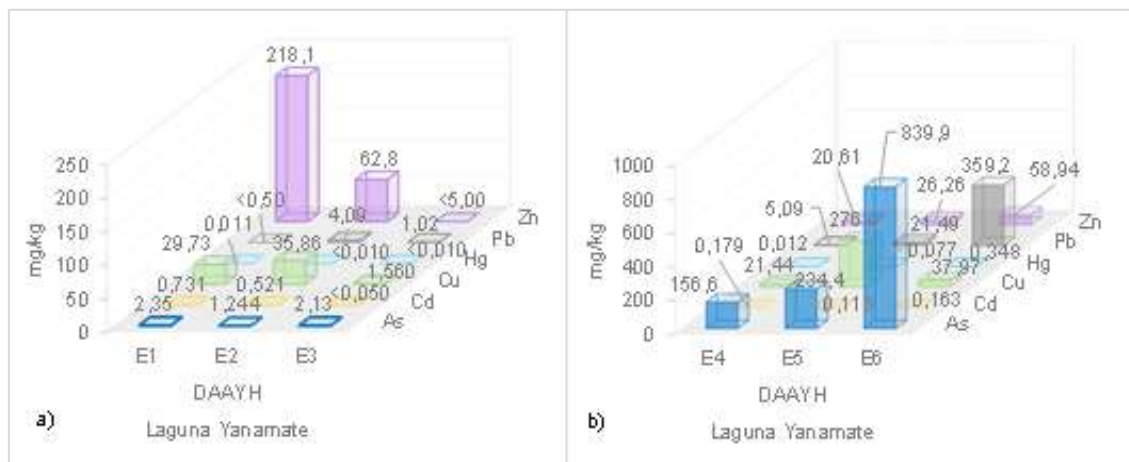
Figura 6.61. Resultados de metales (arsénico, cadmio, cobre, mercurio, plomo y zinc) por extracción Tessier del punto DAAYH en a) extracciones E1, E2 y E3; y b) extracciones E4, E5 y E6 – agosto 2020
