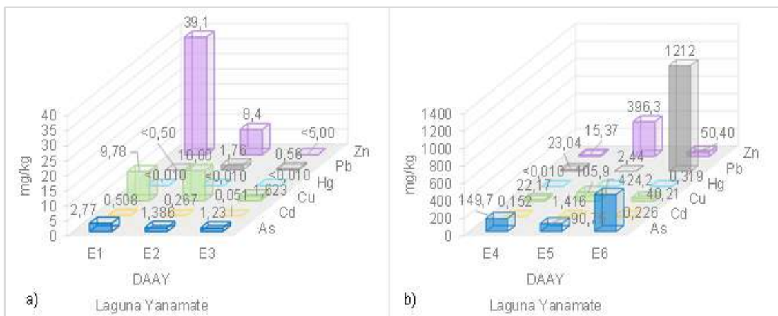
Figura 6.63. Resultados de metales (arsénico, cadmio, cobre, mercurio, plomo y zinc) por extracción Tessier del punto DAA en a) extracciones E1, E2 y E3; y b) extracciones E4, E5 y E6 – agosto 2020
