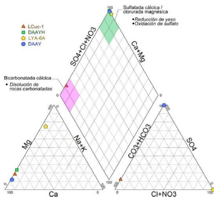
Figura 7.39. Diagrama de Piper para del depósito de aguas ácidas Yanamate (DAAYH, LYA-6A y DAAY) y laguna Chuchis (LCuc-1)
