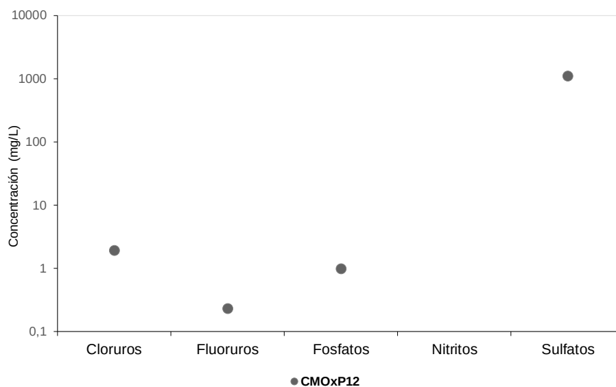
Figura 6.10. Shake Flask aniones en el Tajo Raúl Rojas
