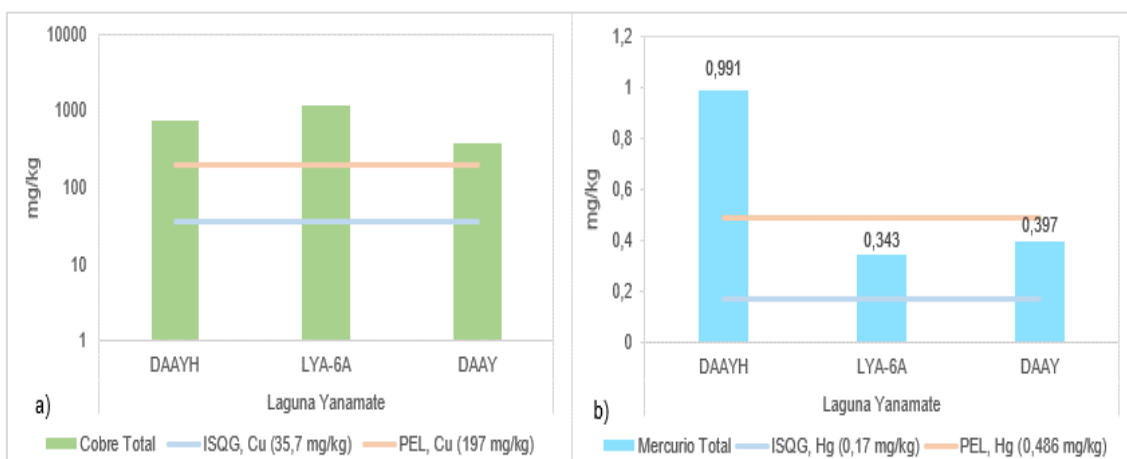
Figura 6.58. Resultados de metales en sedimento, comparados referencialmente con los valores ISQG y PEL de la CEQG-SQG en a) cobre y b) mercurio
