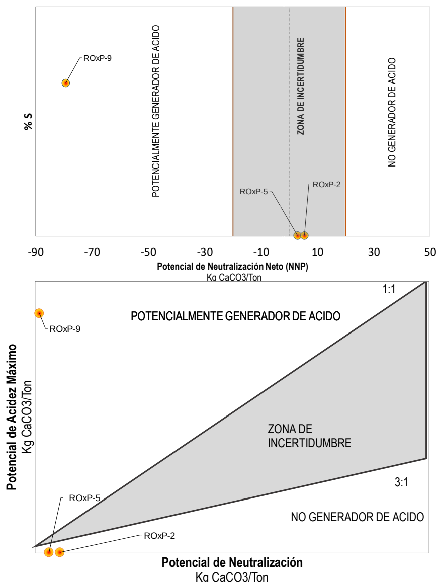
Figura 6.42. ABA en las muestras ROxP-5, ROxP-2 y ROxP-9, según el primer y segundo criterio de evaluación
