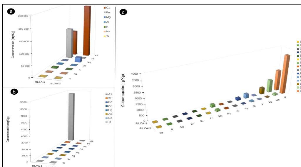
Figura 6.32. Metales totales en el ámbito de laguna Yanamate a) elementos mayores b) elementos menores c) elementos traza
