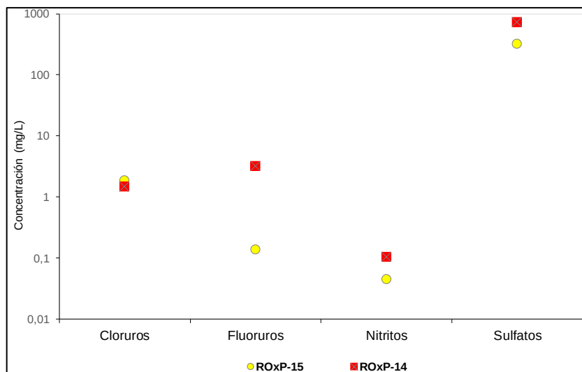
Figura 6.39. Shake Flask aniones en ROxP-15 y ROxP14
