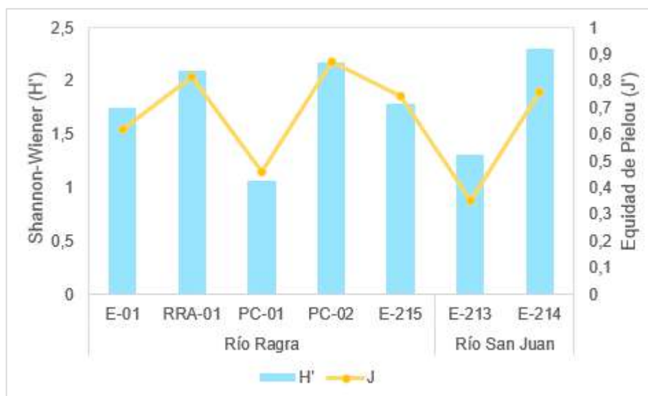
Figura 6.68. Índice de Shannon –Wiener de microalgas – agosto 2020
