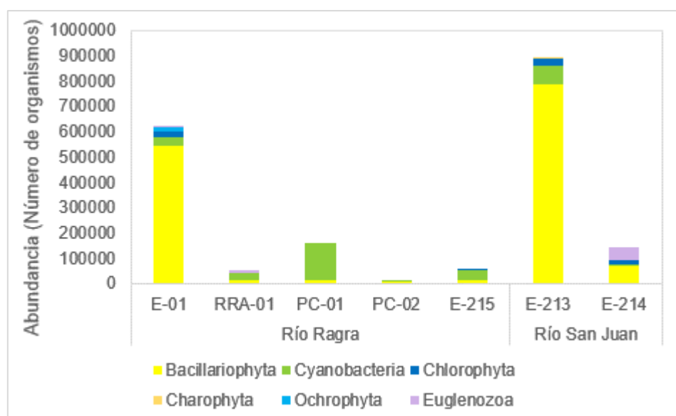
Figura 6.66. Abundancia de microalgas – agosto 2020
