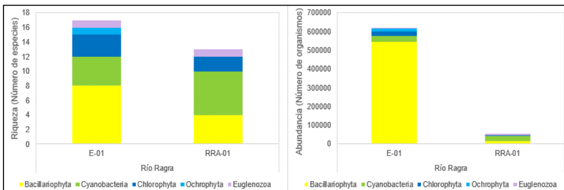
Figura 7.49. a) Composición y riqueza de perifiton (microalgas) y b) Abundancia de perifiton (microalgas) – agosto 2020
