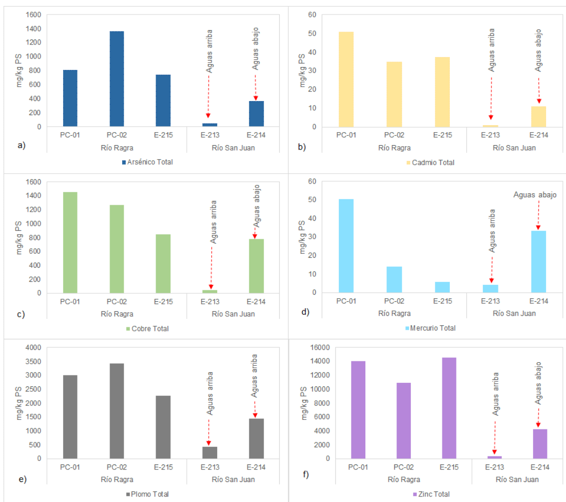
Figura 7.47. Concentraciones de metales en sedimento en el río Ragra y San Juan en a) arsénico, b) cadmio, c) cobre, d) mercurio, e) plomo y f) zinc
