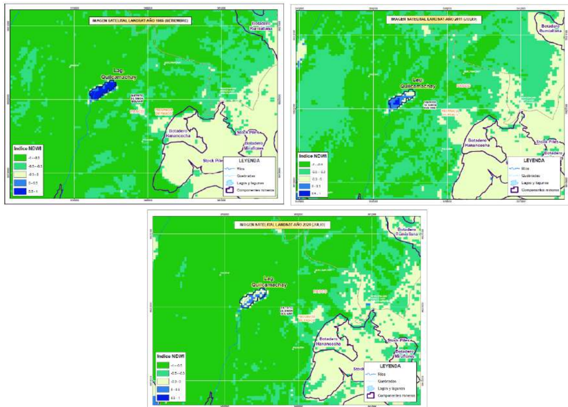
Figura 7.8 Análisis del índice NDWI en la laguna Quilcamachay para los años 1985 (setiembre), 2011 (julio) y 2020 (julio)
