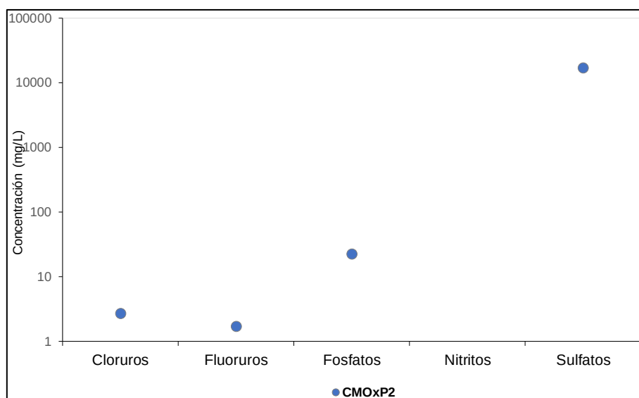
Figura 6.6. Shake Flask aniones en el depósito de desmonte Miraflores
