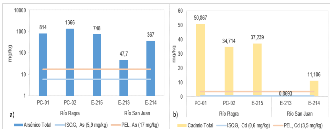
Figura 6.48. Resultados de metales en sedimento, comparados referencialmente con los valores ISQG y PEL de la CEQG-SQG en a) arsénico y b) cadmio – agosto 2020
