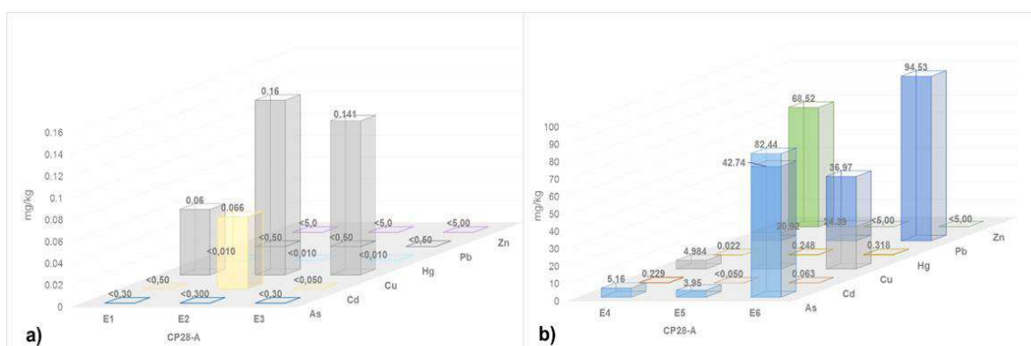
Figura 6.110. Extracción secuencial de metales por la metodología de Tessier, a) extracción 1, 2 y 3; y b) extracción 4, 5 y 6 en la muestra CP28-A
