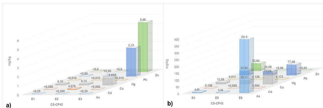
Figura 6.112. Extracción secuencial de metales por la metodología de Tessier, a) extracción 1, 2 y 3; y b) extracción 4, 5 y 6 en la muestra CS-CP43
