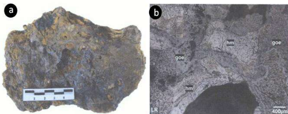
Figura 6.46. Análisis mineralógico por microscopía óptica de la muestra ROxP-14 a) vista macroscópica y b) vista microscópica de agregados irregulares a masivos de goethita (goe) con hematita (hm) que han invadido algunos sectores de la roca.
