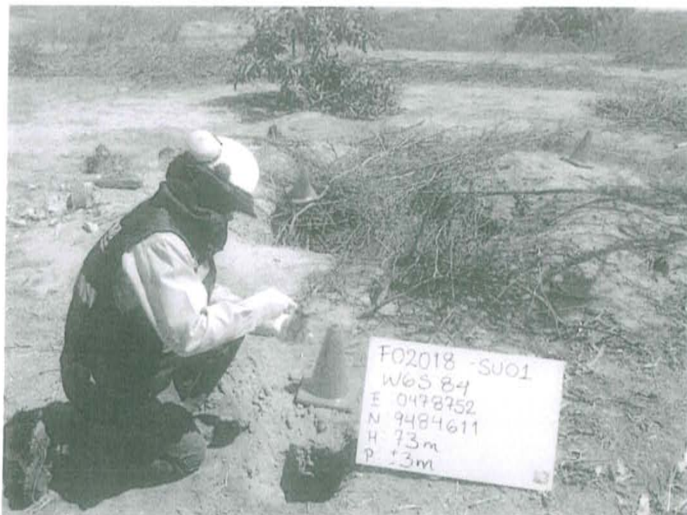
Fotografía N° 1. Toma de muestra de suelo en el punto F02018-SU01, ubicado a 2,5 m aproximadamente del Pozo T3848.
