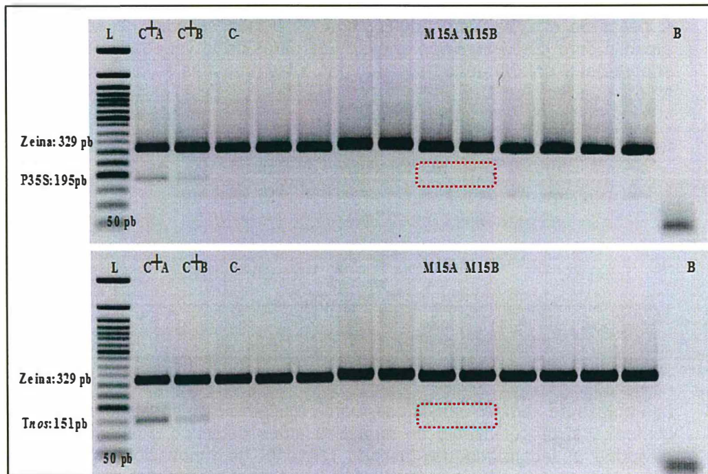
Figura N° 1 Perfil electroforético para la detección de la secuencias P35S y Tnos en la muestra ANC160420 EC01
