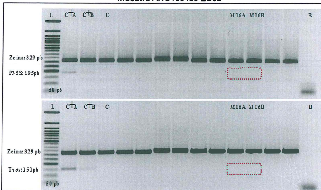
Figura N° 2 Perfil electroforético para la detección de la secuencias P35S y Tnos en la muestra ANC160420 EC02
