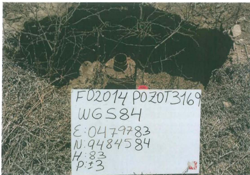
Fotografía N° 1. Pozo T3169, con casing a una altura de 0,25 m desde el nivel del suelo del hoyo, de 9,84 plg de diámetro externo y 3,15 plg de diámetro interno, con brida empernada y sin accesorios que aseguren su hermetismo
