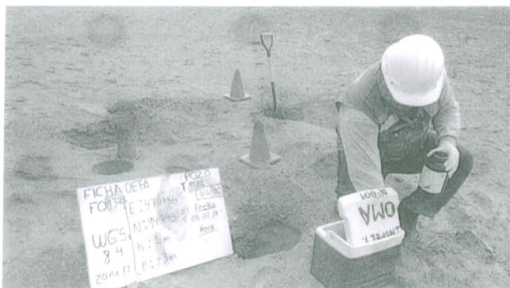
Fotografía N° 2. Toma de muestra de suelo en el punto F01371-SU02, ubicado a 1,3 m aproximadamente del Pozo T1188.
