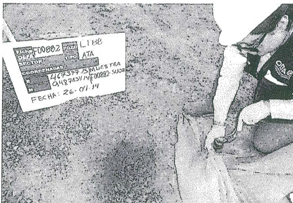
Fotografía N° 2. Toma de muestra de suelo en el punto F00882-SU02, ubicado a 5,6 m de distancia del Casing, Pozo T_888.
