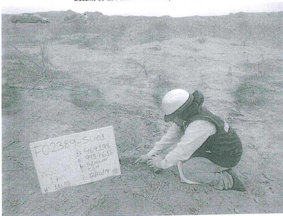
Fotografía N° 1. Toma de muestra de suelo en el punto F02389-SU01, ubicado a 20 m de distancia, al oeste de la posible ubicación del Pozo T_775.
