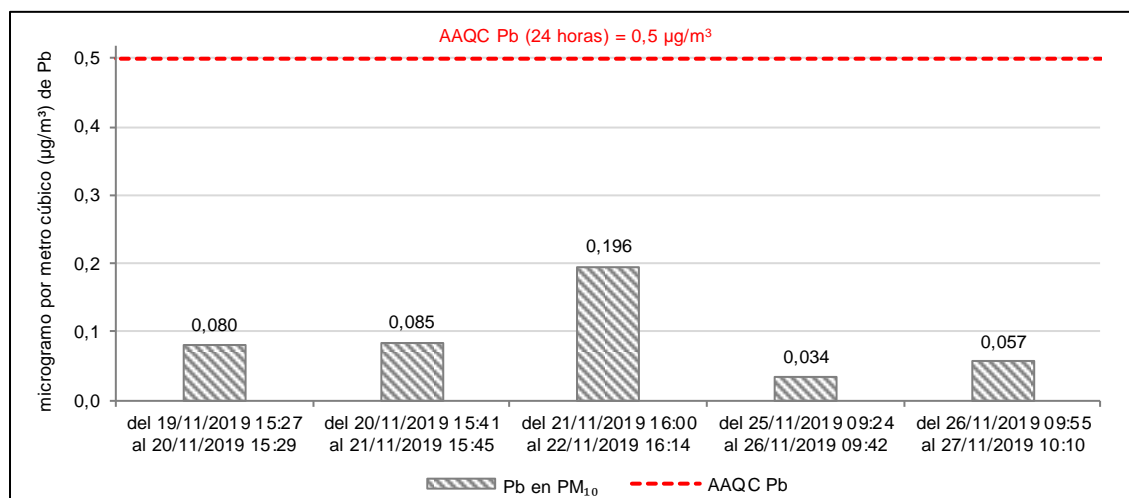
Figura 5.6. Concentraciones de plomo en material particulado con diámetro menor a 10 micras (Pb en PM 10 ) a 10°C y de 24 horas en noviembre 2019, de la estación de vigilancia ambiental de la calidad del aire CA-SB-01, comparadas de manera referencial con la normativa canadiense AAQC-2012.
