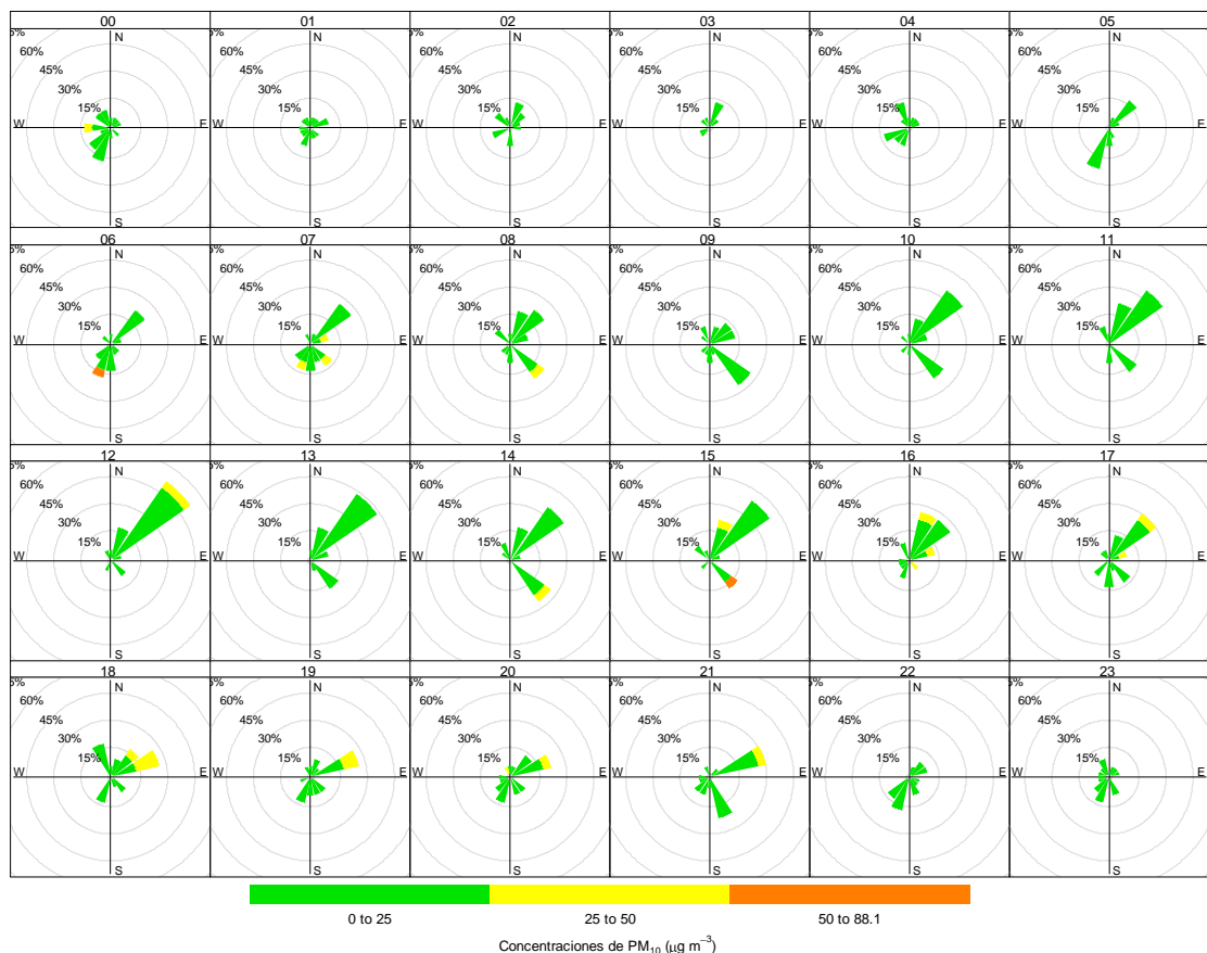
Figura 5.5. Rosas de concentración por horas de PM 10 en la estación de vigilancia CA-SB-01, desde las 00:00 horas hasta las 23:00 horas, en noviembre de 2019 Nota: Las paletas indican la dirección de donde provienen las concentraciones de PM 10
