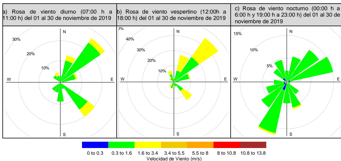
Figura 5.1. Representación gráfica de las rosas de vientos en la estación de vigilancia ambiental CA-SB-01, en noviembre de 2019 a) en horario diurno, b) en horario vespertino, c) en horario nocturno. Nota: Las paletas indican la dirección desde donde provienen los vientos
