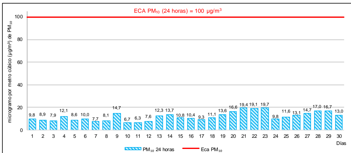
Figura 5.3. Concentraciones de 24 horas de PM 10 en la estación de vigilancia ambiental CA-SB-01, noviembre de 2019.
