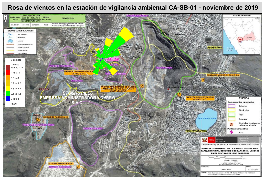
Figura 5.2. Ubicación de la estación de vigilancia ambiental CA-SB-01 y rosa de vientos en noviembre de 2019 Referencia: Imágenes satelitales extraídas de Google Earth.
