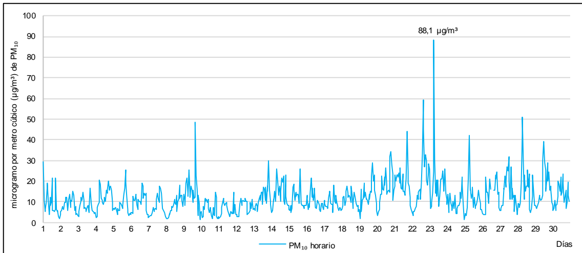
Figura 5.4. Concentraciones horarias de PM 10 en la estación de vigilancia ambiental CA-SB-01 en noviembre de 2019.
